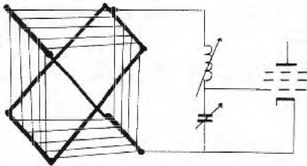
RAAMANTENNE
