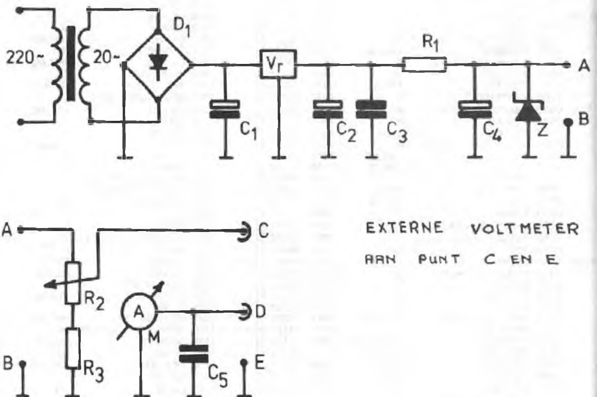
fig. 2 Voeding met resonantie-detector
