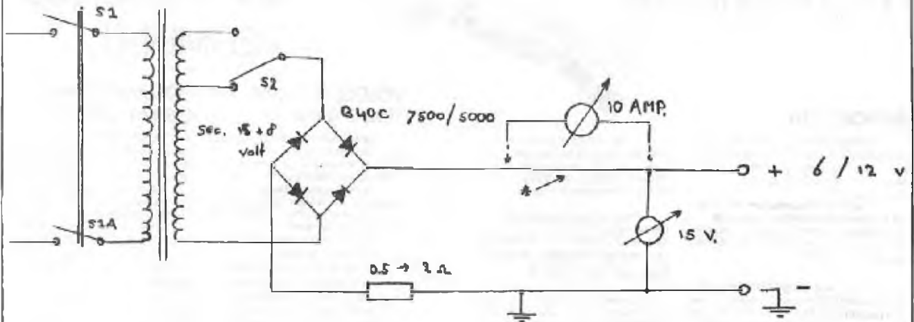
EENVOUDIGE LAAGSPANNINGSVOEDING
