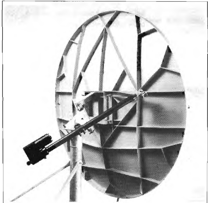
De motor-arm aan de achterzijde van de schotel 'stuurt' de schotel, zodat deze op diverse satellieten gericht kan worden.
