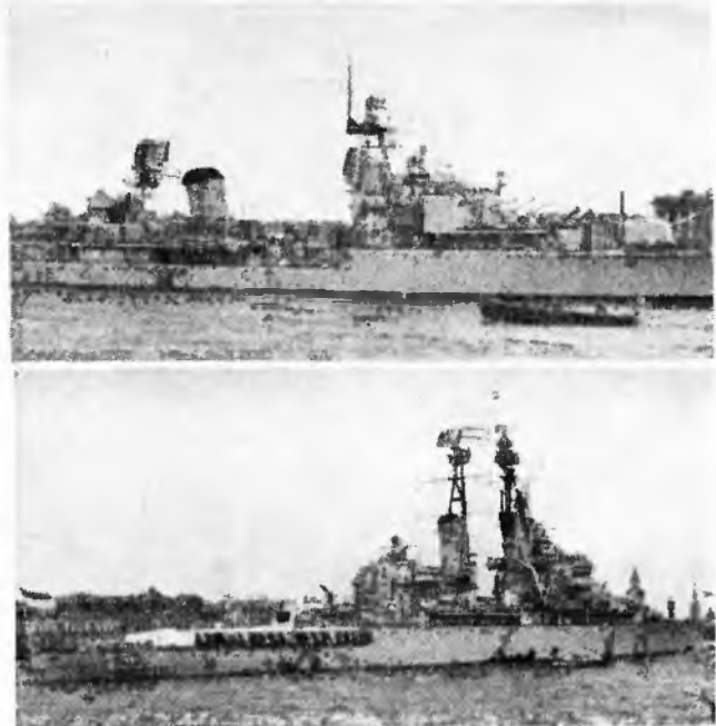
Bild 9–11: Auf den Schiffen sind Radar- antennen zu erkennen. Holländischer Zer- störer (Bild oben) mit Antennen in Bild- mitte und links. Holländischer Kreuzer (Bild Mitte) mit mehreren Antennen über den Schornsteinen. Radarantennen eines holländischen Kreuzers (Bild links).
