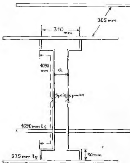
Bild 3: Zweiebenen-Vierelement-Antenne für das 2-m-Band, Abstand D (Rohrmitte zu Rohrmitte): für 240-Ohm-Kabel = 80 mm, für 70-Ohm-Kabel = 25 mm, Strahlerlänge = 975 mm, Reflektorlänge = 1090 mm, Abstand beider = 305 mm.
