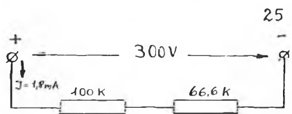
Bild 23–25: Zur Berechnung der Spannungsteilverhältnisse.
