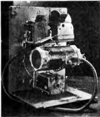
Bild 6: Antennenanpaßgerät, die Spule L ist mehrfach angezapft. Wirksam sind nur die acht Windungen, die unter der Koppelspule liegen.
