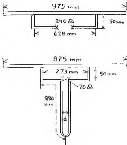
Bild 6: Anpassung bei Verwendung von nur einer Ebene der Antenne nach Bild 4 als Einebenen-9-Element-Antenne. Abstand D (Rohrmitze zu Rohrmitze) = 20 mm.
