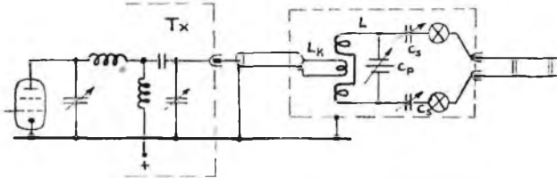
Bild 5: Antennenanpaßgerät, anschließbar an Collinstankkreis mit 70-Ohm-Ausgang. Link-Leitung aus Koaxkabel, die Länge ist beliebig. Anpaßgerät unmittelbar an der Herausführung der Speiseleitung aus dem shack anordnen. L = 8 Wdgn. 2 mm Cu, 60 mm \varnothing , L_k = 2 Wdgn. 2,5 mm Cu im Abstand von etwa 3 mm auf Abstandsklötzchen aus Plexiglas darüber gewickelt. C_s je 500 pF (hier Drehkos aus dem alten VE 301), C_p etwa 100 pF, wichtig ist eine kleine Anfangskapazität (verwendet wurde ein Splitdrehko), Soffittenlampen statt HF-Instrumente zur Anzeige.
