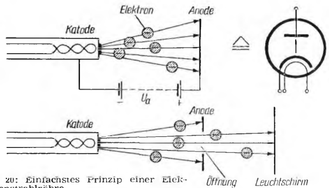
Bild 20: Einfachstes Prinzip einer Elektronenstrahlröhre.
