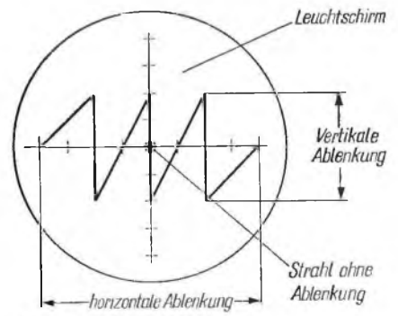
Bild 22: Strahlablenkung.
