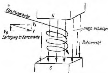
Bild 17: Ablenkung des Elektrons im magnetischen Feld ( V steht nicht \perp zu B ).
