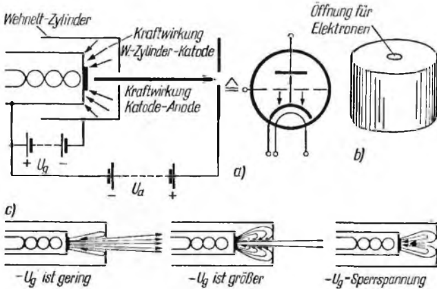
Bild 21: Prinzip, Aufbau und Wirkungsweise des Wehneltzylinders.
