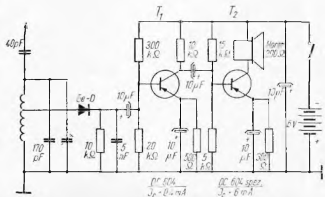
Bild 2: Schaltbild des Transistorempfängers.
