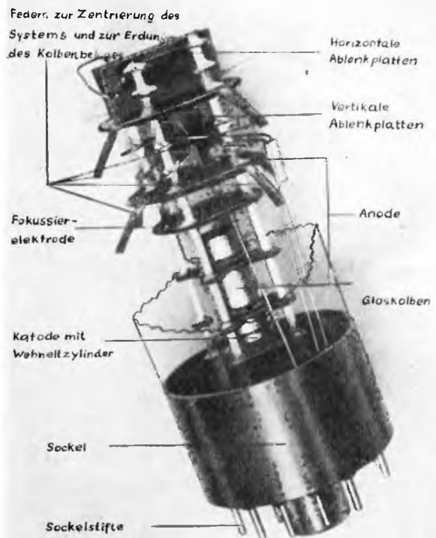
Bild 18: Innerer Aufbau einer Elektronenstrahlröhre mit doppelter elektrostatischer Ablenkung.
