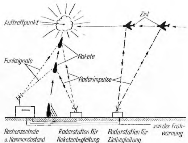
Bild 7: Prinzipdarstellung der Radarsteuerung von Abwehrraketen nach dem Kommandoverfahren.
