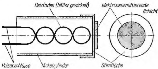
Bild 19: Aufbau der Kathode.
