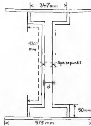
Bild 5: Strahler mit Anpassglied für Antenne nach Bild 4. Alle Rohr-Ø 12 mm, Abstand D (Rohrmitte zu Rohrmitte) 35 mm für 70-Ohm-Kabel (rechts).
