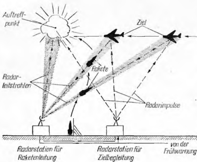
Bild 8: Prinzipdarstellung der Raketensteuerung von Abwehr- raketen nach dem Leitstrahlverfahren.
