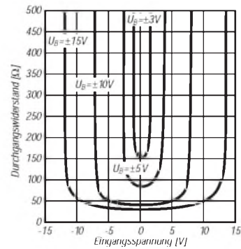
Bild 5: Abhängigkeit des On-Widerstands von der Eingangsspannung bei dualer Versorgung
