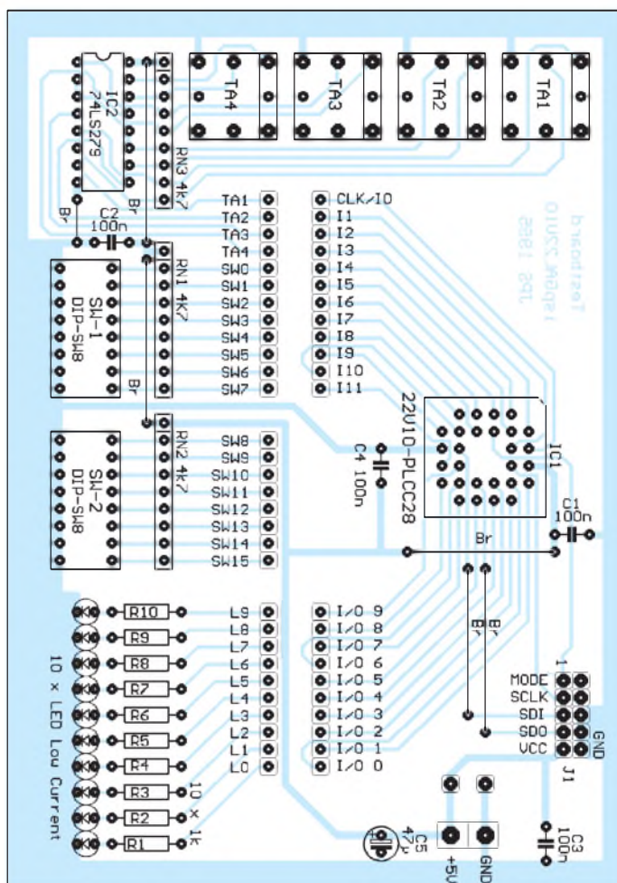
Bild 7 : Bestückungsplan für das Test- und Entwicklungsboard
