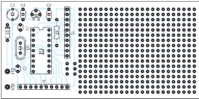
Bild 7: Bestückungsplan
