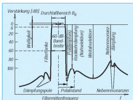
Bild 1: Typische ZF-Filter-Durchlaßkurve
