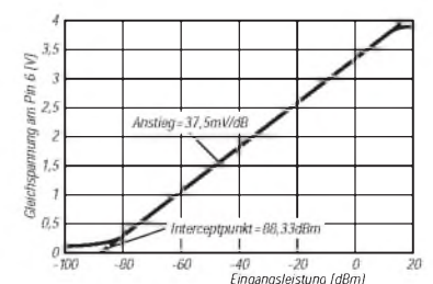
Bild 2: Typischer Verlauf der Übertragungsfunktion
