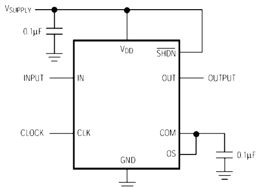
Bild 8: Minimale Außenbeschaltung
