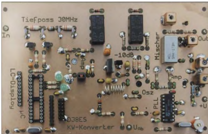
Bild 1: Ansicht der fertig bestückten Musterplatine
