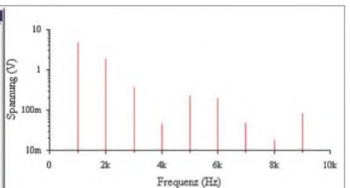
Bild 2: Asymmetrische Verzerrerrstufe mit Dioden. Ausgangssignal und spektrale Zusammensetzung
