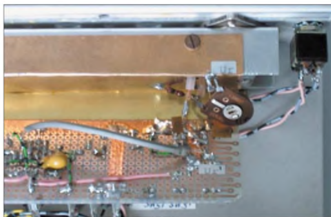
Bild 11: Zur Vermeidung von HF-Einkopplungen auf die schräg davor angebrachte Platine ist der Richtkoppler mit einem Kupferblech verschlossen. Fotos: DL7HG
