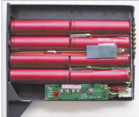
Bild 4: Akku geöffnet, unten erkennbar die Elektronik mit Ladezustandsanzeige
