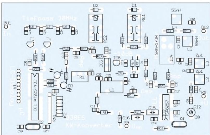
Bild 7: Bestückungsplan für den KW-Konverter
