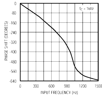
Bild 7: Phasengang in Abhängigkeit von der Eingangsfrequenz
