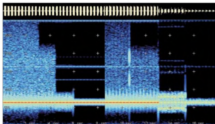
Die Wirkung der Bandbreitenumschaltung bei normalem (links) und zu hohem Eingangspegel (rechts; Anzeigepegel zur Vergleichbarkeit für Gram ausgangseitig wieder angeglichen!). Es entstehen Phantomsignale; das Nutzsignal „geht unter“.
