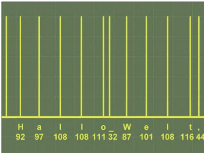
Bild 77: Das gesendete PIM-Signal
