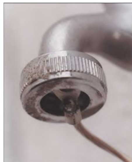
Bild 4: Ein schneller Weg zur Verbindung des Erdungskabels mit dem Wasserleitungsnetz, wenn es denn aus Metall ist ...
