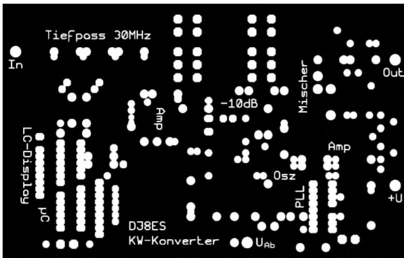
Bild 6: Bestückungsseite der 160 mm x 100 mm großen Platine des KW-Konverters, hier dargestellt im Maßstab 1:1,5
