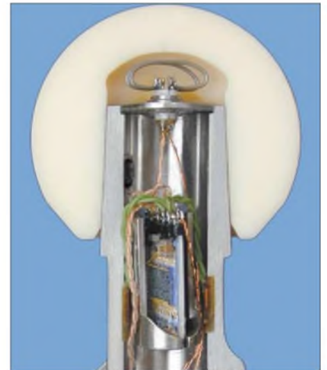
Bild 78: Hüftgelenkprothese mit PIM-Sender Quelle: Biomechanik-Labor, Freie Universität Berlin
