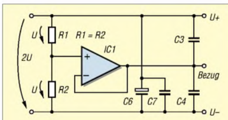
Bild 44: Spannungsfolger zur Aufbereitung einer bipolaren aus einer unipolaren Spannung
