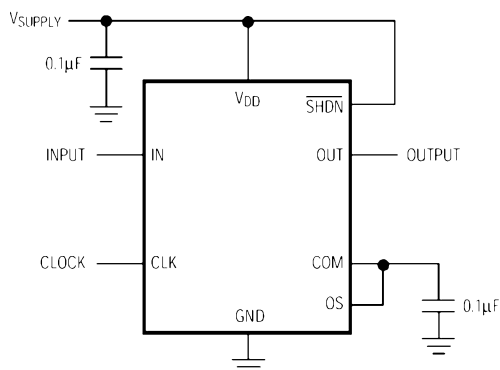
Bild 8: Minimale Außenbeschaltung
