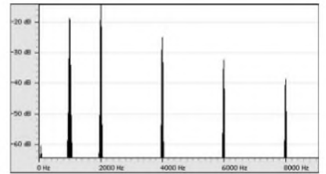
Bild 15: Klangspektrum bei asymmetrischer Verstärkung
