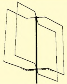
Bild 9: Diese Antenne nach HB9CV ist robust und kompakt. Der Reflektor-Direktor-Abstand darf bis 0,05 \lambda reduziert werden!
