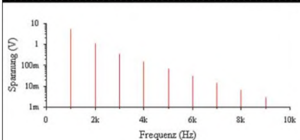
Bild 16: Harmonische Verzerrungen einer übersteuerten Transistorverstärkerstufe
