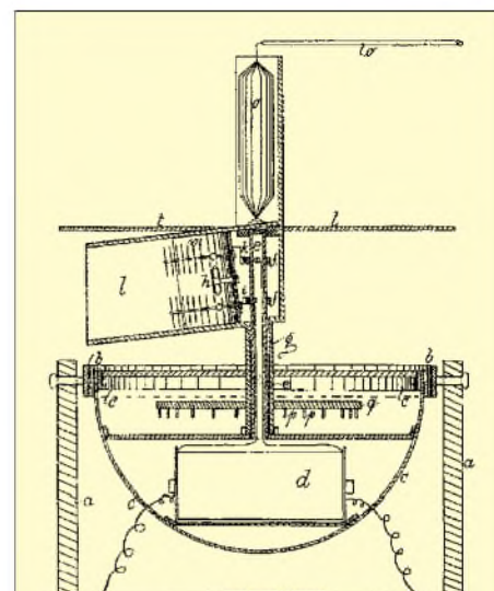
Bild 2: Die Hauptzeichnung von C. Hülsmeiers „Radar“-Patent. Unten eine kardanische Aufhängung abc. Darüber montiert ist der Kasten I mit der Sendeantenne und die Empfangsantenne o. Die Anordnung ist um den Zapfen e drehbar. aus Patent DE 165 546
