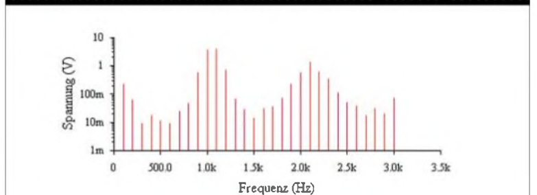
Bild 17: dto., jedoch mit zwei Sinussignalen unterschiedlicher Frequenz beaufschlagt
