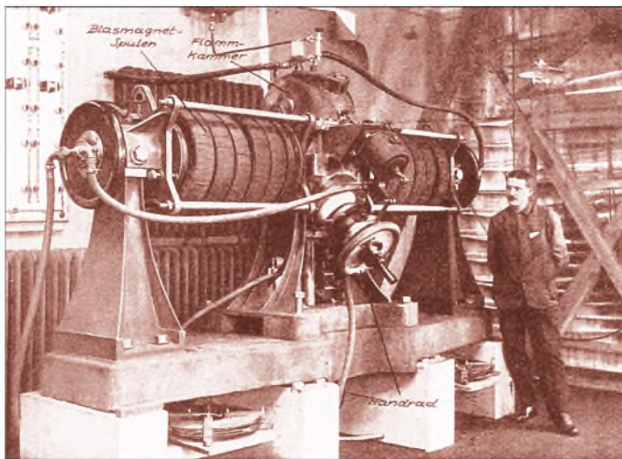
Bild 1: Gut zu erkennen ist das Handrad, mit dem der Kohlestab in der Flammkammer nachgeschoben wurde. Die Abmessungen dieses durch die Firma C. Lorenz hergestellten Poulsen-Senders sind beträchtlich.
