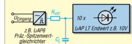
Bild 69: Schaltung zur Anzeige des Spitzenwertes der Eingangsspannung
