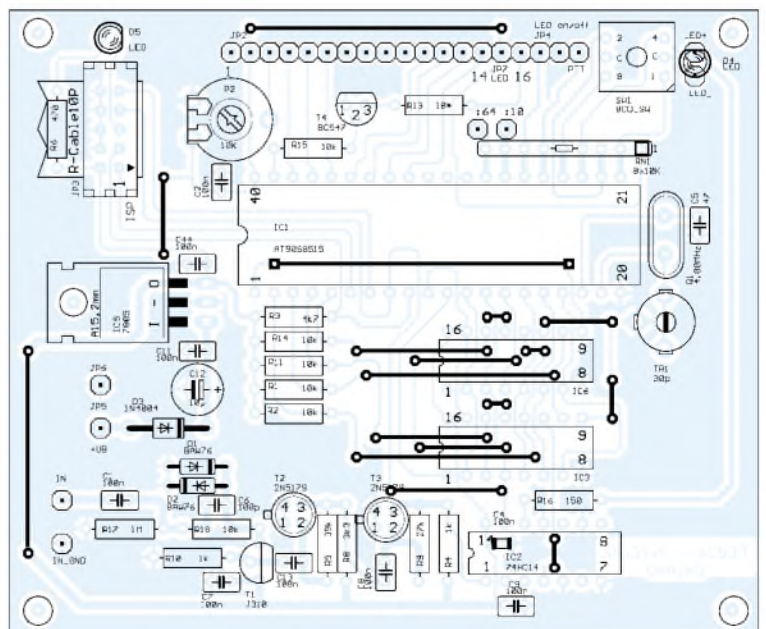
Bild 6: Auf der Bestückungsseite der Platine ist der BCD-Schalter noch eingezeichnet. Er sollte jedoch für eine bessere Bedienbarkeit von der Frontplatte aus erreichbar sein.
