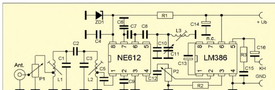
Bild 4: Das übersichtliche Schaltbild eines mit sPlan 5.0 gezeichneten Direktmischempfängers verdeutlicht den Vorteil gegenüber einer Handskizze.
