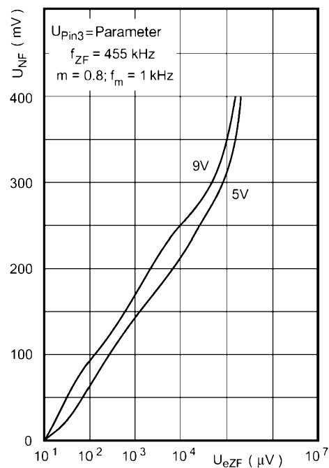
Bild 4: NF-Ausgangsspannung als Funktion der ZF-Eingangsspannung
