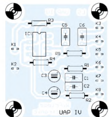
Bild 79: Bestückungsplan der einseitigen Platine UAP IV
