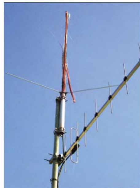
Die X7000 (5 m) des QTC-Autors nach dem Blitzschlag (nur noch knapp 1 m lang). Foto: DL9HQB
