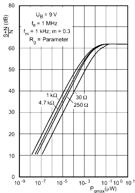
Bild 3: Signal-Rausch-Abstand als Funktion der Generatorleistung am Eingang
