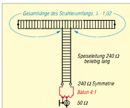
Bild 2: Der Halbwellen-Schleifendipol aus Flachbandleitung; für TV- und BC-Empfänger mit symmetrischem Eingang entfällt der Balun.
