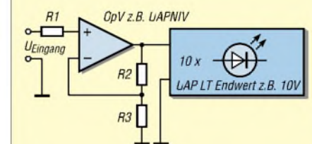
Bild 67: Messspannung im mV-Bereich
