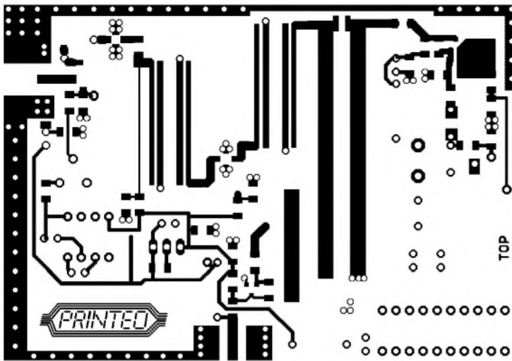
Bild 6: Oberseite der zweiseitigen Platine; die größte Fläche nehmen die aus der Kupferbeschichtung herausgeätzten Streifenleitungen ein.
