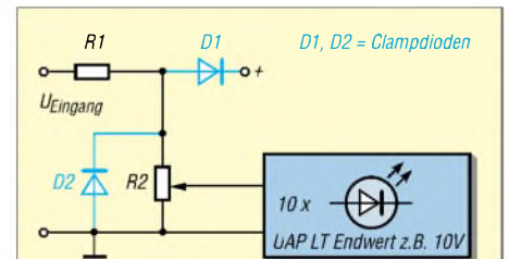
Bild 66: Schaltung für Messspannungen, die größer als 10 V sind
