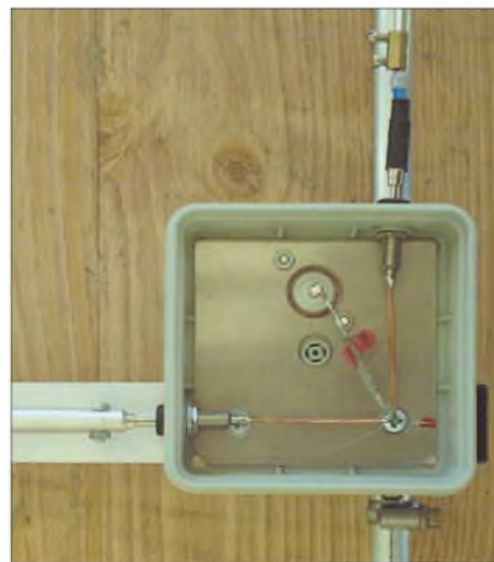
Bild 4: Innenansicht der Anschlussdose mit PL- und Bananenbuchsen
