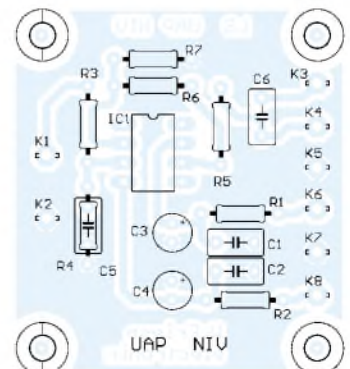
Bild 81: Bestückungsplan der einseitigen Platine UAP IV
