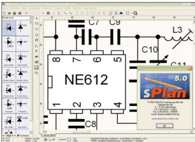
Bild 1: Die übersichtliche Arbeitsoberfläche ermöglicht eine intuitive Programmbedienung. Die Firmeninformation ist hier nur einblendend.
