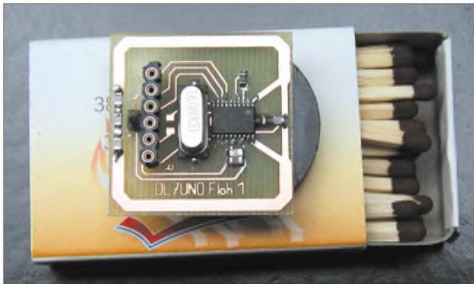
Bild 83: Der Flohsender
