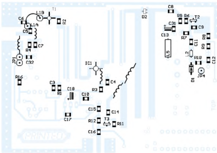
Bild 7: Bestückung auf der Platinoberseite mit dem Analogteil; die verwendeten SMD-Bauteile lassen sich auf Grund des vorhandenen Platzes gut auflöten.
