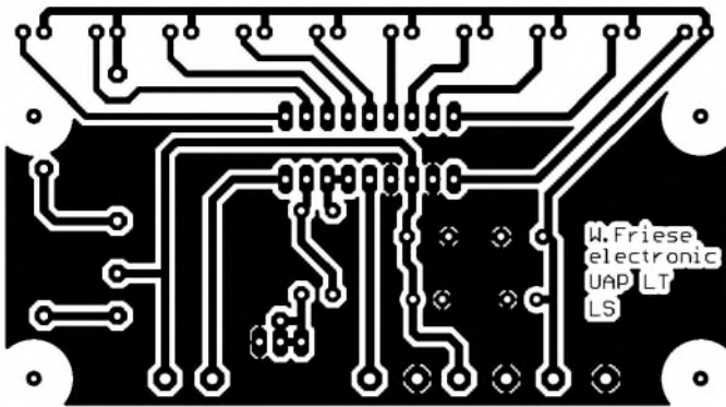
Bild 64: Leiterseite der Platine UAP LT im Maßstab 1:1
