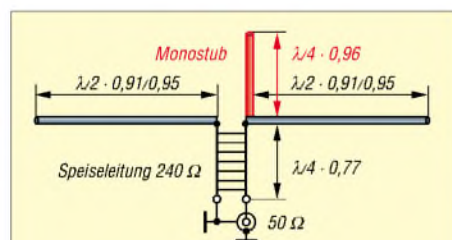
Bild 1: Der Ganzwellendipol mit „Monostub“ benötigt keinen Balun.
