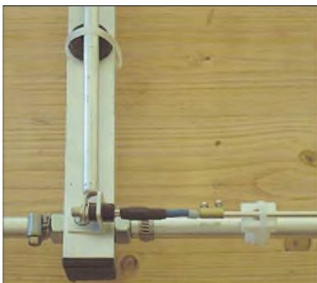
Bild 6: Isoliert angebrachte Telefonbuchse am Boom mit angeschlossenem 6-mm-Phasenleitungsrohr
