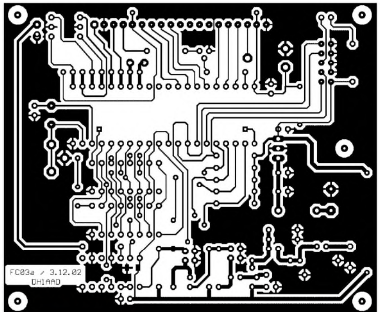
Bild 5: Ein Blick auf das Layout der einseitig beschichteten Platine verdeutlicht die nachbaufreundliche Gestaltung, sodass der Aufbau einfach möglich sein sollte.
