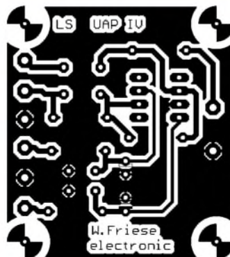
Bild 78: Leiterseite der Platine UAP IV im Maßstab 1:1
