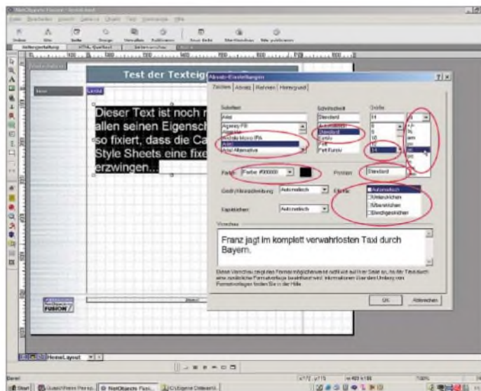
Bild 12: Erst nach manueller Festlegung aller (im Bild markierten) Textformateigenschaften werden diese für das momentan aktive Objekt (und zwar nur für dieses!) in den CSS fixiert.
