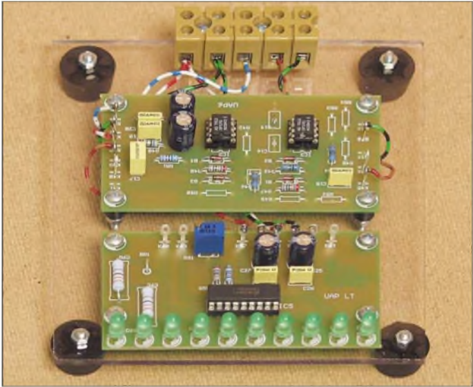
Bild 74: Die Platinen UAP6 und UAP LT ergeben ein gutes Gespann mit vielen Möglichkeiten. UAP6 kann dabei sowohl als Gleichrichterschaltung als auch als Summierverstärker mit invertierender Folgestufe zum Einsatz kommen, siehe Tabelle S. 905.
