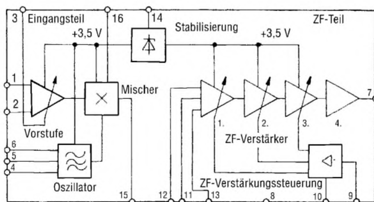
Bild 1: Blockschaltbild des A244/TCA440
