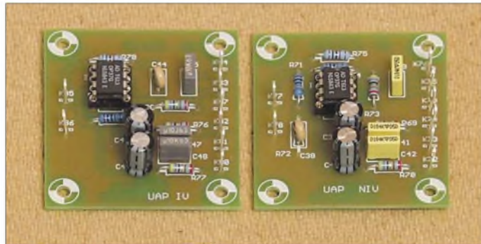
Bild 75: Die zwei kompakten Verstärkerplatten UAP IV und UAP NIV lassen sich u.a. im Zusammenwirken mit UAP LT verwenden.
