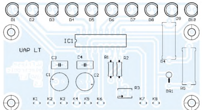
Bild 65: Bestückungsplan der einseitigen Platine UAP LT
