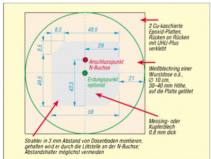
Bild 10: Patch-Feeder, von hinten in Strahlrichtung betrachtet
