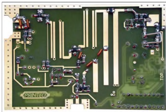
Bild 1: Auf der analogen Seite der bestückten Konverterplatine sind die in Streifenleitertechnik realisierten Filter und Stubs gut zu erkennen.
