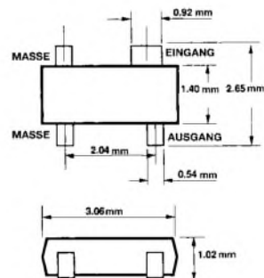
SOT-143
