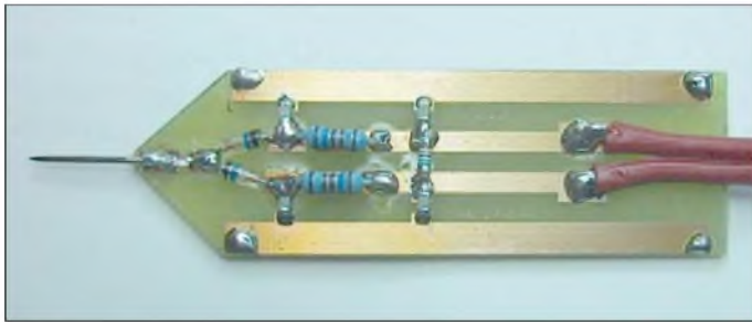
Bild 1: Fast fertiger HF-Tastkopf vor dem Einbau in das Gehäuse. Noch nicht montiert sind die Federbleche zur Verbindung mit dem Metallrohr. Foto: OE2TZL
