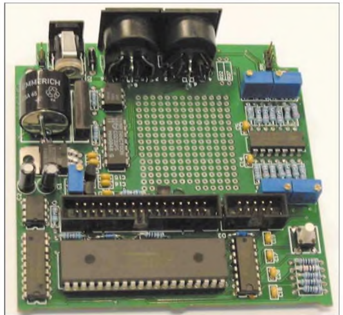
Bild 2: Leiterplatte des fertig bestückten Auroramonitor
