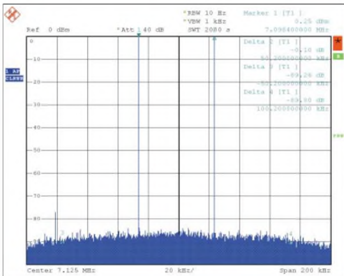
Bild 5: Überprüfung des Messgenerators an einem kommerziellen Spektrumanalyzer. An den Stellen der Marker 3 und 4 liegen die IM-Produkte der Messeinrichtung im Rauschen. Der intermodulationsfreie Dynamikbereich beträgt mindestens 92 dB.
