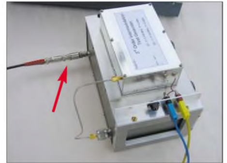
Bild 2: Seitenansicht des Testgenerators mit darunter angeordnetem Dämpfungsglied. Zur Bestimmung des Empfänger-Grundrauschens sind zusätzliche Festdämpfungsglieder aufzustecken (Pfeil).
