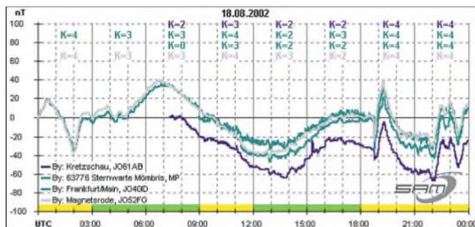
Bild 4: Im Vergleich von vier Magnetogrammen schneiden die drei selbstgebaute Messgeräte (grüne und blaue Kurven) in puncto erreichbare Genauigkeit sehr gut ab. Kurven der besseren Sichtbarkeit halber z.T. v. sich gegeneinander verschoben.
