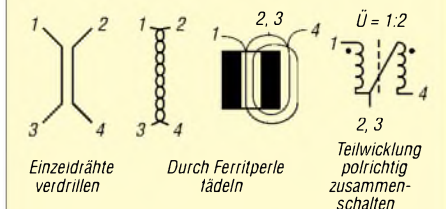
Bild 25: Wickelschema eines Leitungs-Übertragers mit Z_{\bar{u}} = 1:4
