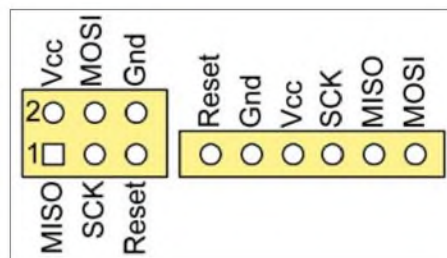
Bild 86: WinAVR- und Atmel-Programmieradapter
