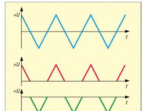
Bild 111: Symmetrische Ausgangssignale in der Betriebsart „Dreiecksspannung“ bei den drei Schalterstellungen von S2 aus Bild 108
