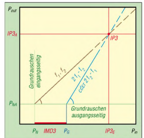
Bild 6: IP3 , Grundrauschen P_N und IM-freier Dynamikbereich IMD3; IP3 lässt sich wegen viel zu hohen Pegels nicht direkt messen, sondern nur berechnen, siehe Kasten.
