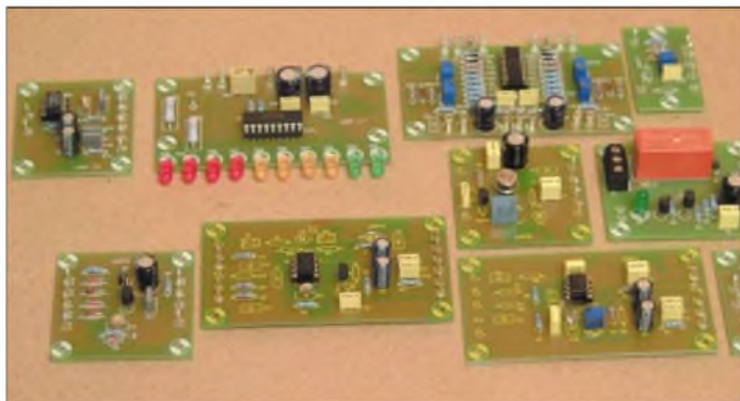
Bild 101: Einige bestückte UAP-Platinen; man kann schon an der unterschiedlichen Bestückung die Vielseitigkeit des Systems erkennen. UAP1, zweite Platine vorn von rechts mit dem Glühlämpchen, ist als klirrarmer Wien-Brücken-Oszillator bestückt.
