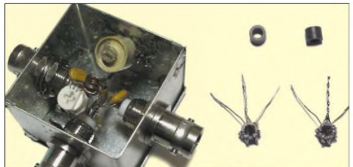
Bild 29: Praktisch aufgebauter modifizierter 3-dB-Power-Splitter; rechts daneben bifilar bewickelte Ringkerne Fotos: DC4KU
