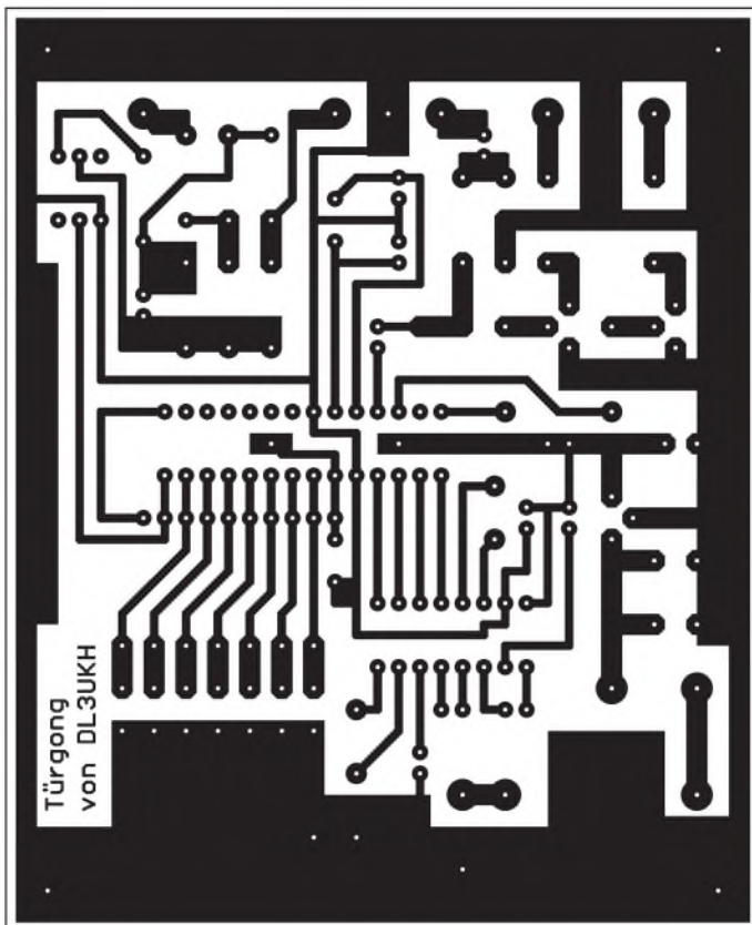
Bild 5: Layout der Steuerleiterplatte
