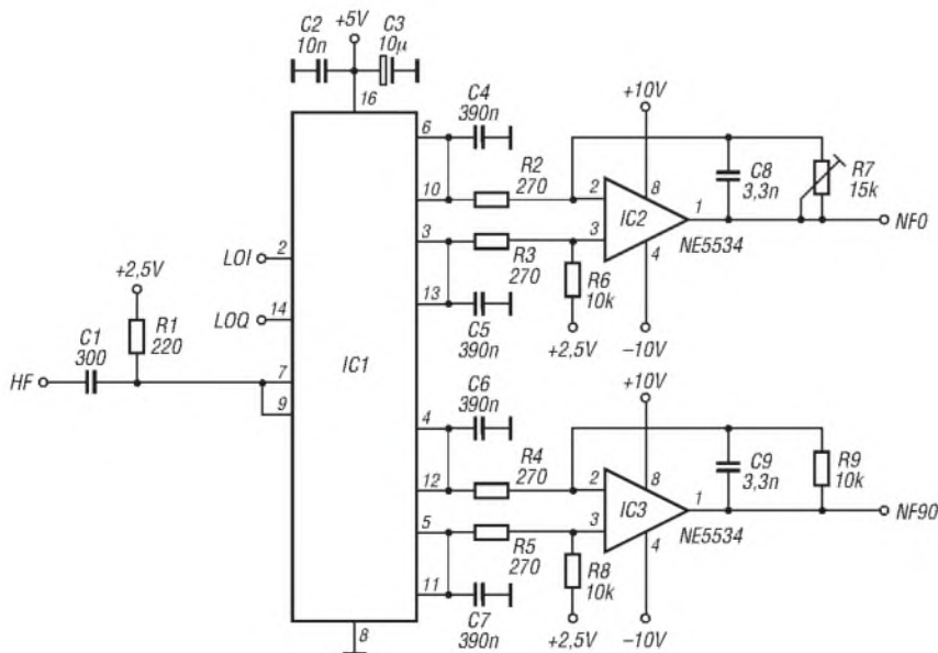
Bild 4: Taylor-Mischer mit einem FST3253; als Lokoszillator sind zwei um 90^\circ phasenversetzte Signale erforderlich.
