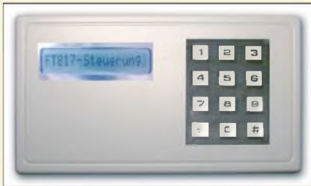
Gerade für den schnellen und gezielten Frequenzwechsel bietet sich diese Tastatur an, mit der sich der Yaesu FT-817 nachrüsten lässt.
