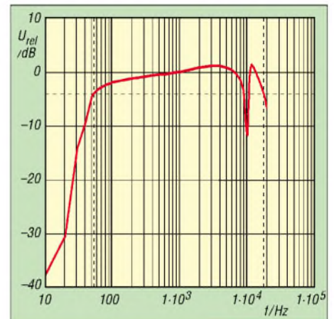
Bild 10: Frequenzgang des ELV413
