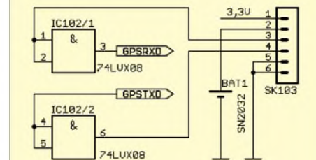
Bild 11: Zur Pegelanpassung zwischen GPS-Modul und Controllerbaugruppe verwenden wir eine Hälfte des 74LVX08.
