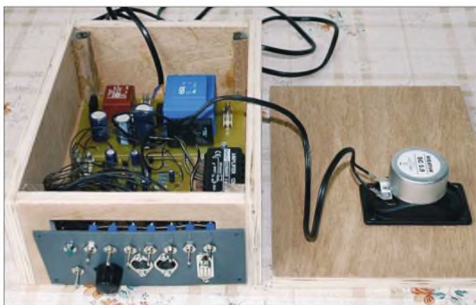
Bild 1: Die Melodieklänge ist möglichst in ein Holzgehäuse einzubauen, da es einen guten Klang wiedergibt und hohen Berührungsschutz bietet.
