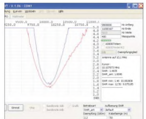
Die Software LinNWT/WinNWT hat jetzt eine wählbare SWV-Skala. Ferner berechnet sie aus gemessenem SWV (rote Kurve) und einzugebenden Kabeldaten auch das SWV an der Antenne (blaue Kurve). Screenshot: -rd
