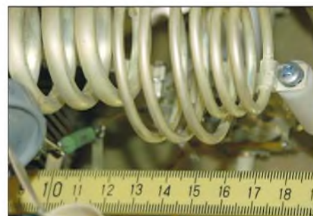
Bild 4: Viel hilft viel – besonders bei 50 MHz muss dem Skin-Effekt Rechnung getragen werden.
