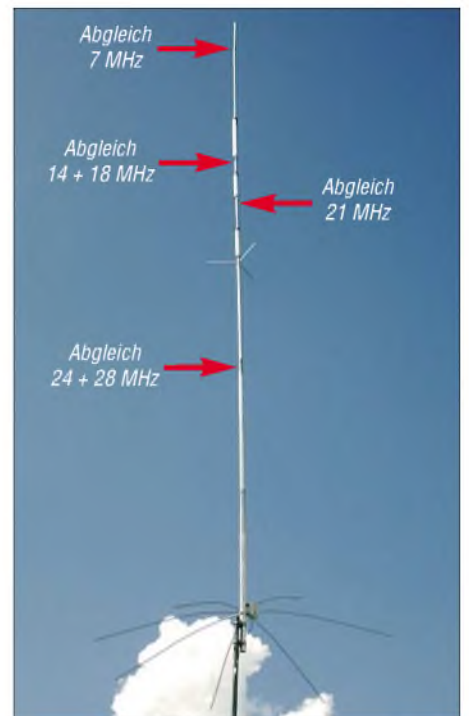
Bild 2: Die Drahtspeichen am Einspeisungspunkt der V7+ sind so dünn, dass sie auf dem Bild zur besseren Erkennbarkeit verstärkt wurden. Die als Abgleichpunkte gekennzeichneten Rohrstücke lassen sich ineinander verschieben und mit Schlauchschellen in der eingestellten Länge fixieren.
