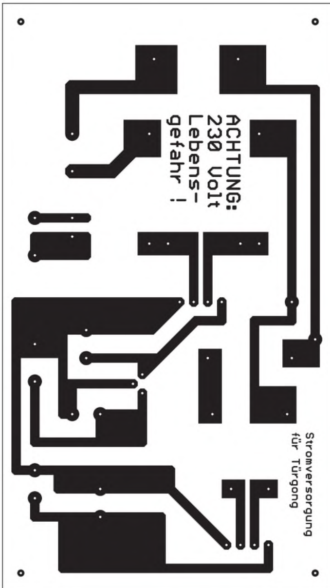
Bild 7: Layout der Stromversorgungsplatine
