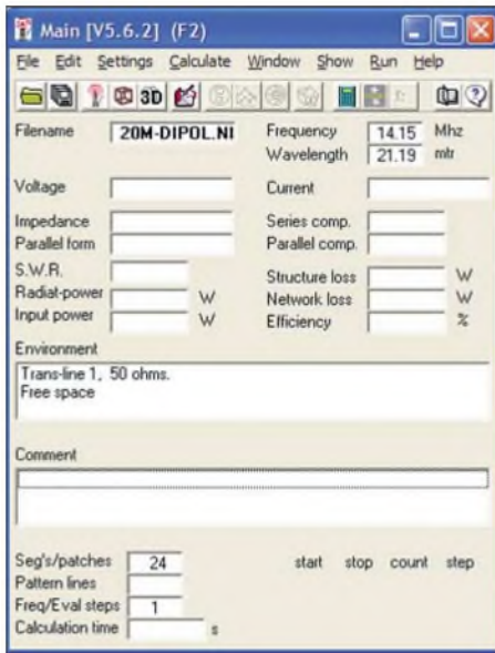
Bild 1: Hauptfenster F2 von 4NEC2; das Verzeichnis bereits definierter Antennen wird durch Anklicken des Punktes File (links oben) erreicht. Der Dateiname der dann ausgesuchten Antenne (hier 20m-Dipol.nec) ist unter Filename zu finden. Nach dem ersten Rechengang füllen sich die Leerfelder mit Zahlenwerten.
