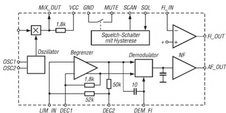
Bild 1: Blockschaltbild des MC3361P/MC3361C
