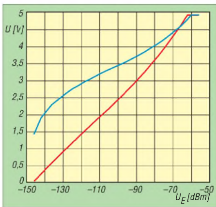
Bild 4: Spannungen am S-Meter-Ausgang (rot) und am Pulse-Ausgang (blau) als Funktion des Eingangspiegels
