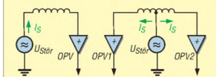
Bild 12: Wirkung von hochfrequenten Störungen, die durch die Netzversorgung bzw. die Erdanbindung verursacht werden, siehe Text
