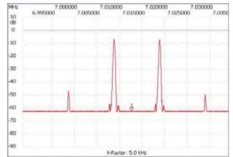
Bild 8: Ermittlung des IM3-Verhaltens des SAV mit 7015- und 7025-kHz-Quarzoszillatoren
