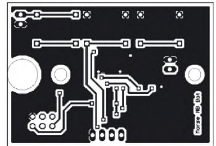
Bild 4: Layout der Unterseite der Leiterplatte, auf der nur die Steckverbinder festgelötet werden; die Platine ist 54 mm × 38 mm groß.
