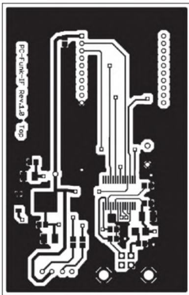
Bild 6: Layoutoberseite des USB-Interfaces; Abmessungen 79 mm × 51 mm
