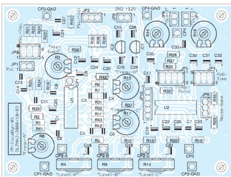
Bild 12: Bestückungs- plan
