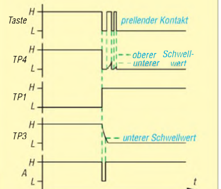
Bild 5: Taktimpulserzeugung bei prellendem Kontakt
