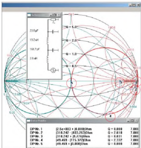
Bild 23: Anpassung mit einem Pi-L-Glied auf 7 MHz; wiederum mit eingezeichneten Kreisbögen konstanter Betriebsgüte
