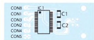
Bild 14: Bestückung der Platinoberseite mit dem USB-Schnittstellenschaltkreis
