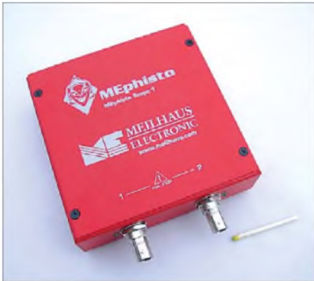
Bild 1: Mephisto Scope UM203 mit autark nutzbarem Datenlogger
