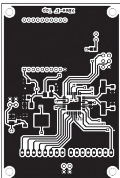
Bild 9: Layoutoberseite der Controllerplatine; Abmessungen 79 mm × 53 mm
