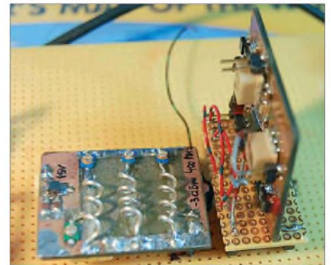
Bild 13: Die DDS-Baugruppe im Versuchsaufbau
