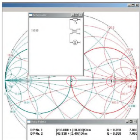
Bild 24: Anpassung mit einem 1:4-Transformator
