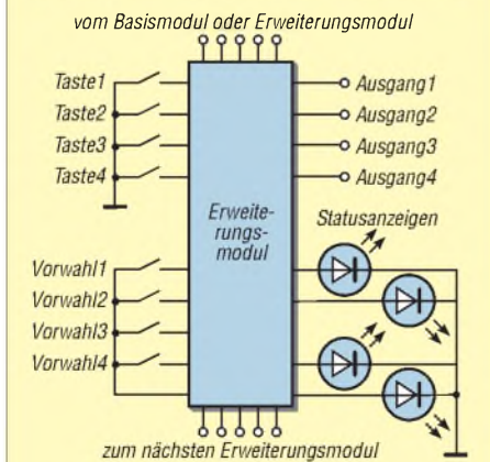
Bild 2: Blockschaltbild des Erweiterungsmoduls
