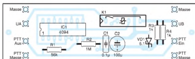
Bild 4: Bestückungsplan; es kommen nur bedrahtete Bauteile zum Einsatz.
