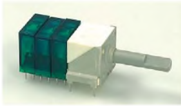
Bild 5: Miniaturdrehschalter mit drei Schaltkammern und Rastkopf mit 20 mm langer Achse bei lückenloser Anordnung der Schaltkammern
