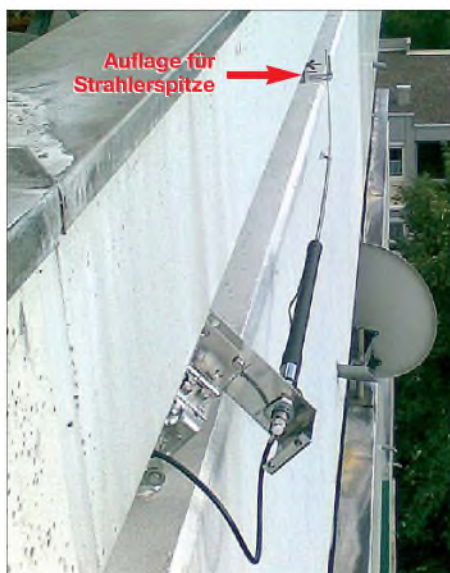
Bild 2: Die Antenne lässt sich bei Betriebsruhe an den Balkon klappen.
