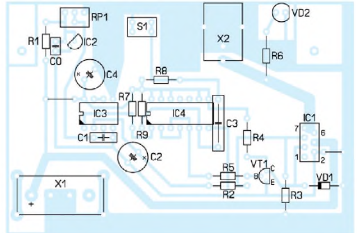
Bild 9: Bestückung der Leiterplatte für die Schutzschaltung 2; der dreipolige IC2 ist nur mit zwei Anschlüssen einzulöten.
