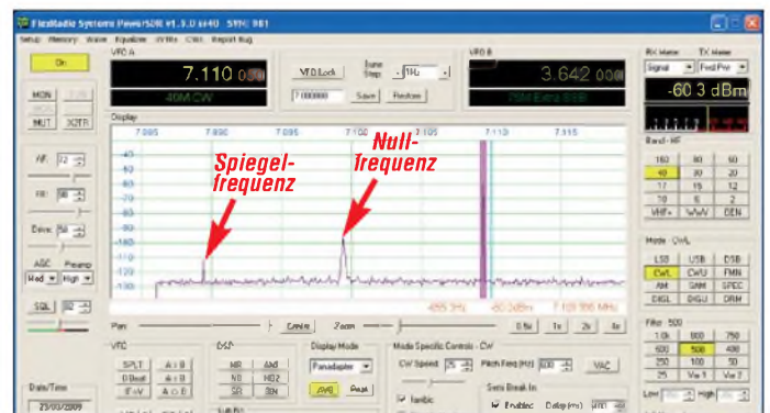
Bild 2: Nutzsinal ohne Störsignale mit der USB-Box E-MU 0202 USB am Laptop und Originalschaltenteil
