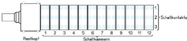
Bild 8: Leiterführung und Bestückung eines Miniaturdrehschalters mit zwölf Schaltkammern
