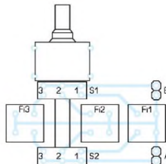
Bild 12: Leiterführung und Bestückung für einen Miniaturdrehschalter mit zwei Schaltkammern; beide Kammern fungieren als getrennte Schalterebenen, da sie nicht versetzt gegeneinander auf die Welle geschoben sind und ihre Kontakte somit bei Betätigung des Rastkopfes gleichzeitig schließen.
