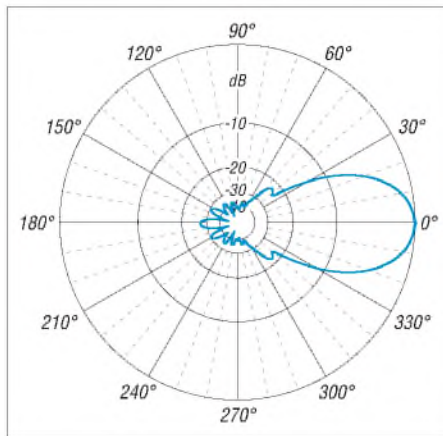
Bild 6: Azimut-Diagramm der Elfelement-G0KSC-Yagi-Antenne
