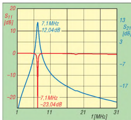
Bild 6: Selektion des Preselektors auf 40 m – stellvertretend für die anderen Bänder; die rote Kurve zeigt die sehr gute Anpassung an 50 \Omega und die blaue die Durchlasskurve mit 12 dB Verstärkung auf 7,1 MHz.
