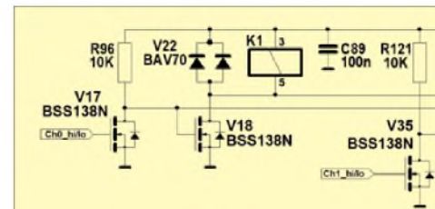
Bild 12: HF-Teil mit dem DDS-IC
