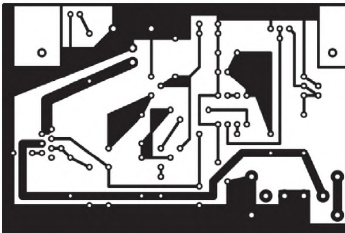
Bild 10: Leiterplatte für die Schutzschaltung 3; Abmessungen 92 mm × 61 mm, M 1:1
