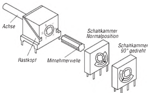
Bild 1: Baukastenprinzip der Miniaturdrehschalter
