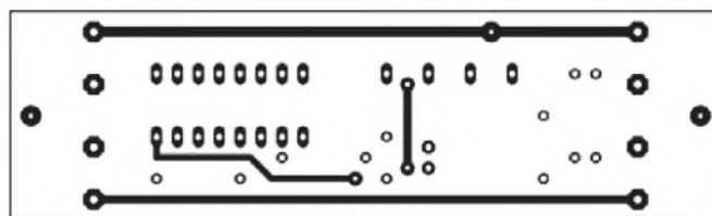
Bild 2: Leitungsführung auf der Platinoberseite; Abmessungen 86,5 mm \times 25,5 mm
