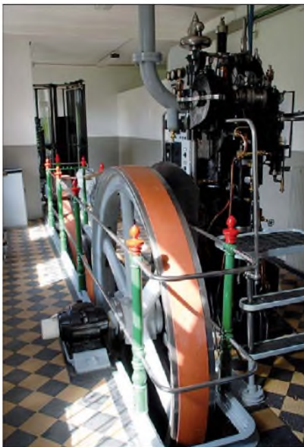
Der 1906 gebaute Dieselmotor mit einer Leistung von 10 kVA (Einzyylinder, 17 l Hubraum)
