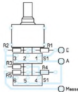
Bild 10: Leiterführung und Bestückung für einen Miniaturdrehschalter mit zwei Schaltkammern; beide Kammern fungieren als eine Schalterebene, da sie um 90° versetzt gegeneinander auf die Welle geschoben sind und ihre Kontakte somit bei Betätigung des Rastkopfes nacheinander schließen.
