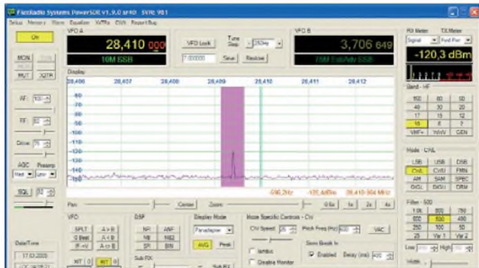
Bild 5: Empfangsbildschirm mit einem Eingangssignal von -120 dBm (0,225 \mu V an 50 \Omega ) auf 10 m; das Grundrauschen liegt bei etwa -145 dBm, das Nutzsignal ragt deutlich heraus.
