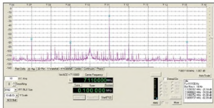
Bild 9: Ausgangsspektrum in der Nähe der Nutzfrequenz; der Träger liegt bei 7,100 MHz, das Nutzausgangssignal bei 7,110 MHz.* Auf 7,07 MHz und auf 7,15 MHz sind IM-Produkte erkennbar, die der Mischer erzeugt.
