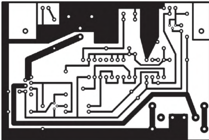
Bild 8: Leiterplatte für die Schutzschaltung 2; Abmessungen 92 mm × 61 mm, M 1:1
