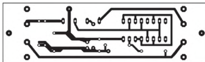
Bild 3: Leitungsführung auf der Platinenunterseite; Maßstab 1:1
