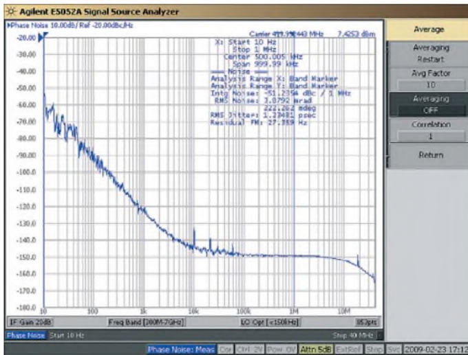
Bild 11: Phasenrauschen des modifizierten Driscoll-Oszillators hinter dem Frequenzvervielfacher
