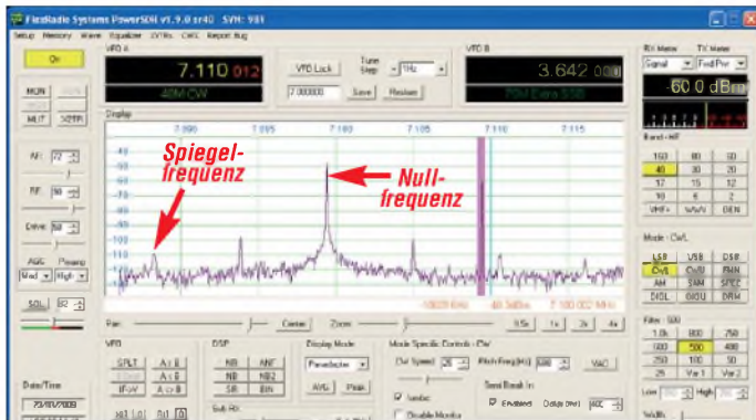
Bild 1: Nutzsinal (violett) und Störsignale mit der Onboard-Soundkarte mit dem AC97-Soundchip und Originalschaltenteil
