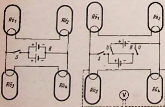
Bild 1. Heizung zweier parallel geschalteter Röhrenguppen (Rö 1 , Rö 2 ; Rö 3 , Rö 4 ) aus zwei Taschenlampenbatterien B (Heizstromentnahme je Batterie 60 mA, S = Heizstromschalter).
