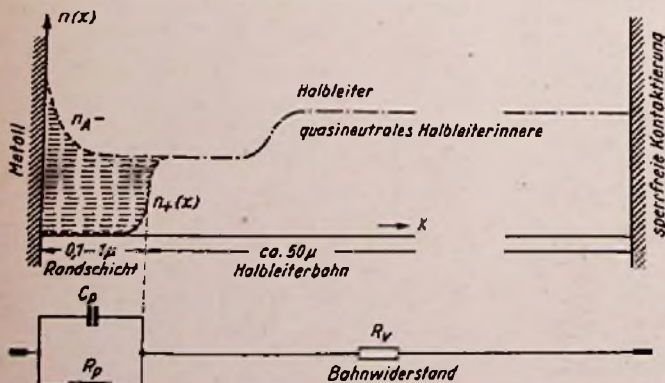
Bild 3. Aufbau eines Randschichtgleichrichters. Oben: Störstellendichte innerhalb des Halbleiters (Defektleitung), unten: elektrisches Ersatzbild (nach Dr. Arnulf Hoffmann).
