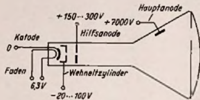
Bild 62. Grundsätzliche Elektrodenanordnung bei normalen Bildröhren
