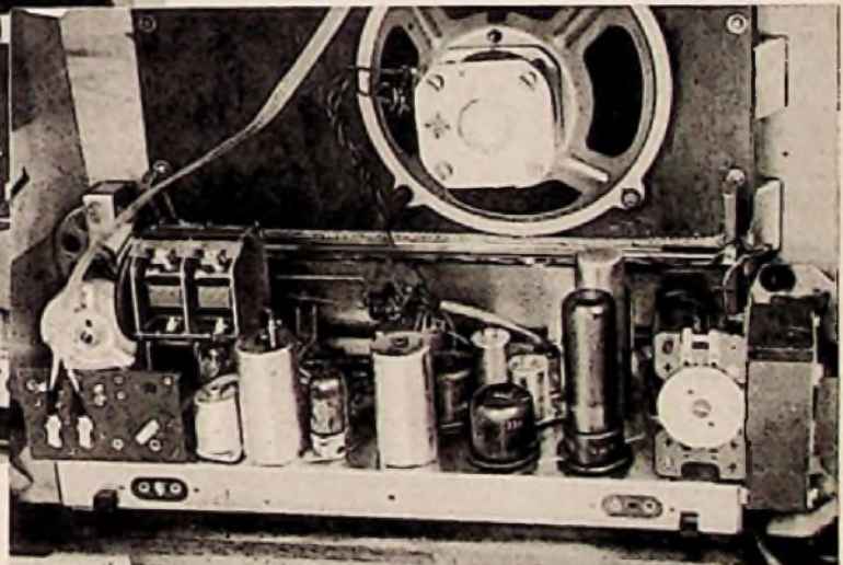
Charakteristisch für die Innenausstattung zahlreicher AM-FM-Superhets ist der Einbau einer UKW-Innenantenne, die auch der Telefunken 7/8-Kreis-Super „Operette 52“ verwendet. Das Bild zeigt allerdings nur die Zuleitung
