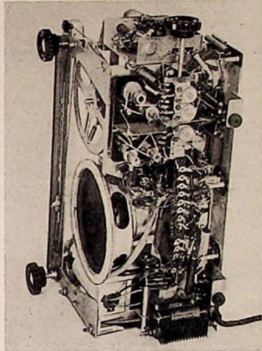
Die Verdrahtungsansicht des Lorenz „Wendelstein U“ zeigt einen sorgfältig überlegten Aufbau
