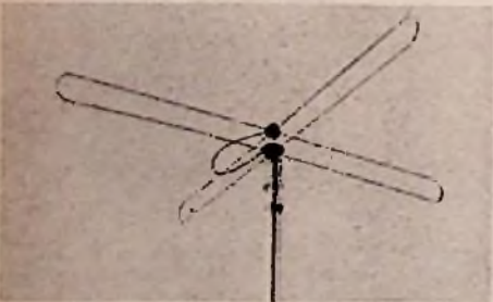
Runddipol mit Rohrbefestigung für Dachmontage von Dr. Reif
