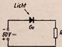
Bild 4. Schaltung der Fotodiode 1 N 77
