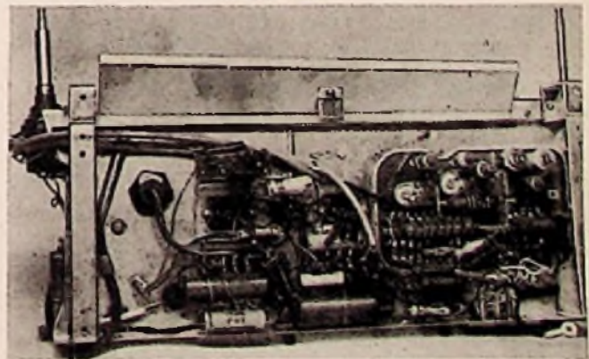
Verdrahtungsansicht des Telefunken „Kurier 52“
