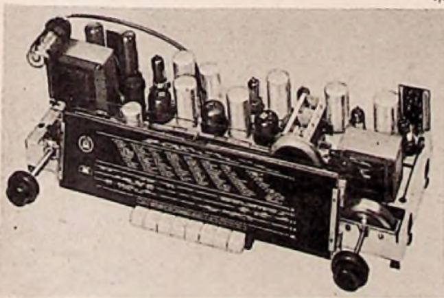
8/9-Kreis-Drucktastensuper mit 10-Watt-Gegentaktendstufe (Metz 520)
