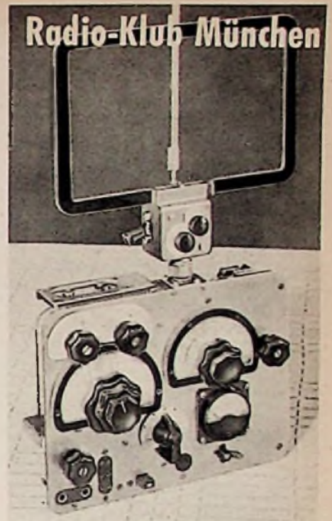
Bild 1. 80-m-Peilempfänger mit eingebautem 2-m-Transceiver
