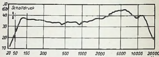
Bild 5. Schalldruckverlauf des Lorenz-Ovallautsprechers LP 1725/19/90 R
