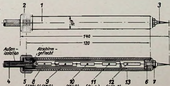
Bild 2. Aufbau des Tastkopfes
