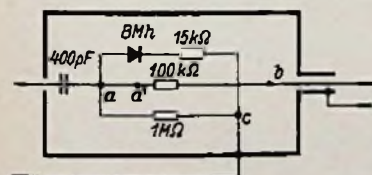
Bild 1. Schaltung des Tastkopfes
