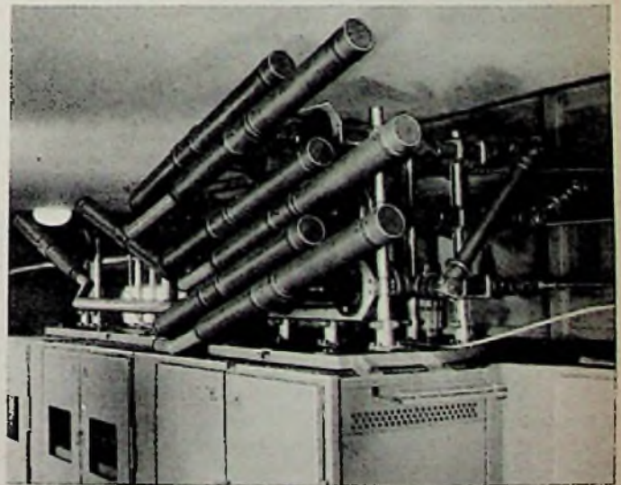
Kein Raketenwerfer, sondern das Einseitenbandfilter des neuen Lorenz-Fernsehsenders auf dem großen Feldberg. Es unterdrückt, wie der Name andeutet, das eine Modulations-Seitenband der Bildsenderfrequenz. Eine weitere Einrichtung, der Diplexer (links im Hintergrund), entkoppelt Bild- und Tonsender, so daß sie gemeinsam an eine Antenne angeschlossen werden können. Beide Einrichtungen sind in einer neuartigen Technik als „Brücken“ in Form koaxialer Ringleitungen ausgeführt
