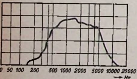
Bild 7. Frequenzkurve des Ultratone-Kommandolautsprechers
