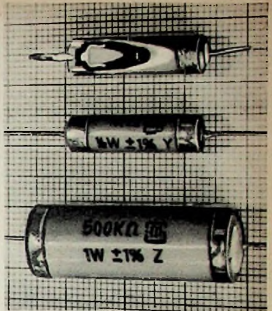
Hermetisch abgeschlossene Präzisions-Schichtwiderstände der Steatit-Magnesia-AG.
