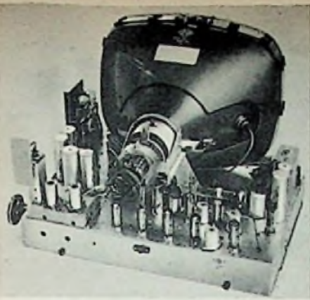
Bild 5. Chassis des Telefunken FE 9. Man beachte den Platz des Kanalschalters (links außen)
