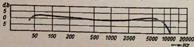
Bild 1. Frequenzkurve des Bändchenmikrofons M 31 von Beyer
