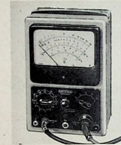
Grundig-Universal-Röhrenvoltmeter
