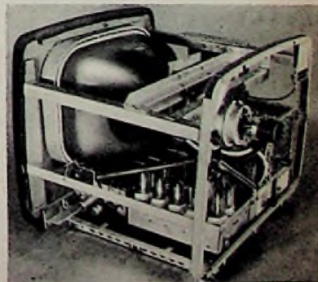
Bild 3. Interessante Rahmenkonstruktion der neuen Philips-Fernseh-Tischempfänger. Chassis und Frontplatte bilden eine Einheit
