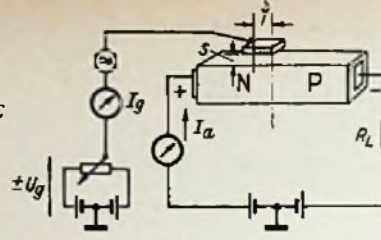
Bild 4. p-n-Feldistor
