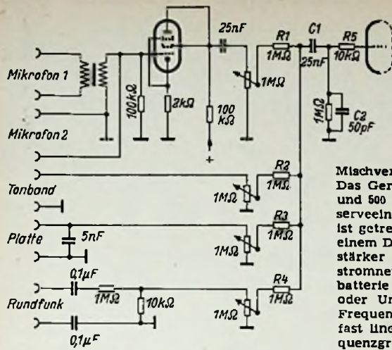
Bild 10. Eingangsschaltung eines modernen Kraftverstärkers (Tekade)
