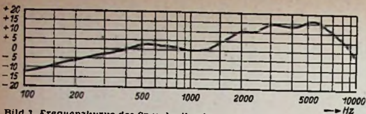
Bild 3. Frequenzkurve des Sprachmikrofons MD 7 (Labor Wennebostel)
