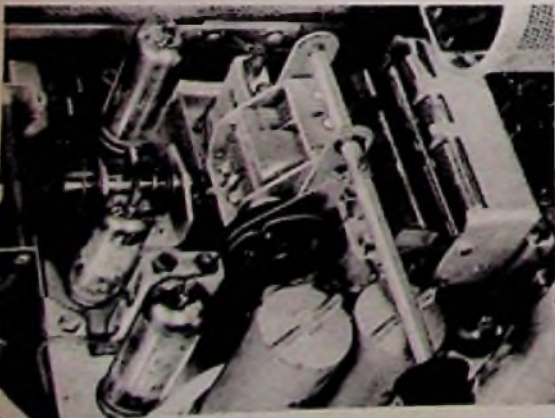
Links: Bild 2. Drei Drehkondensator-Aggregate in einem Gerät. Links: UKW-Drehkondensator, Mitte: Drehkondensator für die „Ortstaste“, rechts: Drehkondensatorpaket für die AM-Abstimmung (Philips-Uranus 53)
