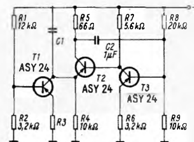
Bild 1. Prinzipschaltbild des Kippgenerators
