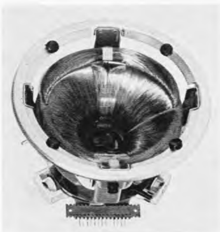
Bild 3. Ablenk- und Konvergenzeinheit für Farbbildröhren ohne Permanentmagnete zum Einstellen der statischen Konvergenz (Video)
