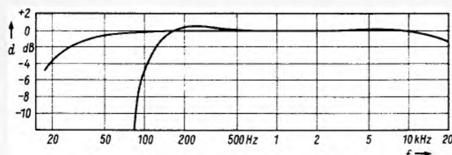
Bild 4. Die Frequenzkurve des Trittschallfilters
