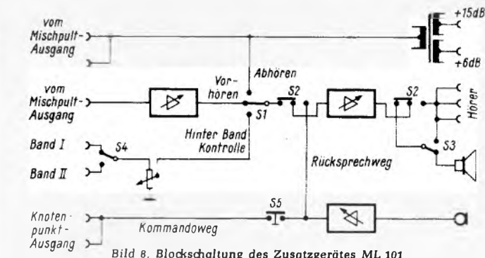
Bild 8. Blockschaltung des Zusatzgerätes ML 101
