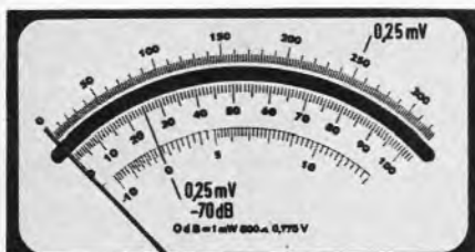
Bild 4. Der Spannung 0,25 mV (Meßbereich 1 mV nach Bild 3) entspricht der Spannungspegel p = - 70 dB
