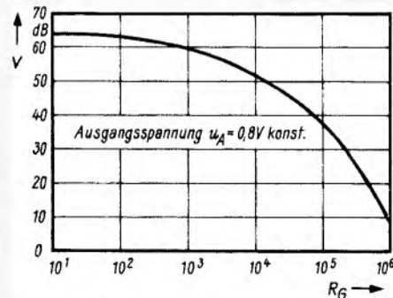
Bild 2. Spannungsverstärkung der Schaltung nach Bild 1 in Abhängigkeit vom Innenwiderstand der Signalquelle
