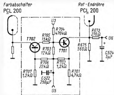
Aurenmat nennt Telefunken eine seit der Hannover-Messe eingeführte Schaltung für Farbfernsehgeräte, durch die das Schwarzweißbild eine leichte Blautönung, das Farbbild jedoch eine leichte Rottönung erhält
