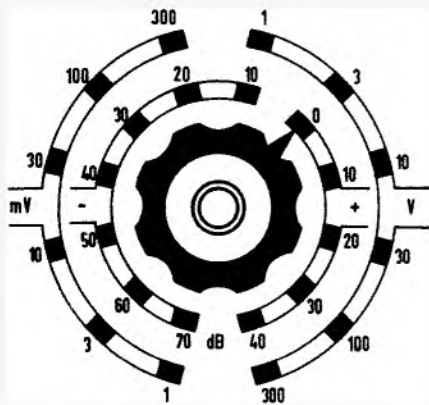
Bild 3. Meßbereichschalter eines elektronischen Spannungsmessers
