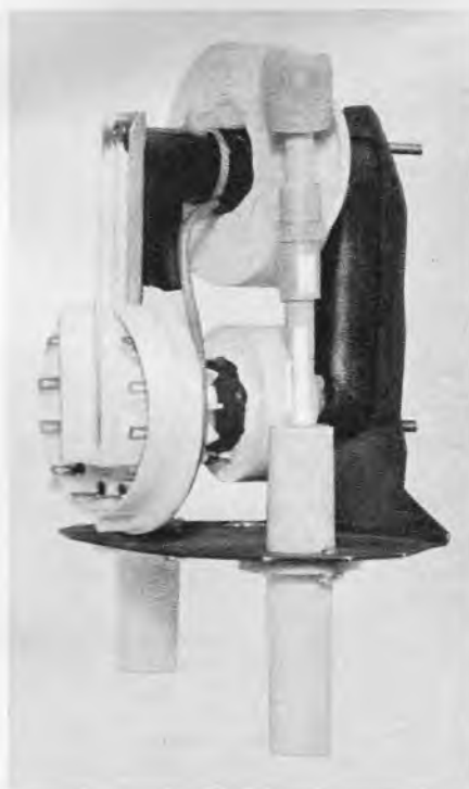
Bild 2. Hochspannungs-Transformator für transistorbestückte Farbfernsehempfänger mit zwei Einneggleichrichtern für 7 kV und 25 kV (Videon)
