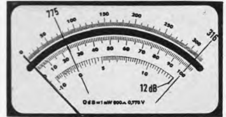
Bild 2. Anzeigeteil eines elektronischen Spannungsmessers mit zusätzlicher dB-Skala
