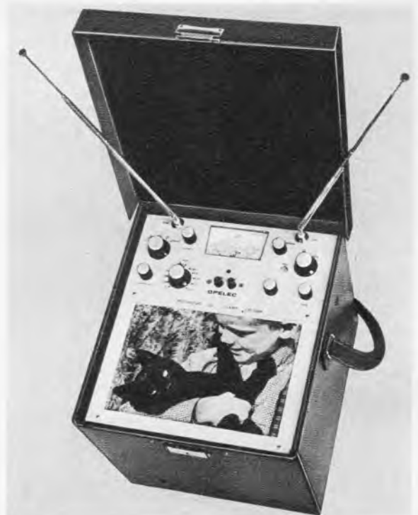
Bild 1. Ein besonders handliches Antennenmeßgerät von Opelec, einstellbar auf die Kanäle F 2 bis F 12 im VHF-Bereich sowie auf alle Kanäle im UHF-Bereich bis 825 MHz (Modell OP 728 F)
