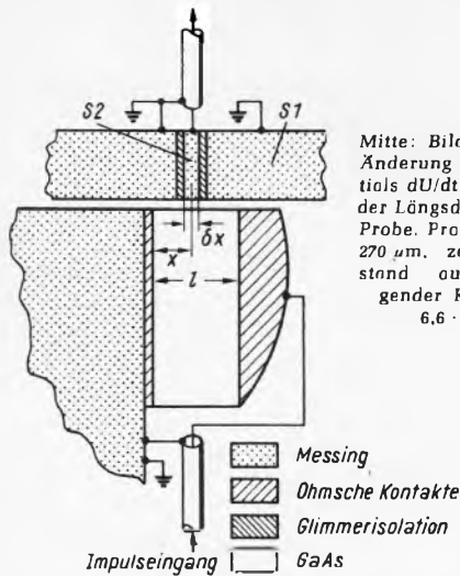
Bild 3. Messanordnung mit kapazitiver Sonde
