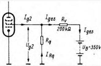
Bild 3. Schirmgitterkreis einer Nf-Stufe
