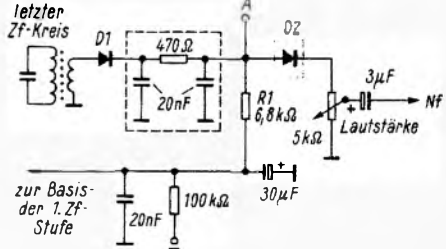
Schaltung einer Rauschperre für Funksprechgeräte
