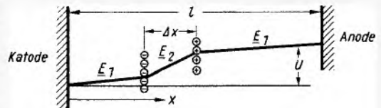
Bild 6. Negativwiderstands-Domäne einer GaAs-Probe
