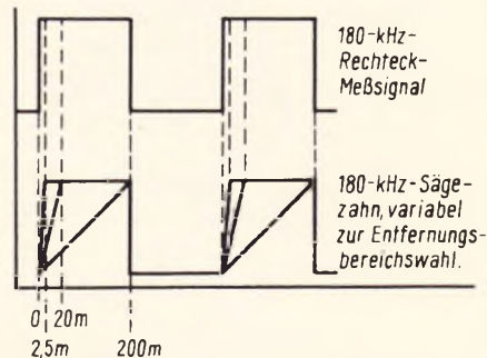
Bild 7. Entfernungsbereichswahl im Empfangsteil (nicht maßstabgetreu)
