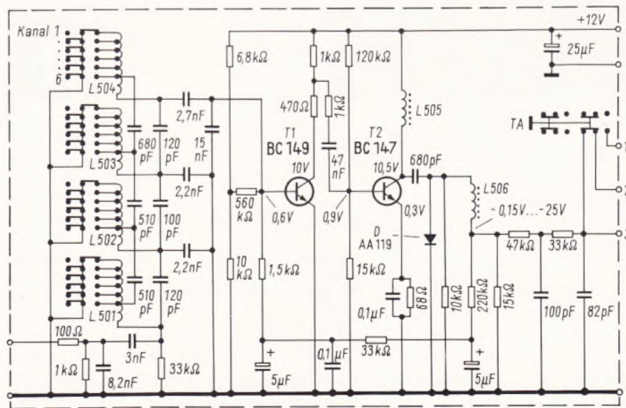
Schaltung des Hf-TR-Empfangsvorsatzes Sondyna 6739.01 (Walzenform mit Schalter) oder 6839.02 (flache Form mit Drucktasten)
