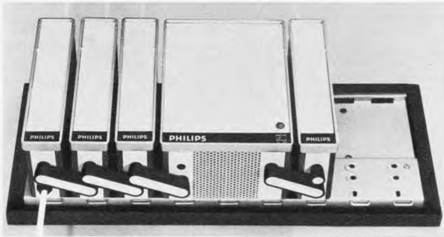
Bild 5. Montageschiene mit Netzteil und gemischter Bestückung mit Star- und Super-Star-Verstärkern
