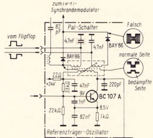
Bei Fehlern im Pal-Schalter tritt oft der sogenannte Jalousie-Effekt auf. In dem fehlerhaften Gerät hatte der gekennzeichnete 4,7-nF-Kondensator einen Feinschluss
