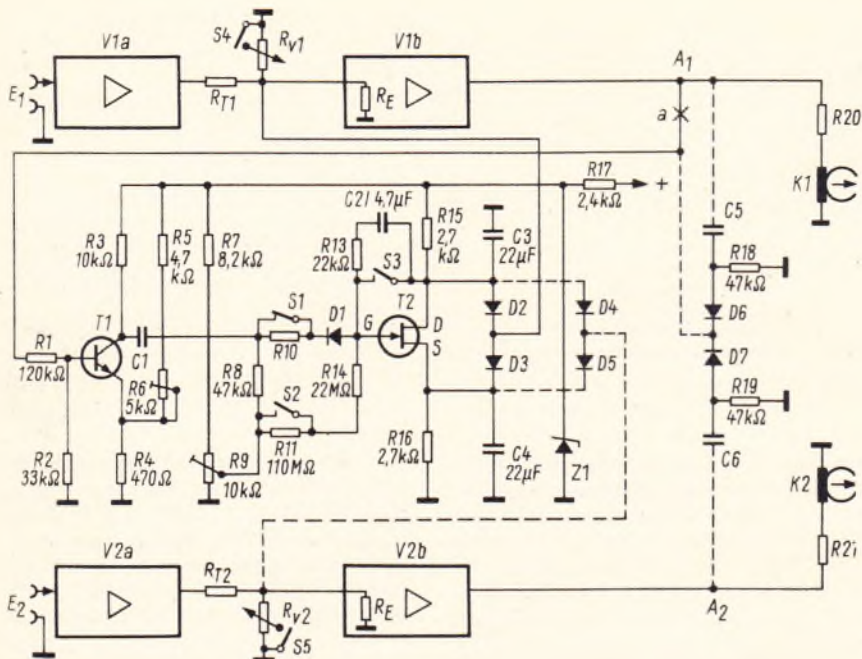
Bild 7. Gesamtschaltbild einer Regelaomatik für Grundig-Tonbandgeräte in Mono- und Stereo-Version
