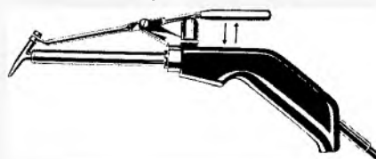
Bild 10. Entlötspistole Pico 3481 von Lötring. Der obere Hebelgriff wird nach unten gedrückt und die Kolbenspitze auf die Lötstelle gesetzt. Beim Loslassen des Hebels drückt der Stahlraht durch die Spitze hindurch und damit das Bauelement aus der Lötstelle heraus
