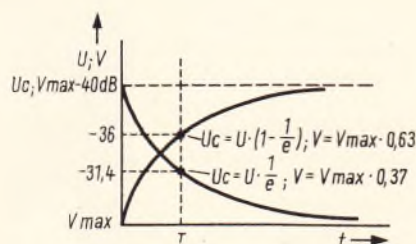
Bild 1. Auflade- und Entladekurve des Kondensators ( U_C ) eines RC-Gliedes mit der Definition der Zeitkonstante T = R \cdot C . Analog dazu der Verstärkungsverlauf ( V ) einer Aussteuerungsautomatik bei einem Regelhub von 40 dB, wobei der Wert T für die Definition der Ansprech- und Abklingzeitkonstante gültig ist
