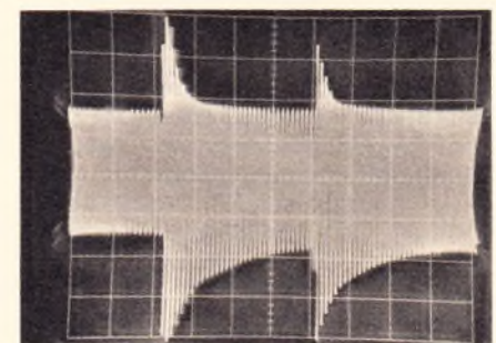
U_e = Vollpegel +20dB +40dB 40 Hz
