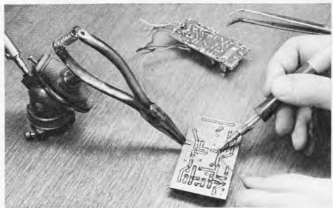
Unten: Bild 11. Selbstgebaute Klemm- vorrichtung aus einem Foto-Neigekopf und einer Justierzange (eine „dritte Hand“)
