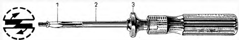
Bild 2. Ausführung eines Festhalte-Schraubendrehers. 1 = geteilte Klinge, 2 = Hülse, 3 = Griff zum Spreizen der Klinge. Links: vergrößerte Darstellung der geteilten Klinge
