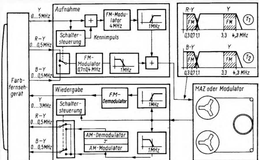
Bild 6. Prinzip einer weiteren Variante zu Bild 4. Y + (R-Y) \leftrightarrow Y + (B-Y)
