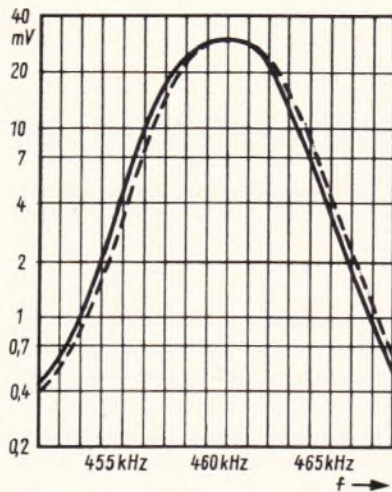
Bild 4. Abgleichkurven eines 3-Kreis-Filters mit Keramikfilter als Koppelglied. f_{res} des Keramikfilters = 461 kHz. Ausgezogene Linie: Abgleich bei 460 kHz. Gestrichelte Linie: Abgleich bei 462 kHz
