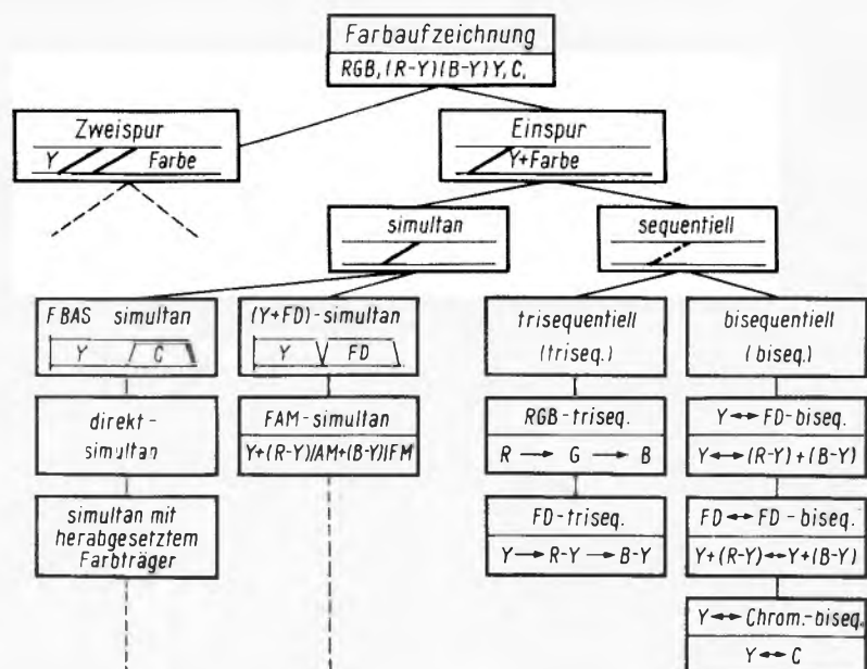
Bild 1. Übersicht über die verschiedenen Farbaufzeichnungsprinzipien
