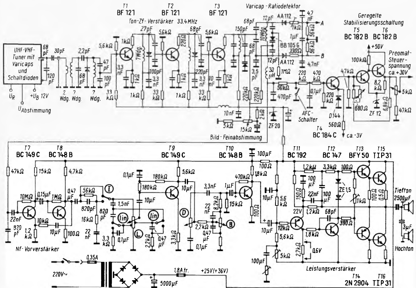
Bild 2. Schaltung des Tonkanals und der Regelstufen für Bild und Ton im „Hi-Fi-Vision“. Lin = Lineartaste, I = Intimtaste, D = Diskant, B = Baß, L = Lautstärke
