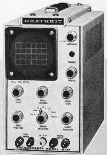
7-cm-Breitband- Kleinoszillograf IO-17*
