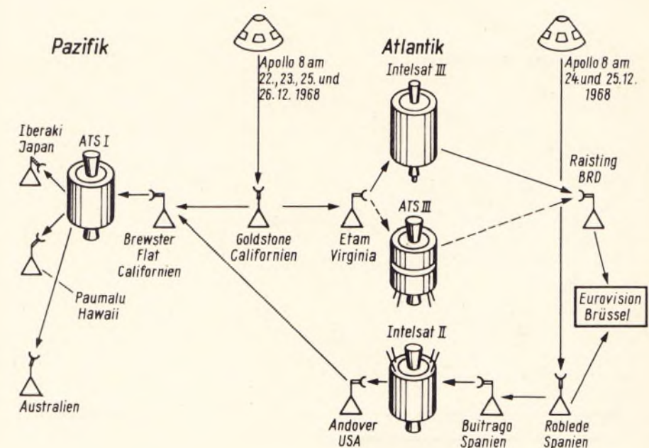
Bild 1. Weltweites Verteilernetz der Fernsehaufnahmen aus dem All während einer Apollo-Mission, dargestellt an den Verhältnissen während des Apollo-8-Fluges
