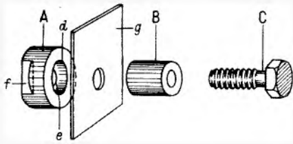
Links: Bild 4a. Die Teile des Record-Lochers: A = Gegenstück mit Gewinde, B = Stempel, C = Gewindeschraube, d = Öffnung des Gegenstückes, in das der Stempel eindrückt, e = Gewinde, f = Flächen für Schraubstock oder Schraubenschlüssel, g = zu stanzendes Werkstück
