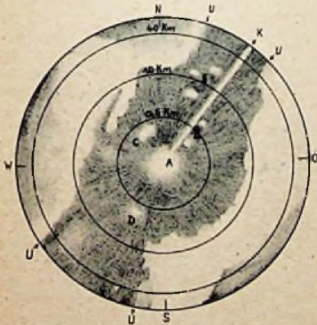
Abb. 1. Beispiel einer Radaranzeige bei Fahrt durch einen breiten Strom. Die dunkle Fläche des Schirmbildes gibt die abgetastete Wasseroberfläche wieder. Es bedeuten: A = Lichtfleck des eigenen Fahrzeuges (Schirmbildmittelpunkt), B = Bojen, C = Fahrzeug auf Backbord, D = Fahrzeug achtern, E = Fahrzeug backbord voraus, K = Kurslinie, U = Uferumrißlinien
