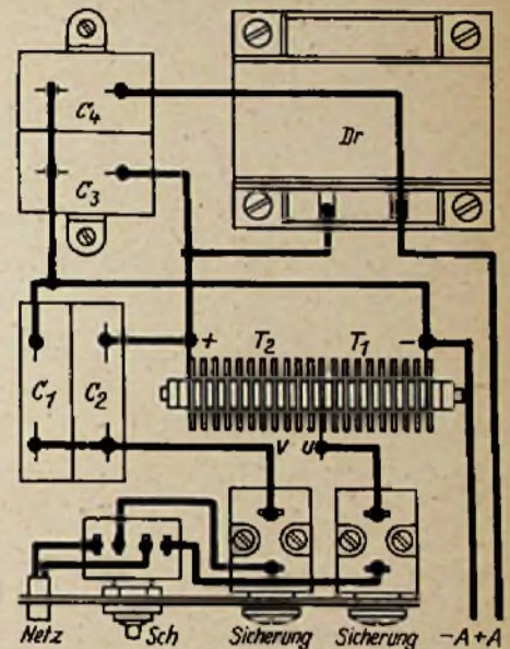
Abb. 5. Schaltplan eines Delon-Gleichrichters
