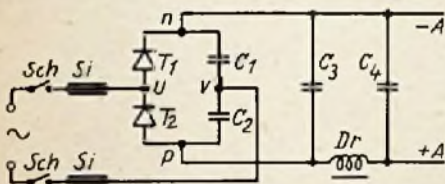
Abb. 1. Schaltbild eines Gleichrichters nach der Delonschaltung
