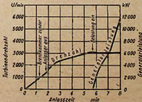
Abb. 2. Anlaßschaubild für ein ausgeführtes zweistufiges Gasturbinenkraftwerk von 12 000 kW
