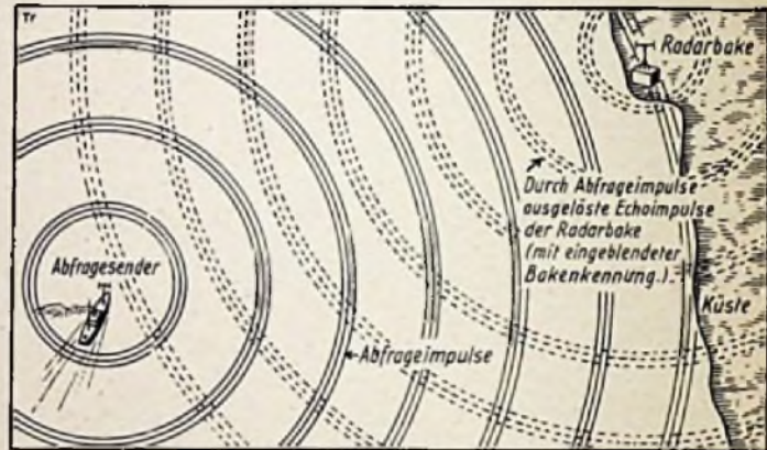
Abb. 4. Schematische Darstellung der Wirkungsweise einer Radarbake. Der Zeitunterschied zwischen Aussenden eines Abfrageimpulses und Empfang des künstlichen Echoimpulses der Bake ist ein Maß für die Entfernung zur Bake. Der Empfang der Echoimpulse mittels Richtantenne liefert außerdem die Richtung, in der die Bake steht. Beides zusammen bestimmt den Standort des Fahrzeuges, auf dem der Abfragesender steht
