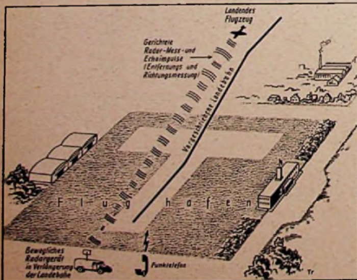
Abb. 3. Radarführung eines landenden Flugzeuges bei schlechter Sicht. In der Darstellung ist das Flugzeug nach der Radarmessung höher, als der vorgeschriebenen Landebahn entspricht. Es erhält daher funktellefonisch die Anweisung „Sinkgeschwindigkeit vergrößern“ Zeichnungen Trester
