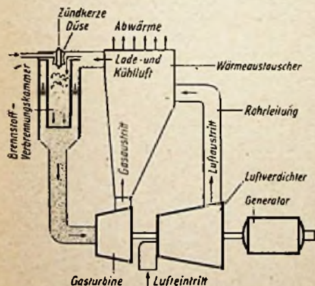
Abb. 1. Grundsätzlicher Aufbau eines Gasturbinenkraftwerkes. Luftverdichter, Gasturbine und Generator auf einer Welle. Kühlung der Brennkammer durch Ladeluft und Vorwärmung der Ladeluft durch entspannte Abgase
