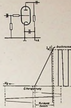
Abb. 3. Erzeugung und Formung von rechteckigen Stromimpulsen in einer Stufe. Oben: Schaltbild. Unten: Verstärkende und begrenzende Wirkung der verwendeten Triade
