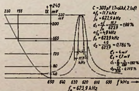
Abb. 6. Resonanzkurve eines Kreises mit Trolitul- bzw. Luftkondensator
