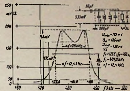
Abb. 7. Resonanzkurve eines Bandfilters
