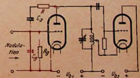
Abb. 23. Frequenzmodulation durch eine Reaktanzröhre
