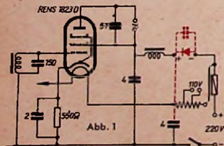
Einfaehes Prüfgerät
