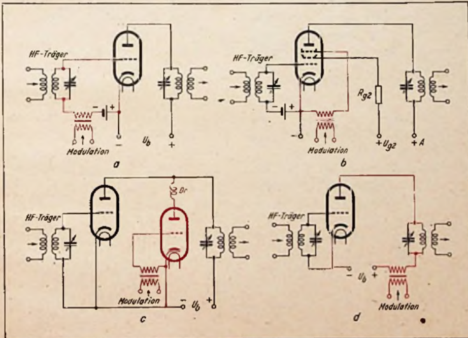
Abb. 21. a) Gitterspannungsmodulator; b) Bremsgittermodulator; c) Anodenspannungsmodulator; d) Anodenstrommodulator
