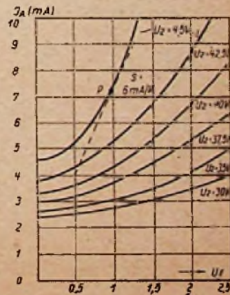
Abb. 7 (rechts). Gleichstrom-Kennlinienfeld des Transistors. (Ströme unabhängig variabel, Spannungen abhängig veränderlich.)
