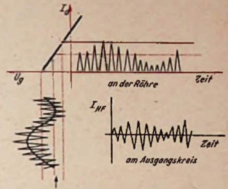
Abb. 22. Der Modulationsvorgang in der Röhre (Gittermodulation)
