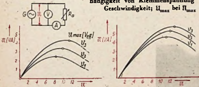
1. Typo: 4 Pole Rechts: 2. Typo: 8 Pole Typenschild: 6,9 V 2,1 VA Typenschild: 10 V 4,5 VA
