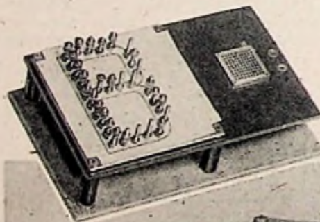
Abb. 1. Tasttableau von unten gesehen
