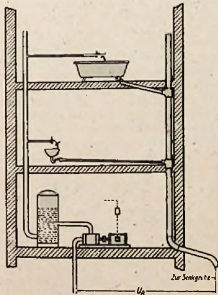
Abb. 2. Berührungsspannungen an den Wasserzapfstellen ( U_B = Berührungsspannung)
