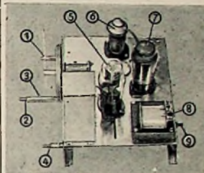
1. Lautstärkeregl. 2. Bereichschalter, 3. Abstimmung, 4. Rückkopplung, 5. Gleichrichterröhre AZ 11, 6. Audionröhre EF 9, 7. Endröhre EL 11, 8. Netztransformator mit Sicherung, 9. Netzschalter
