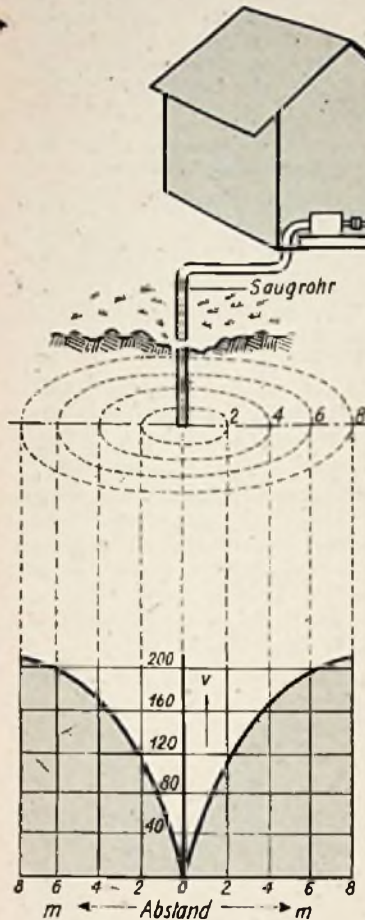
Abb. 1. Schrittspannungen um das Saugrohr bei einer Spannung von 220 V gegen Erde
