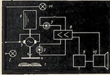
Abb. 5. Blockschema zum zweiten Verfahren.
