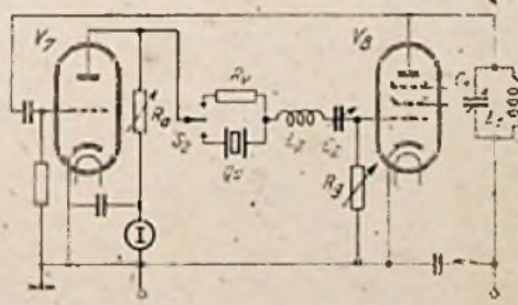
Abb. 6. Abänderung der Heegner-Schaltung zur Messung der Kristalldaten
