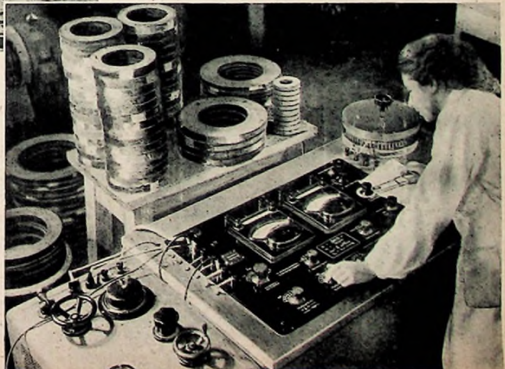
Fertigungskontrolle. Vorbereitungen zur Prüfung von Durchführungs-Meßstromwandlern
