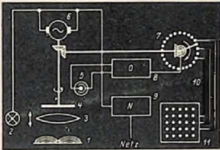
Abb. 4. Blockschema nach dem ersten Verfahren. 1. abzutastendes Buch, 2. Beleuchtungslampe, 3. verschiebbare Optik, 4. Lochscheibe (rotiert durch Motor 6), 5. Fozelle, 6. Motor (Antrieb für Scheibe und Schaller), 7. rot. Schalter für das Tasttableau, 8. Oszillator, gesteuert durch die Fozelle 5, 9. Netzgerät, 10. Leitungen zum Tasttableau (nur teilw. gezeichnet), 11. Tasttableau
