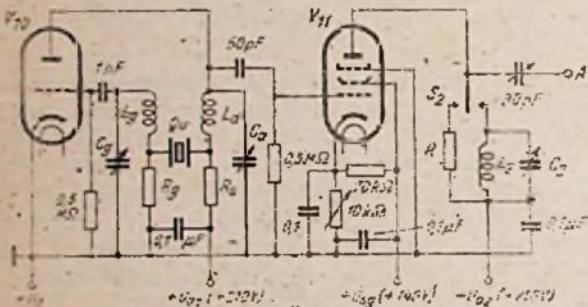
Abb. 8. Quarzoszillator nach Heegner (2. Art), mit Verstärkerstufe
