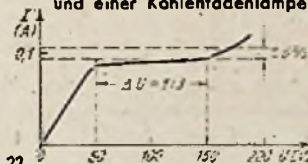
Abb. 22. Regelkurve eines Eisenwasserstoffwiderstandes
