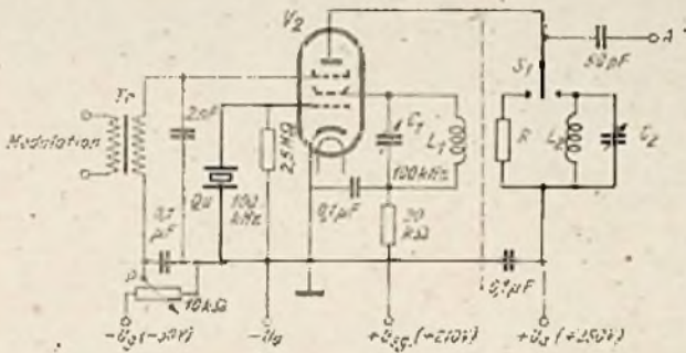
Abb. 3. Pierce-Schaltung mit einer Pentode
