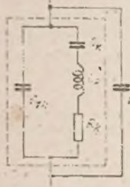
Abb. 1. Ersatzschaltbild eines Quarzes
