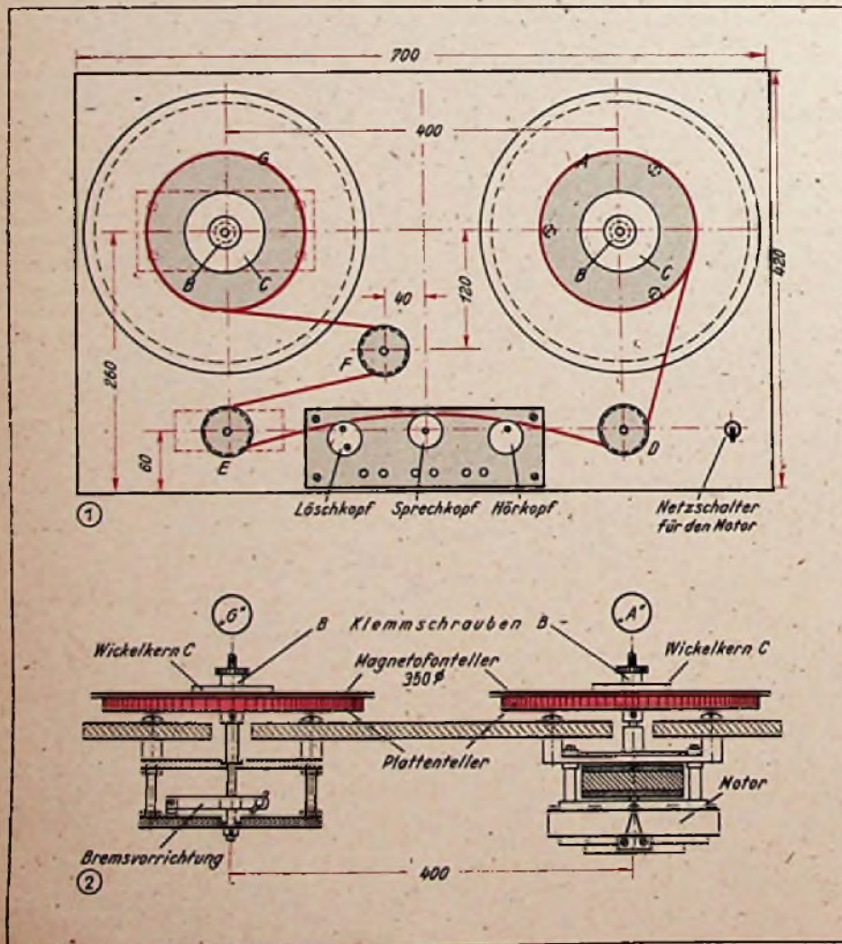
Abb. 2. Querschnitt der Montageplatte. Links: Vorrattstrommel mit Bremsvorrichtung Rechts: Antriebsteller mit Synchronmotor
