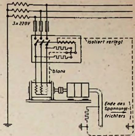
Abb. 3. Schutzgeschaltete Hauswasserpumpe
