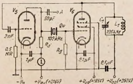
Abb. 5. Quarzoszillator nach Heegner (1. Art)
