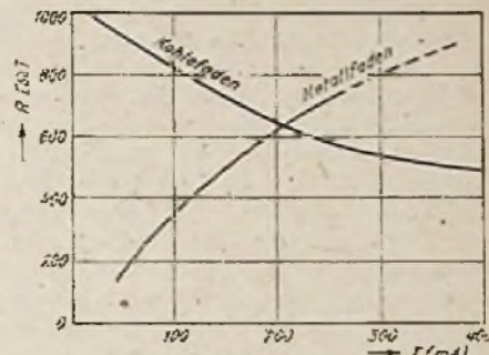
Abb. 21. Widerstandskurven einer Metallfaden- und einer Kohlefadenlampe
