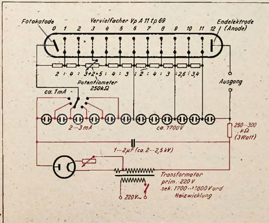
Abb. 3. Einfach stabilisiertes Netzgerät (Widerstandswerte 2 : 4 : 3 = 100 \text{ k}\Omega : 200 \text{ k}\Omega : 150 \text{ k}\Omega )
