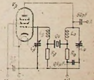
Abb. 7. Quarzoszillator nach Heegner (2. Art)
