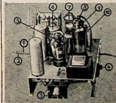
1. Abstimmung, 2. Bereichschalter, 3. Lautstärkeregl., 4. Netzspannungswähler, 5. AZ 11, 6. ECH 4, 7. ECH 4, 8. EBL 1, 9. und 10. ZF-Filter
