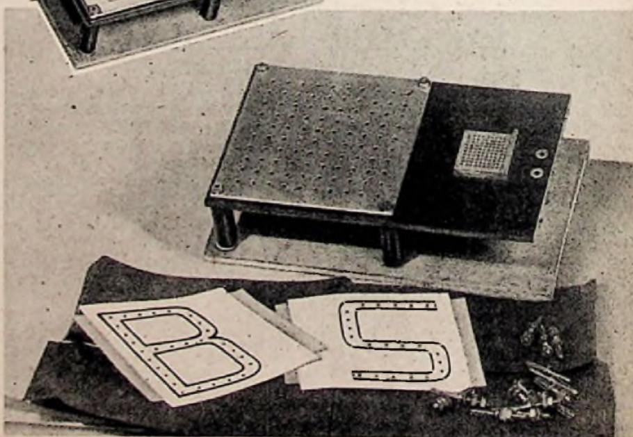
Abb. 3. Tasttableau mit Kontaktplatte
