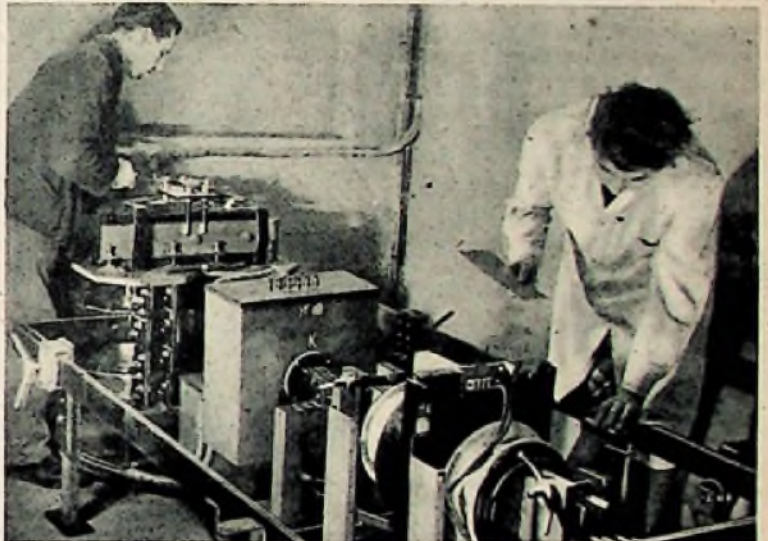
Fertigungskontrolle. Vorbereitungen zur Prüfung von Durchführungs-Meßstromwandlern
