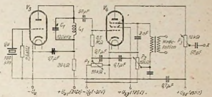
Abb. 4. Pierce-Quarzoszillator mit Verstärker-Verzerrerstufe
