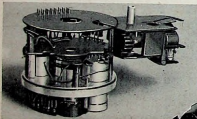
Links: Teilchassis. Bildkippgerät und Ablenkjoch sind seitlich herausgezogen
