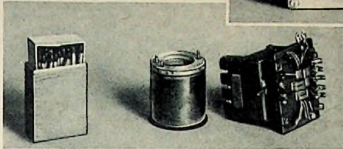
Kipptransformator für Zeilenablenkung und Ablenkloch für die Bildablenkung (oben). Die Erregerspulen des Ablenkloches sind durch gemeinsame Schutzölle abgedeckt. Zwischen den Polschuhen befindet sich das Spulensystem zur Zeilenablenkung, wobei die Polschuhe gleichzeitig als Rückschluß für das Zeilenablenkfeld dienen
