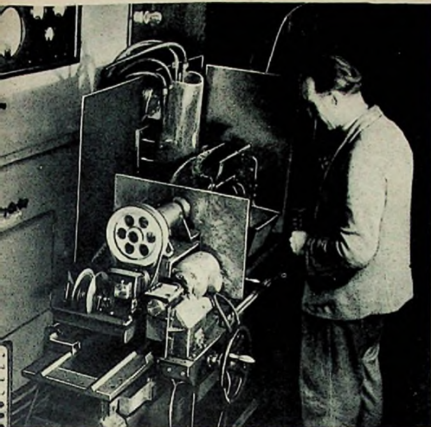
Generators. Eine Universal-Härtevorrichtung vor dem Sender. Lamplattenkühlern für die Röhren- und Werkstückkühlung
