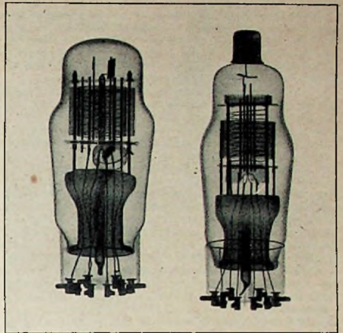
Röntgenaufnahme der UL 2 (links) und der UF 6 (rechts)
