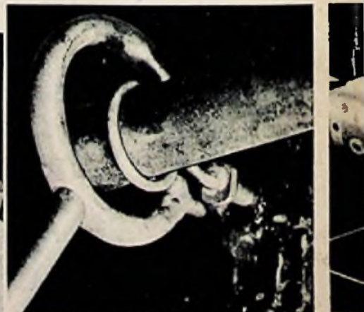
Vorshubhärtung einer Welle und eines Lagerzapfens. Besonders gut die Heizleiterschleife (kleiner Ring), durch die das Kühlwasser unter hohem Druck zum Absaugen
