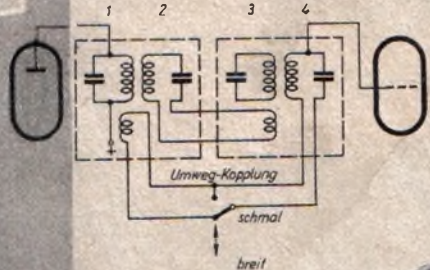
Das Vierkreis-Bandfilter mit Umweschaltung von Nord-Mende
