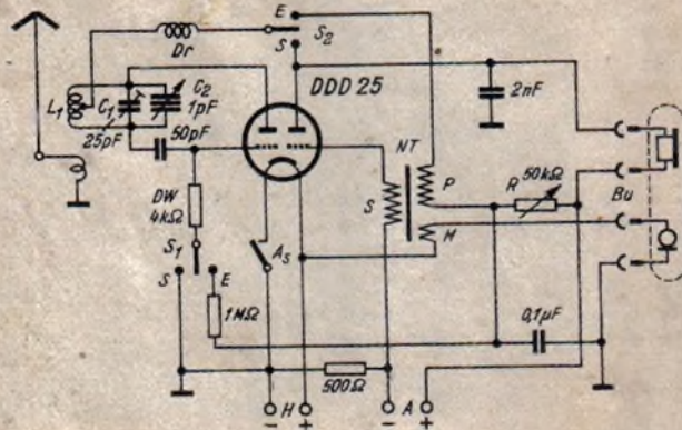
Abb. 2 Schaltbild eines einfachen, tragbaren UKW-Sender-Empfängers mit der Doppeltriode DDD 25 für Batteriebetrieb. L 1 = 3 Wdg. 1,5 Cu, 10 mm Ø, 10 mm lang; L 2 = 1 Wdg., 1 Cu, 10 mm Ø. Dr = 1 W Widerstand, vollgewickelt; mit 0,2 CuL. NT = M 42 15. P = 4000 Wdg., 0,1 CuL. S = 12000 Wdg., 0,05 CuL. M = 400 Wdg., 0,25 CuL
