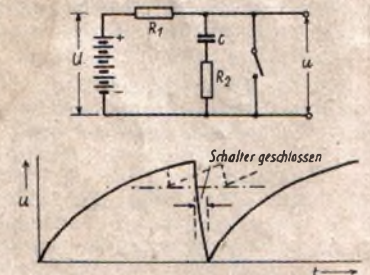
Abb. 4. Erzeugung einer Sägezahnspannung durch periodisches Aufladen eines Kondensators C über einen Widerstand R_1 und Entladen über R_2 < R_1 durch Kurzschließen mittels eines Schalters. Die gestrichelte Sägezahnkurve verläuft in einem als geradlinig anzunehmenden Bereich der beiden Exponentialkurven für Aufladung und Entladung
