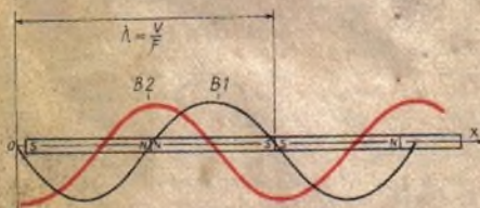
Abb. 3. Magnetische Felder längs des Tonträgers (Feld B1) und an seiner Oberfläche (Feld B2)
