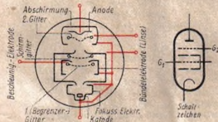
Abb. 1. Aufbau der FM-Demodulorröhre 6 BN 6
