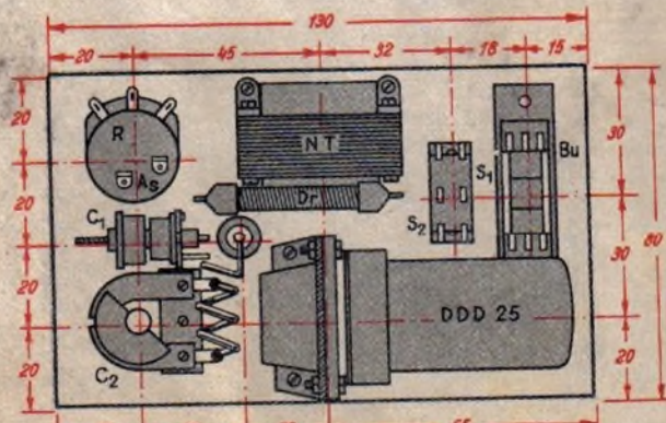
Abb. 3 Aufrißplan für das Einröhren-Radio-Telefon
