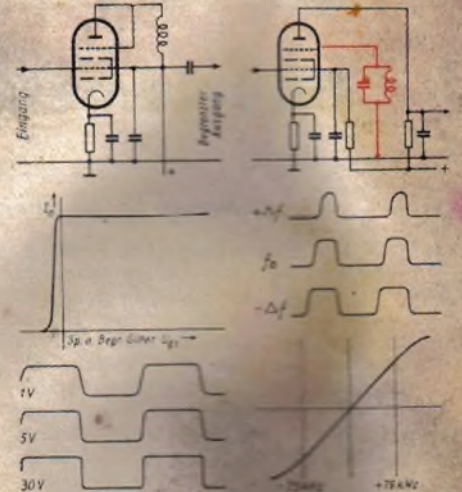
Abb. 3. Die Begrenzerwirkung der 6 BN 6 entsteht durch eine sehr steile Kennlinie. Oben: Grundsätzliche Begrenzerschaltung; Mitte: Dozugenhöriger Anodenstromverlauf; Unten: Rechteckwellen, entstanden durch Begrenzung einer Sinusschwingung verschiedener Spannungshöhe
