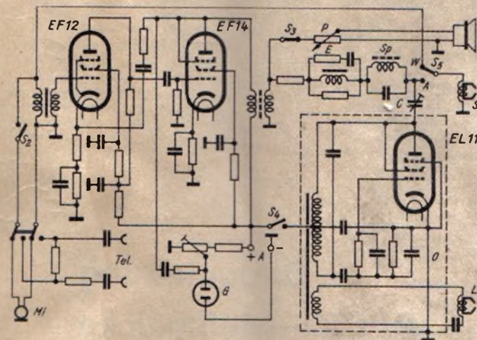
Abb. 6. Schaltung des Lorenz-Stahltongerätes LDG 1
