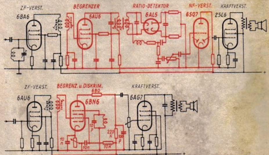
Abb. 5. FM-Demodulationsstufe üblicher Art (oben); und gleichwertige, mittels Begrenzer- und Diskriminatorröhre vereinfachte Stufe (unten). Die geübten Schaltungen stammen nicht aus gewöhnlichen UKW-FM-Rundfunkempfängern, sondern aus amerikanischen Fernsehgeräten, bei denen hinter dem Bildgleichrichter eine tontragende Schwebefrequenz entnommen ist (Zwischenfrequenzträger-Verfahren). Diese frequenzmodulierte Schwingung enthält zugleich eine starke Amplitudenmodulation. Die als ZF-Verstärker bezeichnete Stufe ist daher eigentlich ein Geradeausverstärker und dient zur Vorverstärkung des entnommenen Tonfrequenzbandes von 4,5 MHz Mittelfrequenz
