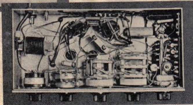
Chassis und Untersicht der Meßbrücke
