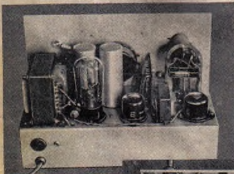
Chassis und Untersicht der Meßbrücke
