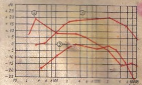
Abb. 8. Frequenzkurven: 1 Lorenz-Stahltongerät LDG 1, 2 Wire-Way-Gerät, 3 Tantoster CS 1
