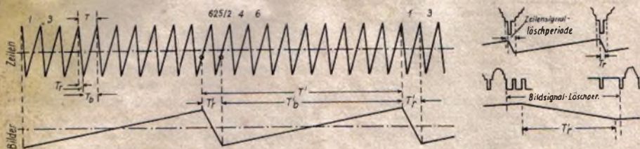
Abb. 2. Verlauf der Strahlableitungskräfte in einer Bildröhre, oben für die Horizontal-, unten für die Vertikalbewegung. Der Übersichtlichkeit halber ist nur eine geringe Zahl von Zeilen angenommen, so daß der Bildrücklauf während einer einzigen Zeilenhin- und -rückbewegung zu erfolgen scheint; in Wirklichkeit kommen auf den Bildrücklauf zwischen den beiden Halbbildern etwa 10 ... 20 Zeilen. Die Darstellung rechts zeigt, wie Beginn und Ende der Hin- und Rückbewegung des Elektronenstrahles innerhalb der Signallöscherperioden liegen. T_r = Zeilenrückschlagdauer, T_b = sichtbare Zeilendauer, T_r' und T_b' sind die entsprechenden Zeiten für die senkrechte Strahlbewegung
