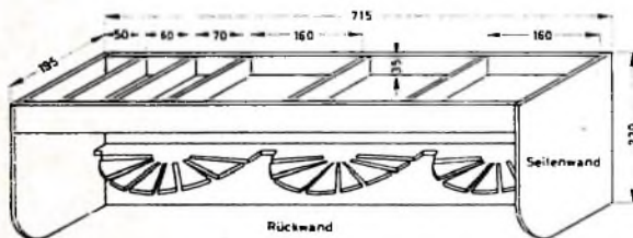
Konstruktionskizze und Abmessungen des Kabelrechens
