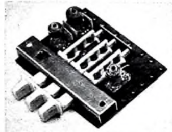
Drucktastenaggregat „Flat“ in sehr flacher Bauweise von Orega mit leicht zugänglichen Kontaktsätzen
