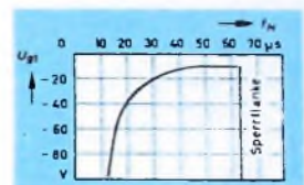
Bild 5. Schaltung der Horizontal-Endstufe: Steilheit der Sperrflanke \leq 50 V/µs, Sperrbreite > 22\% bei -100 V, Höhe \leq 110 V
