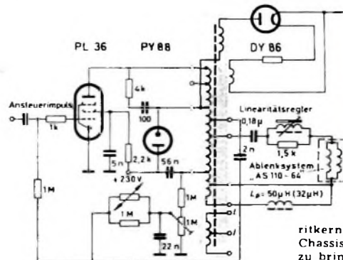
Bild 5. Schaltung der Horizontal-Endstufe: Steilheit der Sperrflanke \leq 50 V/µs, Sperrbreite > 22\% bei -100 V, Höhe \leq 110 V
