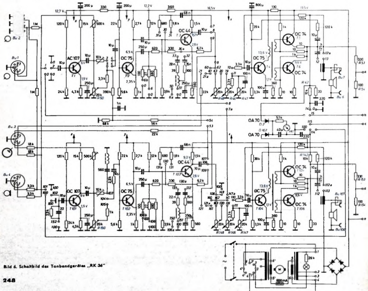
Schaltplan des „RK 36“
