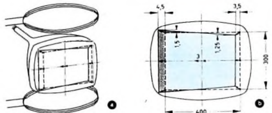
Bild 2 (oben). Einfache Anordnung zur Messung des Erdfeldinflusses (a); durch das Erdfeld hervorgerufene Verzeichnung (b)
