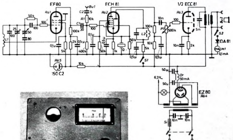
Bild 5 Schaltung des Frequenzmessers
