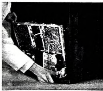
Bild 3. Programm-Wählautomatik mit Stationsdrucktasten; die Spindeln für die einmalige Grundeinstellung der VHF- und UHF-Sender sind in die Tasten eingelassen und durch einen abnehmbaren Schieber verdeckt
