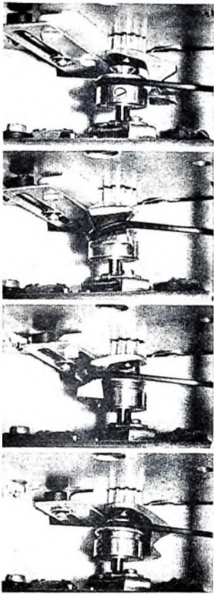
Bild 3. Umschalten der Bandgeschwindigkeit; die durch Tastendruck bewegte Zahnstange dreht das mit einem Ritzel verbundene Kurvenstück, die schräge Nut ertast den Antriebsriemen, der anfangs auf dem großen Durchmesser der Riemenscheibe liegt (9,5 cm/s), und führt ihn schräg nach oben. Bei der weiteren Drehung des Kurvenstücks gleitet der Riemen auf den kleinen Scheibendurchmesser (4,75 cm/s)
