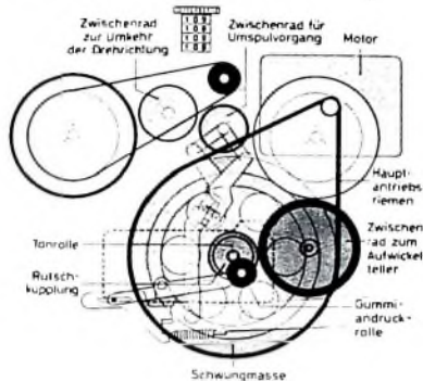
Bild 4. Schematische Darstellung des Antriebs
