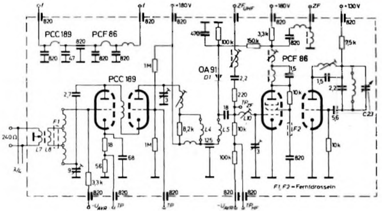
Bild 2 Gesamtschaltbild der VHF-Kanalwähler „NT 1009“ und „NT 1010“
