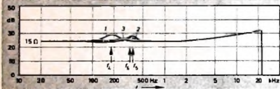
Bild 5. Impedanzverlauf des Mittelton-Lautsprechers (aus hochohmiger Quelle gespeist): 1 Gehäuse offen, 2 Gehäuse geschlossen und leer, 3 Gehäuse geschlossen und 60% mit Steinwolle gefüllt
