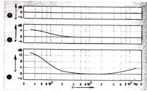
Bild 5. Einfluß der gehörrihtigen Lautstärkeerregung auf den Frequenzgang; a) Lautstärkeerregler voll aufgeregt, b) Schleifer am oberen Abgriff, c) Schleifer am unteren Abgriff
