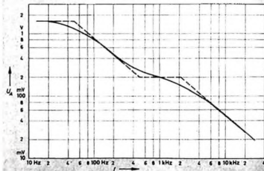
Bild 4. Frequenzgang der Schneidkennlinienentzerrung
