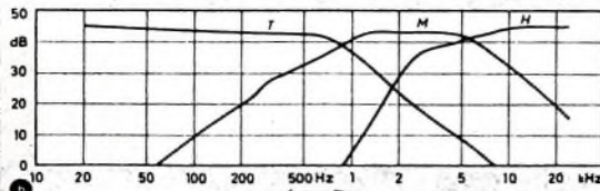
Bild 9b. Spannungsverlauf an den über das Netzwerk gespeisten Einzellautesprechern (T Tieftön-, M Mitteltön-, H Hochtön-Lautsprecher)
