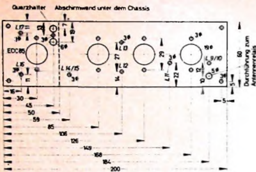
Bild 12. Abmessungen des Konverterchassis
