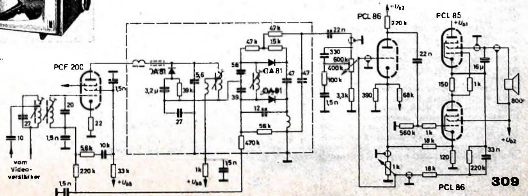
Bild 6. Schaltung des Ton-teils der „Fernseh-Philetta“
