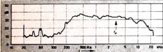
Bild 6. Frequenzgang des eingebauten Mittelton-Lautsprechers, gemessen mit gewobbeltem Sinus in einem Raum von 48 m 3 Volumen
