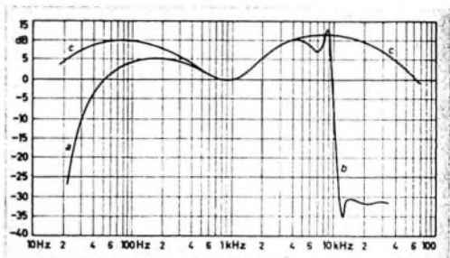
Bild 9. Frequenzgänge der gehörlichen Lautstärkeregelung
