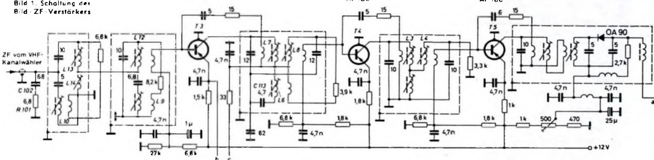
Bild 1. Schaltung des Bild-ZF-Verstärkers
