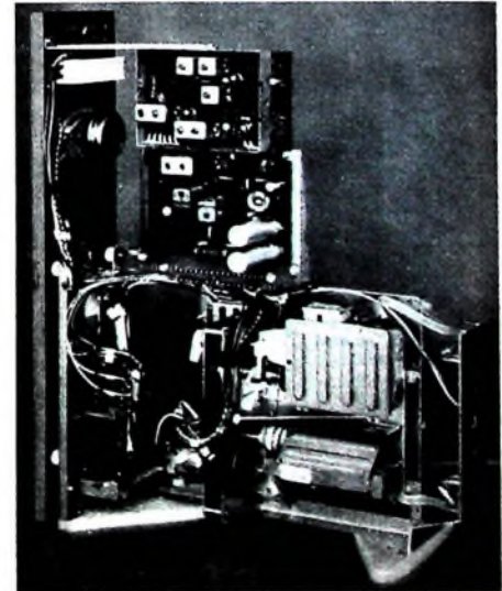
Bild 6. HF-Baustein mit dem neuen UHF-Tuner (unten rechts) für ein Fernsehgerät mit elektronisch gesteuerter Motor-Suchlaufautomatik
