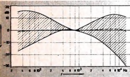
Bild 4. Regelbereich der Höhen- und Tiefenregler
