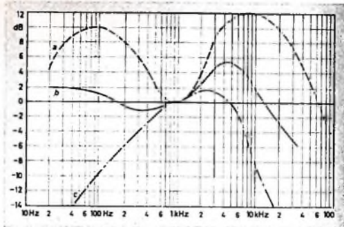
Bild 7. Frequenzgang des Entzerrers; a magnetischer Abtaster (IEC), b Kristallabtaster, Mikrolan-Rundfunk, Magneton
