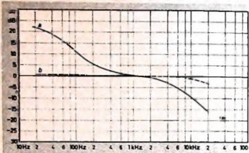
Bild 7. Frequenzgang des Entzerrers; a magnetischer Abtaster (IEC), b Kristallabtaster, Mikrolan-Rundfunk, Magneton
