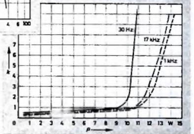
Bild 6 (unten). Klirrfaktor k in Abhängigkeit von der Ausgangsleistung für verschiedene Frequenzen
