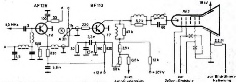
Bild 2. Videoverstärker des „Wegavision 3000“
