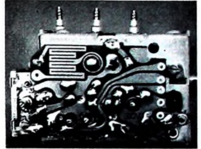
Bild 4. Innenansicht des neuen Nordmende-UHF-Tuners; alle Hochfrequenz führenden Bauteile befinden sich innerhalb des Tunergehäuses
