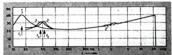
Bild 3. Impedanzverlauf des Tiefton-Lautsprechers (aus hochohmiger Quelle gespeist); 1 Gehäuse offen, 2 Gehäuse geschlossen und leer, 3 Gehäuse geschlossen und 60% mit Steinwolle gefüllt
