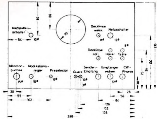
Bild 14. Anordnung der Bedienelemente auf der Frontplatte
