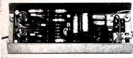
Bild 2. Innenansicht des „TVV 43“
