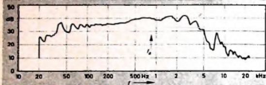
Bild 4. Frequenzgang des eingebauten Tiefton-Lautsprechers, gemessen mit gewobbeltem Sinus in einem Raum von 48 m 3 Volumen (vgl. 4.1.3.)
