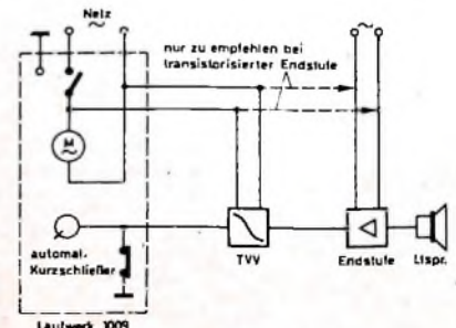
Bild 5. Gemeinsame Anschaltung von Entzerrervorverstärker und Lautwerk an das Netz
