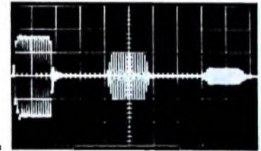
Von links nach rechts: Direkt übertragener Impuls, erste Reflexion, zweite Reflexion; Meßfrequenz 2,95 kHz
