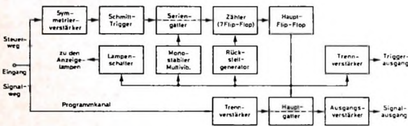
Bild 4. Blockschaltbild des Tonburst-Generators „1396-A“
