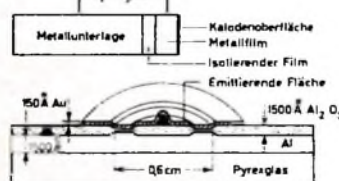
Bild 5. Konstruktionsprinzip der Tunnelkatode (nach J. Appl. Phys. Bd. 32 (1961) Nr. 4)
