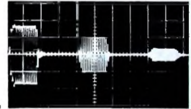
Die gleichen Impulsformen bei einer auf 3 kHz erhöhten Frequenz
