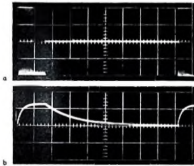
Bild 6. Untersuchung von Meßgeräten mit Gleichrichternetzwerken: a) Tonburst vor einem Gleichrichternetzwerk großer Einschwingzeitkonstante (32 Perioden je Impuls, 10 kHz); b) nach dem Passieren des Gleichrichters
