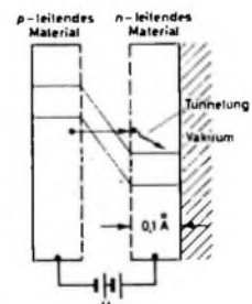
Bild 6. pn-Schichtkatode (nach Phys. Rev. Letters Bd 7 (1961) Nr. 3)
