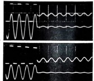
Bild 5. Belastungskennlinien eines übersteuerten Verstärkers. Die durchgehende untere Linie zeigt die Eingangsspannung, die obere abgekoppelte Sinuslinie die Ausgangsspannung (Meßfrequenz 1 kHz, 4 Perioden): a) der Verstärker zeigt bei einer vierfach überhöhten Eingangsspannung fast keinen Spannungsabfall während der Überlastungszeit; b) die Ausgangsspannung des Verstärkers sinkt bei sechsfacher Übersteuerung (anderer Maßstab) ab
