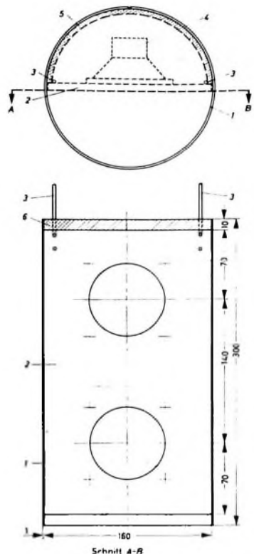
Bild 2. Maßskizze für den Stereo-Seitenlautsprecher: 1 Streckmetallgehäuse, 2 Schallwand, 3 Zuleitungen, 4 Lautsprechersystem, 5 Filzdichtung (250 mm x 280 mm x 10 mm), 6 Filzdeckel (160 mm ø x 10 mm)
