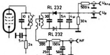
Bild 21. Ratiodetektor im UKW-Vorsatzgerät „S/III“ (Saba)
