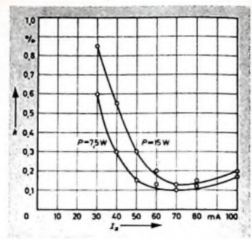
Bild 5. Klirrfaktor k bei 1 kHz als Funktion des Anodenruhestroms I_a im Endröhrensystem
