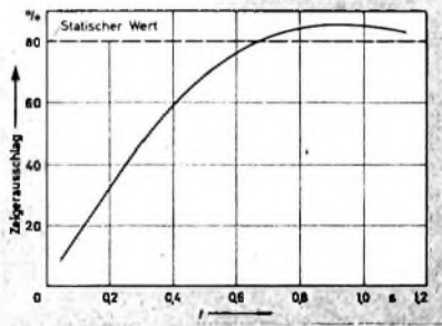
Dauerionmessung bei einer Frequenz von 2,95 kHz
