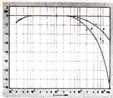
Bild 4. Frequenzgang des Verstärkers a) volle Wicklung unbelastet oder belastet, Anzapfung unbelastet; b) Anzapfung belastet, Übertrager 1x verschachtelt
