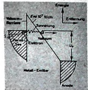
Bild 3. Veranschaulichte Darstellung des Feldemissionsvorgangs; starke elektrische Felder veranlassen die Elektronen zu ihrem Austritt aus der Kaltkatode (nach AIEE Trans. l v. 28. Jan. 1962)
