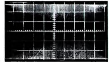
Dauerionmessung bei 3 kHz; infolge Ausbildung stehender Wellen ist die Frequenzcharakteristik des Prüflings nicht erkennbar
