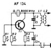
Bild 1. Schaltbild des Eichgenerators
