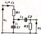
Bild 4. Grundschaltung des frequenzabhängigen Zweiges der Brücke (Sulzar-Vierpol)
