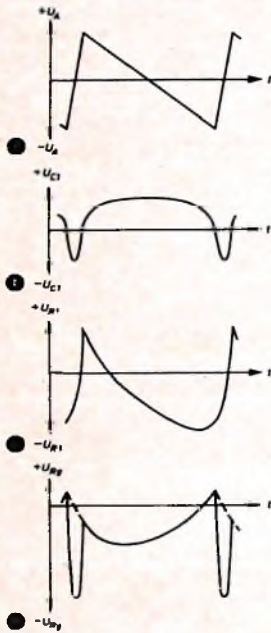
Bild 90. Parabellörmige Vorverzerrung der Steuerspannung der Bild-Endröhre: a) Anodenspannung U_a (ohne Rücklaufspitze), b) Spannung U_{c1} an C_{81} , c) Spannung U_{g1} an R_{81} ( U_{g1} = U_a - U_{c1} ), d) Steuerspannung der Bild-Endröhre U_{g2} = U_{g1} - U_{g2} = -U_a + (U_a - U_{c1})
