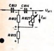
Bild 94. Entstehung der Steuerspannung U_{S11}
