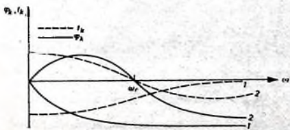
◀ Bild 8. Frequenzabhängigkeit von |R_k| : 1 Widerstand mit Kondensator überbrückt, 2 Netzwerk nach Bild 10
