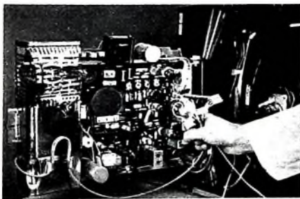
Fernsehempfänger-Chassis „1823“ von Kuba-Imperial
