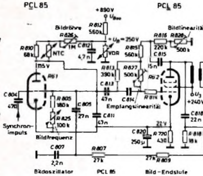
Bild 91. Gesamtschaltung der Bildablenkung mit abgewandeltem Sperrschwinger
