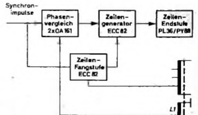
Bild 1. Blockschaltbild des Zeilenteils
