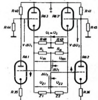
Bild 3. Funktionsschaltung des Oszillators mit Darstellung der Spannungsverhältnisse
