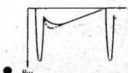
Bild 94. Entstehung der Steuerspannung U_{S11}
