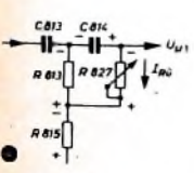
Bild 93. Prinzipschaltung der Korrektur der Anfangslinearität: a) Rücklauf, b) Hinlauf
