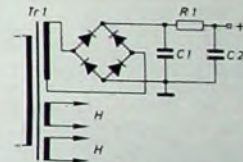
Bild 114. Einfacher Niederspannungs-Netzteil
