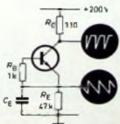
Bild 2. Der Lawinenzustand erzeugt kurze Impulse und Sägezähne
