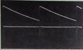
Bild 6. Spannungsverläufe an den Sägezahn- und Impulsausgängen eines Frequenzteilers
