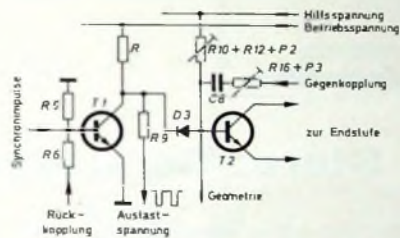
Bild 6 Schaltung zur Gewinnung der Austastspannung
