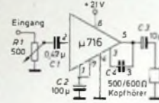
Bild 5. Kanalverstärker für Fernsprechsysteme
