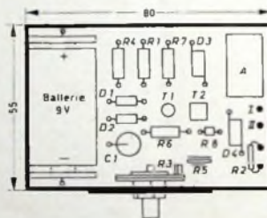
Bild 2. Einzelteilanordnung auf der Montageplatte
