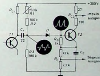
Bild 5. Von einer vorhergehenden Stufe synchronisierter Frequenzteiler
