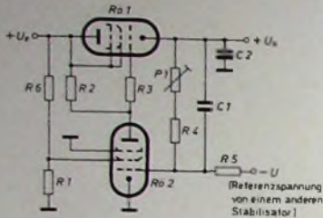
Bild 115. Röhrenstabilisator für niedrige Spannungen
