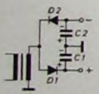
Bild 116 Ein einfacher Verdoppler
