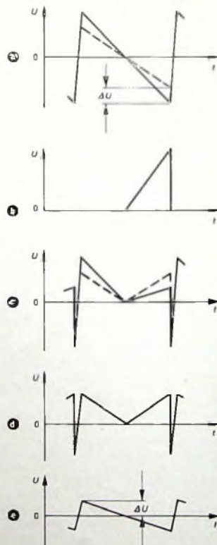
Bild 5. Spannungsverläufe zur Gesamtgeometrie-Einstellung: a) Spannungsabfall an 0,75 \cdot R 20 durch den Ablenkstromverlauf, b) Spannungsabfall an R 20 durch den Emitterstromverlauf von T 4, c) resultierender Spannungsverlauf am Emitter von T 4, der sich in den ursprünglichen V-Spannungsverlauf (d) und die mitlaufende Ladespannung (e) zerlegen läßt
