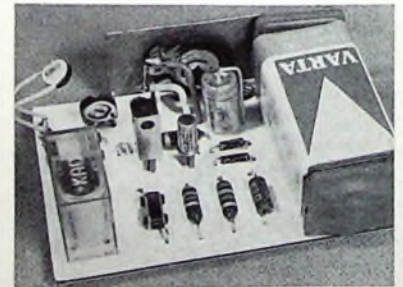
Bild 4. Rückansicht des Thermo-schalters
