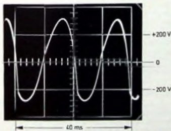
Bild 13. Oszillogramm der Ausgangsspannung
