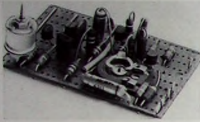
Bild 4. Oszillator-Baugruppe
