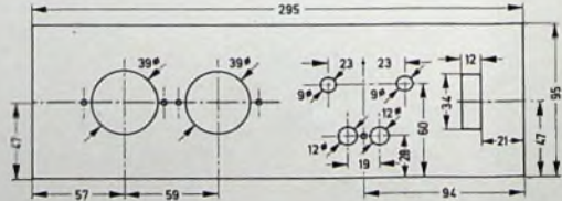
Bild 5. Einzelteileanordnung
