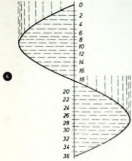
Bild 133. Lissajous-Figur, Frequenzverhältnis 3:1, \varphi = 90^\circ
