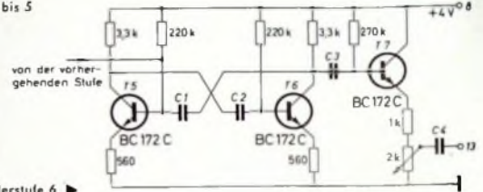
Bild 6. Teilerstufe 6
