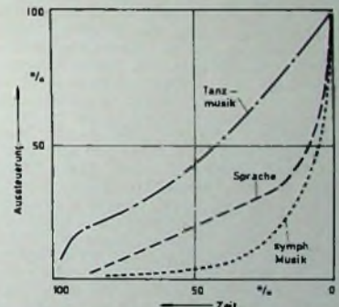
Bild 2. Amplitudenverteilung von Sprache und Musik (nach van den Valentyn); Integralmittelwerte: Tanzmusik 49%, Sprache 22%, symphonische Musik 12%
