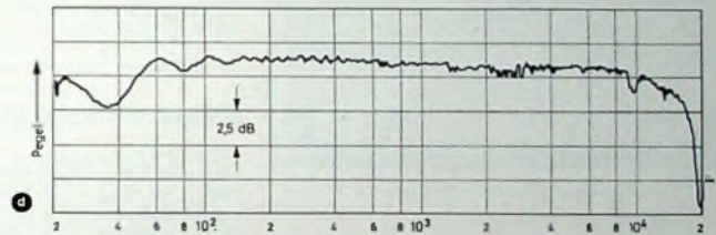
Bild 4 (rechts). Frequenzgänge des „PRO 12“ a) Wiedergabefrequenzgang eines Kanals bei 9,5 cm/s, b) Wiedergabefrequenzgang eines Kanals bei 19 cm/s, c) Überalles-Frequenzgang eines Kanals bei 9,5 cm/s, d) Überalles-Frequenzgang eines Kanals bei 19 cm/s
