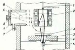
Bild 3. Schematische Darstellung der Objektschleuse mit Ablenssystem: A Arbeitsstellung der Objektpatrone, B Schließstellung der Objektpatrone, C Elektronenstrahl, D Ablenssystem, E Objektisch, F Objekt, G Schließventil, H automatisches Belüftungssystem, I äußere Schleusenöffnung
