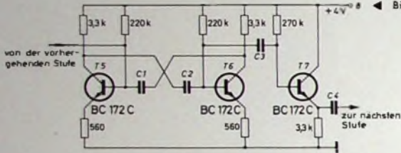
Bild 4. Oszillator-Baugruppe
