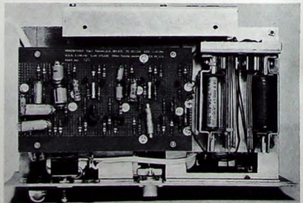
Bild 10. Frequenzteiler-Baugruppe
