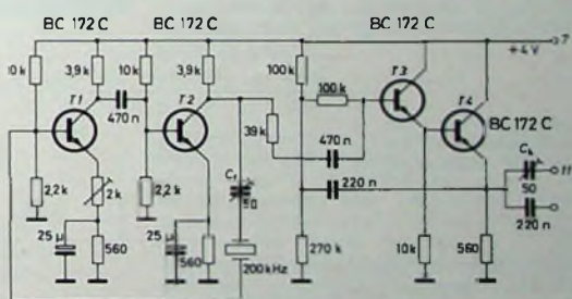
Bild 2. Schaltbild Quarzoszillator
