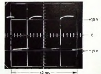
Bild 9. 50-Hz-Rechteckspannung am Ausgang der Teilerkette
