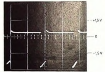
Bild 8. Schirmbild an der Basis der Trennstufe T7
