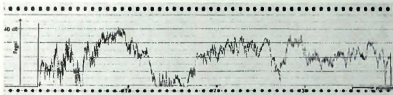
Bild 1. Zeitlicher Pegelverlauf am Beispiel symphonischer Musik (Hiller-Variationen für großes Orchester von Max Reger: Anfang bis kurz vor dem Ende der zweiten Variation)
