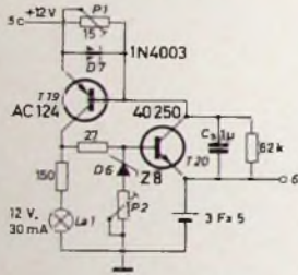
Bild 20. Ladeschaltung
