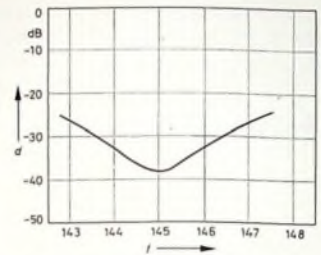
Bild 8 Dämpfungsverlauf einer Stichleitung für die Frequenz 145 MHz
