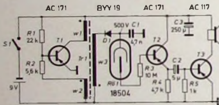
Bild 1. Schaltung des Gerätes
