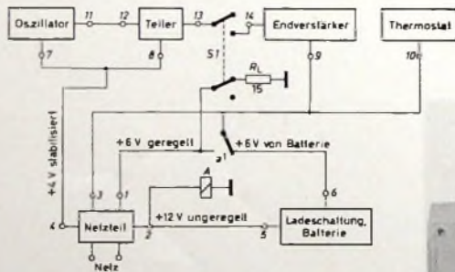
Bild 22. Zusammenschaltung der Baugruppen
