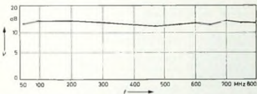
Bild 1. Verstärkung V des Allbereichs-Verstärkers „TK 60“ von Astra in Abhängigkeit von der Frequenz f
