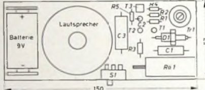
Bild 2. Anordnung der Einzelteile auf der Montageplatte
