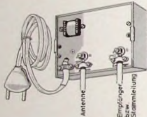
Bild 5 Allbereichs-Verstärker „TK 60“ (Astro)
