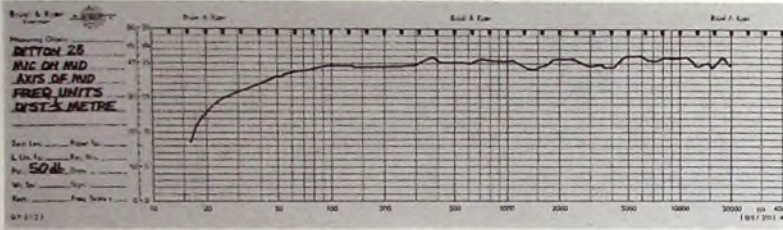
Frequenzgang der Hi-Fi-Lautsprecherbox „Ditton 25“ von Celestion
