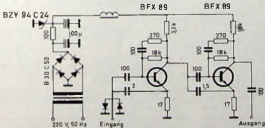
Bild 2. Schaltung des Allbereichs-Verstärkers „TK 60“ (Astira)
