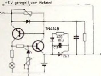
Bild 21. Ladeschaltung mit kontaktloser Umschaltung
