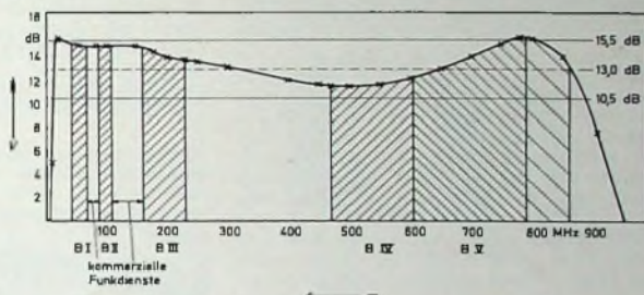
Bild 4. Verstärkung V des Allbereichs-Verstärkers „FVM 10“ (R. Bosch Elektronik)
