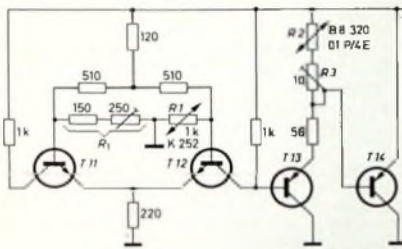
Bild 14. Schaltung des Thermostaten ( T11 : T12: BC 172 C; T13 : AC 124; T14 : AD 130)
