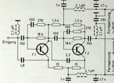
Bild 3. Schaltung des Allbereichs-Verstärkers „FVM 10“
