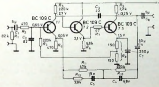
Bild 1. Schaltung des Phonoerzerrerverstärkers
