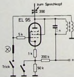
Bild 1. Schaltung des Löschen-generators in einem Tonbandgerät
