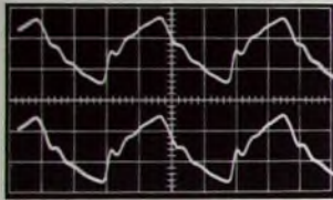
Bild 4 Ausgangsspannungen eines Stereo-Abtasters mit Entzerrer-Vorverstärker bei Seitenschritt
