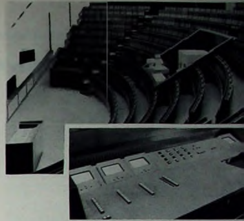
Bild 2. Hörsaal mit Eidophor-Projektionskanzel und dem links unten erkennbaren Regiepult. Der Ausschnitt zeigt das Regiepult mit Bedienungsorganen, Monitoren und der Glaspalte (rechts) der Fernschreibeinrichtung mit dem dazugehörigen Monitor
