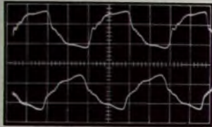
Bild 3 Ausgangsspannungen eines verpolt angeschlossenen Stereo-Abtasters (Seitenschritt, mit Entzerrer-Vorverstärker)
