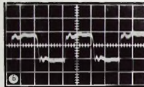
Bild 4 Ausgangsspannungen eines Stereo-Abtasters mit Entzerrer-Vorverstärker bei Seitenschritt
