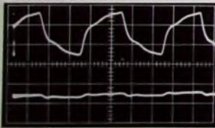
Bild 5 Oszillogramm der Spannung des rechten Kanals (oben) und der Übersprechspannung im linken Kanal (unten) bei Flankenschrittabtastung (mit Entzerrer-Vorverstärker)
