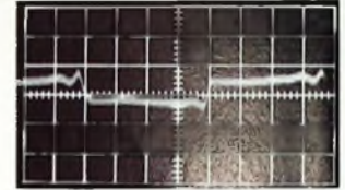
Bild 9 Ausgangsspannung des rechten Kanals bei 16\frac{2}{3} \text{ U/min} ( R_b = 39 \text{ kOhm} , Auflagekraft 2 p)
