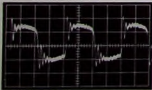
Bild 6 Ausgangsspannung des rechten Kanals bei R_b \approx 1 \text{ MOhm} (ohne Entzerrer-Vorverstärker, Auflagekraft 2 p)
