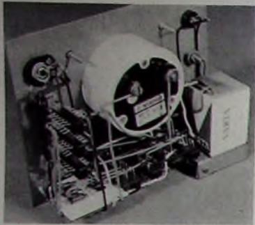
Bild 2. Blick auf die Verdrahtung des Prüfgerätes
