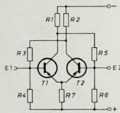
Bild 33. Grundschaltung eines Flip-Flop-Kreises
