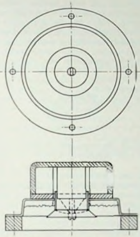
Bild 12 Hochtonlautsprecher in schematischer Darstellung (Maßstab 1:2)
