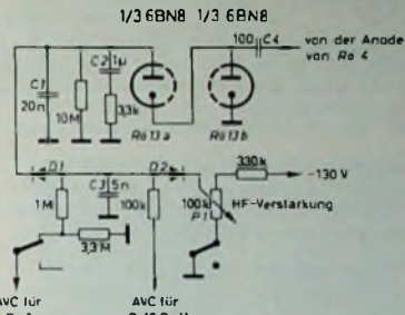
Bild 6. Schaltung der Regelspannungserzeugung im Empfangsteil
