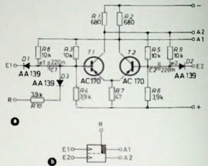
Bild 34. Vollständige Flip-Flop-Schaltung; a) konventionelle Darstellung, b) Flip-Flop-Symbol
