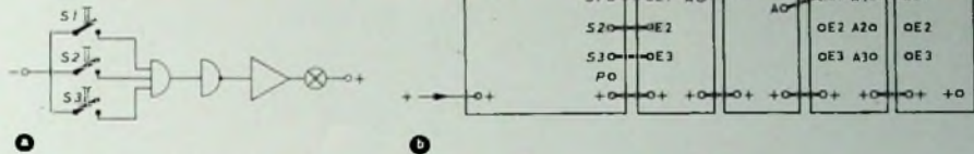
Bild 28 Versuch 6: a) Schaltung (symbolische Darstellung), b) Aufbau auf dem Rahmen
