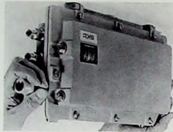
Bild 3. Ansicht eines Hauptstammleitungsverstärkers (SKL)
