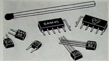
Si-Planar-Dioden der SAY- und SAM-Reihe in Plastikgehäusen
