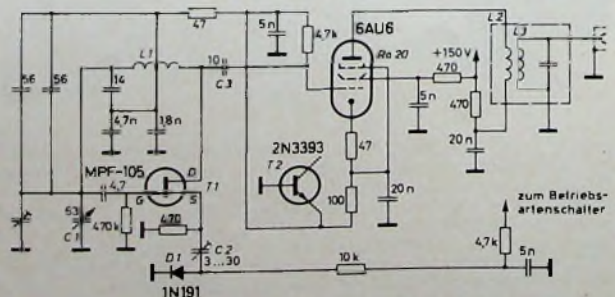
Bild 4. Schaltung des VFO mit VFO-Verstärker
