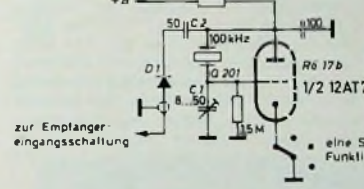
Bild 6. Schaltung der Regelspannungserzeugung im Empfangsteil
