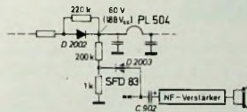
Bild 13 (oben). Kurzschluß-Warnschaltung in den Schwarz-Weiß-Fernsehempfängern von Metz
