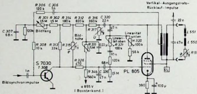
Bild 3. Schaltung der Vertikalablenkstufe der neuen Blaupunkt-Schwarz-Weiß-Fernsehempfänger
