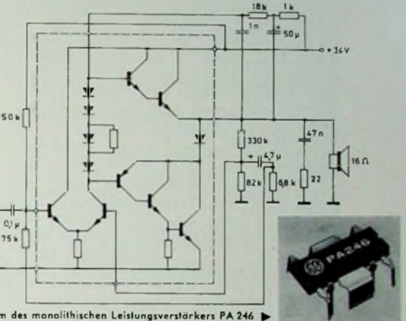
Bild 6. Bauform des monolithischen Leistungsverstärkers PA 246
