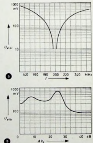
Bild 3. Kreuzmodulationseigenschaften der Schaltung nach Bild 2; a) zusätzliches Störsignal U_{Stör} für 1% Kreuzmodulation als Funktion der Frequenz, b) bei 1% Kreuzmodulation zulässige Störspannung als Funktion der Abregelung \Delta V_V der Leistungsverstärkung
