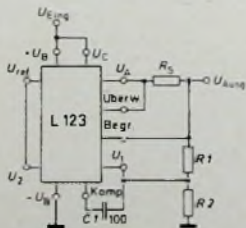
Bild 9. Grundschaltung eines Konstantspannungsreglers für 7 \dots 37 V mit der monolithischen Schaltung L 123 nach Bild 8 von SGS
