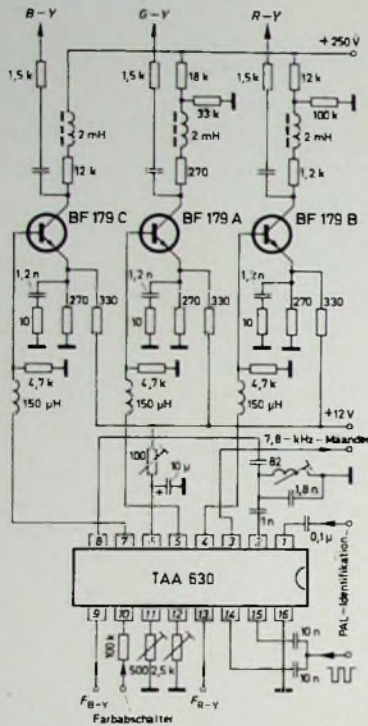
Bild 7. Schaltungsbeispiel für die Gewinnung der Farbdifferenzsignale mit Hilfe der integrierten Schaltung TAA 630 von Valvo
