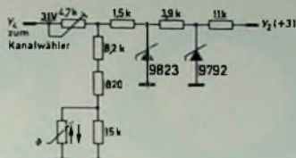
Bild 1. Alle Schaltung zur Gewinnung der stabilisierten Abstimmspannung
