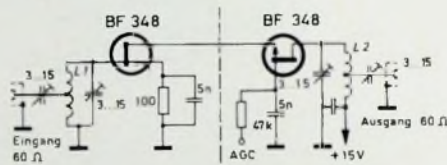
Bild 2. Kaskodeverstärker mit Feldeffekttransistoren für Frequenzen um 200 MHz
