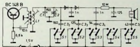
Bild 19. Schaltung des Ultraschallgebers nach Bild 18
