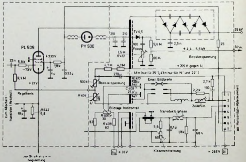
Bild 4. Schaltung der Horizontalablenkstufe mit Spannungsverdreifacher der neuen Blaupunkt-Farbfernsehempfänger
