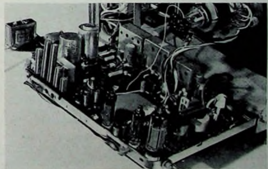
Bild 8 Herausgeklapptes Einplatinenchassis der neuen Schwarz-Weiß-Fernseheräte von Grundig
