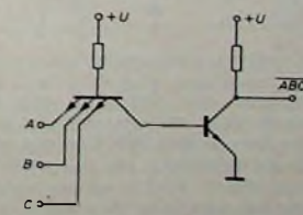
Bild 9. NAND-Gatter in Transistor-Transistor-Technik TTL
