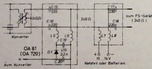
Bild 8. Schaltung der Gleichstromweichen für 240-Ohm-Leitung
