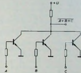
Bild 6. NOR-Gatter in Alltransistor-Technik RTL
