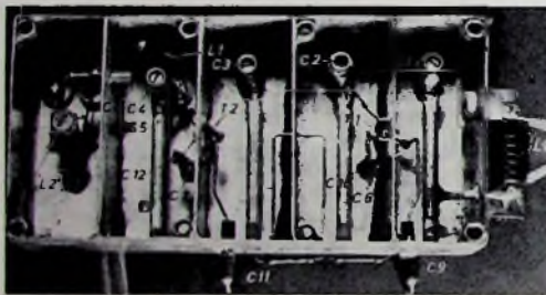
Bild 6. Innenansicht des Konverters
