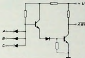
Bild 3. NAND-Gatter in DTL-Technik
