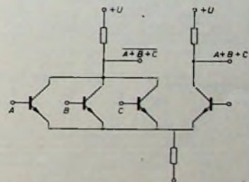
Bild 8. NOR-Gatter in Stromgesteuerter Logik CML
