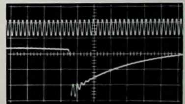
Bild 2. Durch eine 25-MHz-Schwingung (oben) wurde der unten dargestellte Triggerimpuls synchronisiert
