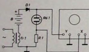
Bild 107. Schaltung zur Untersuchung von Referenzröhren
