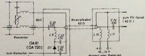
Bild 9. Schaltung der Gleichstromweichen für 60-Ohm-Koaxialkabel
