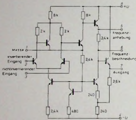
Bild 20. Operationsverstärker mit großer Bandbreite (MIC 712)
