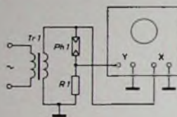
Bild 106. Schaltung zur Kennlinienaufnahme von Photowiderständen
