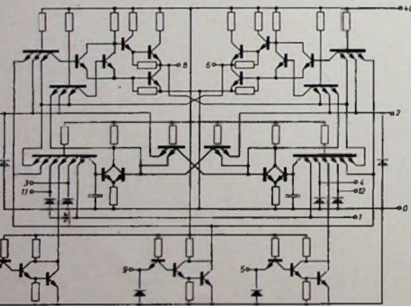
Bild 12 (oben). Bistabiler Flip-Flop MIC 9001
