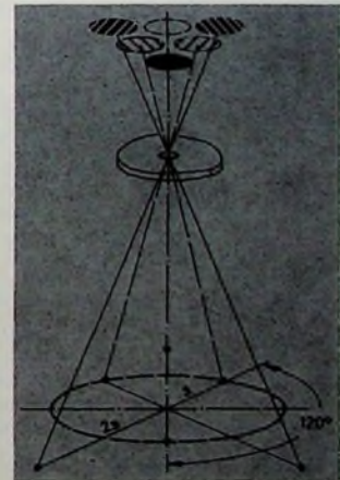
Bild 7. Bei indirekter Belichtung treffen die Lichtstrahlen Farbpunkte der benachbarten Farbtripel
