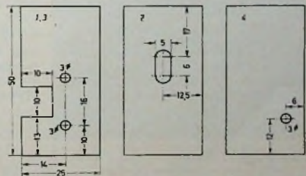
Bild 2. Maßskizze des Convertergehäuses
