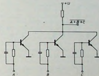
Bild 7. NOR-Gatter in Widerstands-Kondensator-Transistor-Technik RCTL
