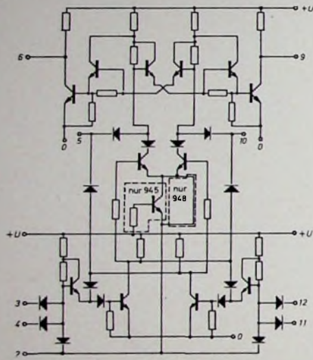
Bild 10. Bistabiler Flip-Flop MIC 945/MIC 948
