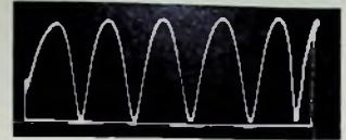
Bild 115. Sprungwellenverlauf längs einer Leitung bei Verwendung des Wobbelverfahrens [2]
