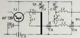
Bild 4. Ausgangsschaltung für 60 Ohm
