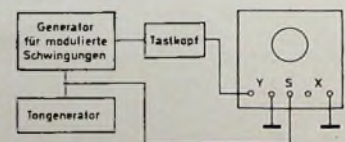
Bild 109. Schaltung zur Untersuchung modulierter Schwingungen
