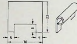
Bild 5. Maßskizze des Blechkerns der Eingangsumwegleitung L 12
