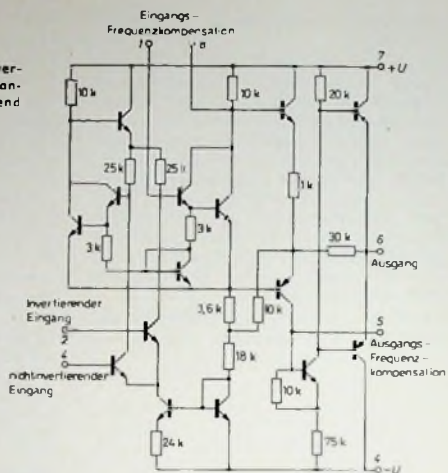
Bild 19. Operationsverstärker mit hoher Verstärkung (MIC 709)
