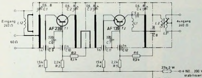
Bild 1. Schaltung des Converters mit 240-Ohm-Ausgang
