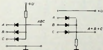
Bild 1. Positives UND-Gatter mit Dioden. Bild 2. Positives ODER-Gatter mit Dioden
