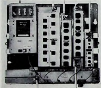
Bild 6. Gehäuse des Transistorverstärker-Baukastens von Hirschmann mit Netzgerät, Frequenzumsetzer und Verstärkereinsätzen
