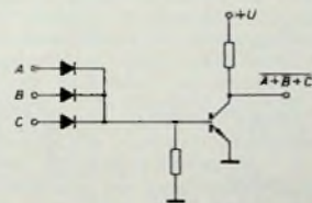
Bild 4. NOR-Gatter in DTL-Technik
