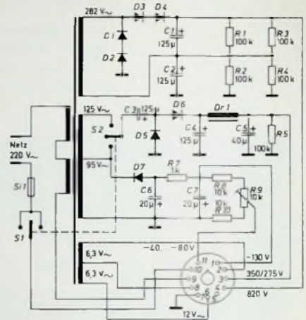
Bild 12 Schaltung des Stromversorgungsteils für den Transceiver
