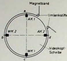
Bild 4. Videokopf-Scheibe des Halbbildspeichers
