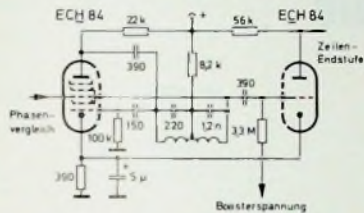
Bild 1. Teilschaltung des Zeilenoszillators eines Fernsehempfängers
