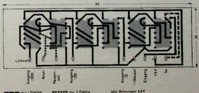
Bild 8 Leitungsführung für die Zeitteiler mit 3 Dekaden nach Bild 6 (Ansicht auf Leitungsseite); die gestrichelten Leitungen sind nur auf der zweiten Platine erforderlich, dafür entfällt dann dort der Toranschluß
