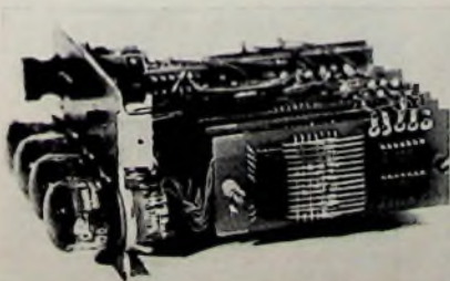
Bild 14. Leitungsführung auf einer Zähldekaden-Platte; Ansicht auf Leistungsseite
