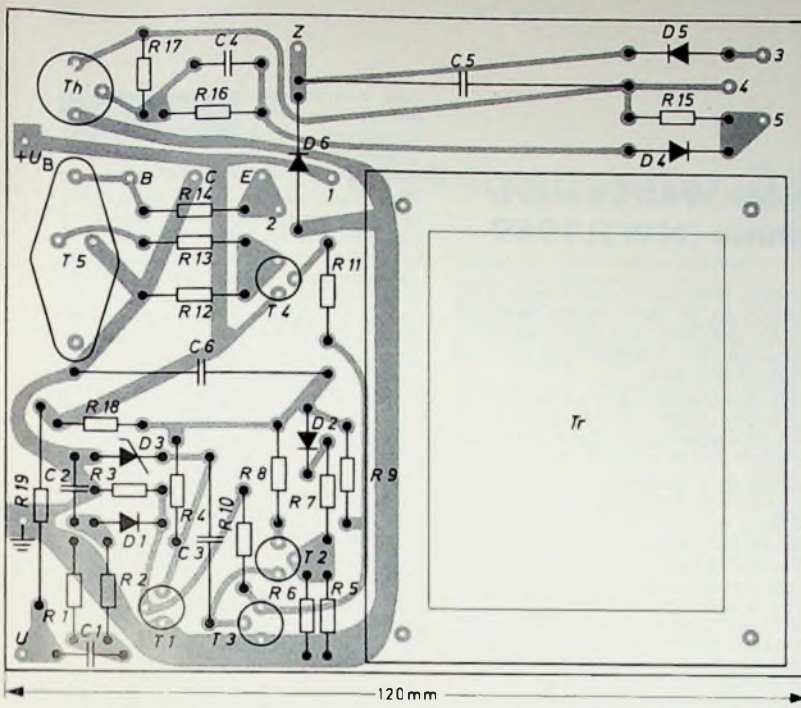
Bild 5. Platine, im Maßstab 1:1, zugleich Bestückungsplan; Ansicht von unten auf die Leiterbahnen
