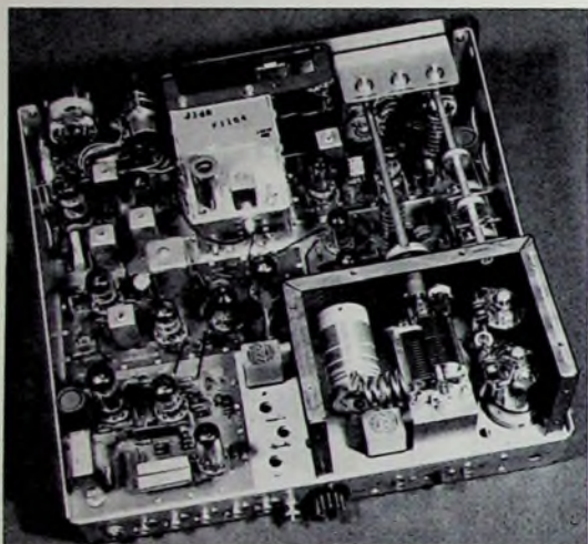
Bild 8 Blick in den Innenaufbau des 5SB/CW-Transceivers, 5B-101
