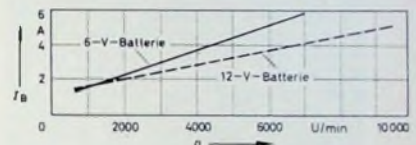
Bild 9. Effektivwert des aufgenommenen Stromes I_{\text{eff}} in Abhängigkeit von der Drehzahl n
