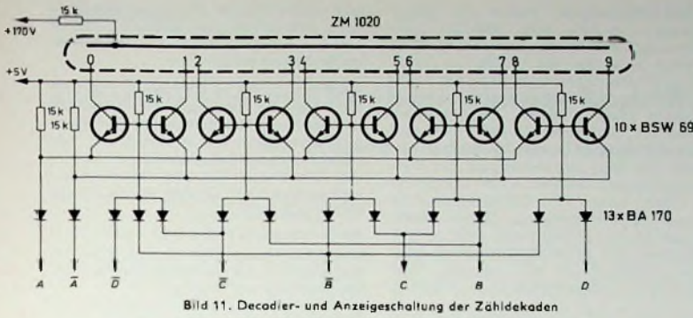
Bild 11. Decodier- und Anzeigeschaltung der Zähldekaden
