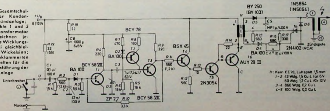
Bild 1. Prinzipschaltung des fremdgesteuerten Sperrwandlers zur Kondensatoraufladung
