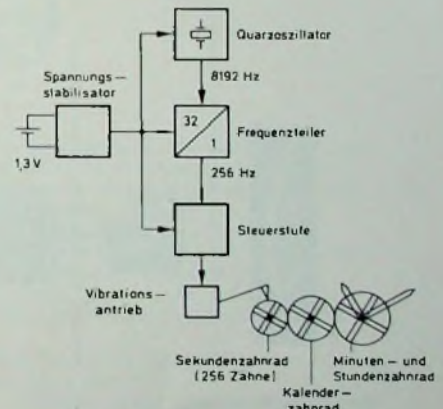
Bild 3. Blockbild der quartzgesteuerten elektronischen Armbanduhr
