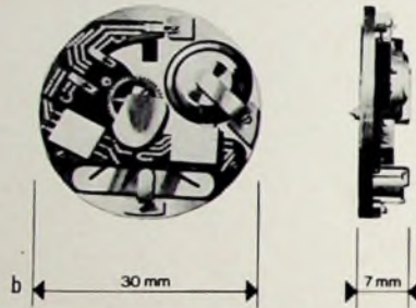
Bild 4 Elektronische Hochfrequenz-Armbanduhr im Maßstab 1:1 (a) und Ansicht des Werkes (b) ( Girard-Perregaux SA, La Chaux de Fonds )
