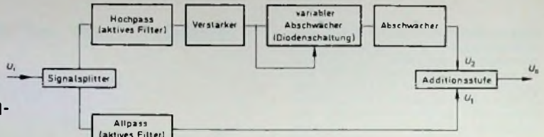
Bild 1: Blockschaltung des DNL-Rauschbegrenzers
