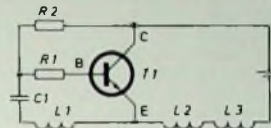
Bild 1. Schaltung einer Stimmgabeluhr (Unisonic „52“)
