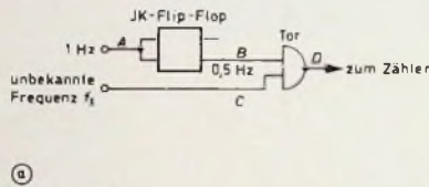
Bild 1 Prinzipschaltung der Frequenzmessung
