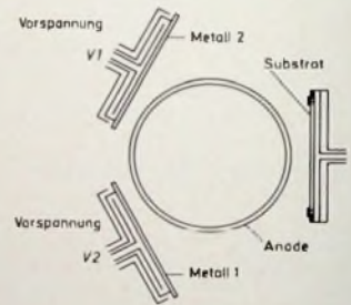
Bild 7 Schema der Katodenzerstäubung nach dem Triodenverfahren
