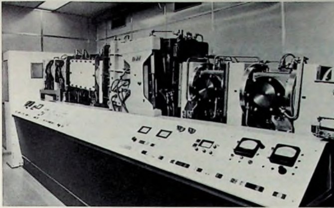
Bild 9 Industrielle Anlage für Katodenzerstäubung mit mehreren Zerstäubungskammern (CIT Alcatel)
