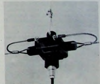
Bild 3 Ringkern-Breitband-Balun von Fritzel
