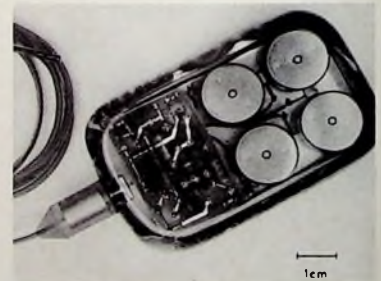
Bild 5 Implantierbarer Herzschrittmacher mit Katheterelektrode (Elema-Schönder-Siemens)
