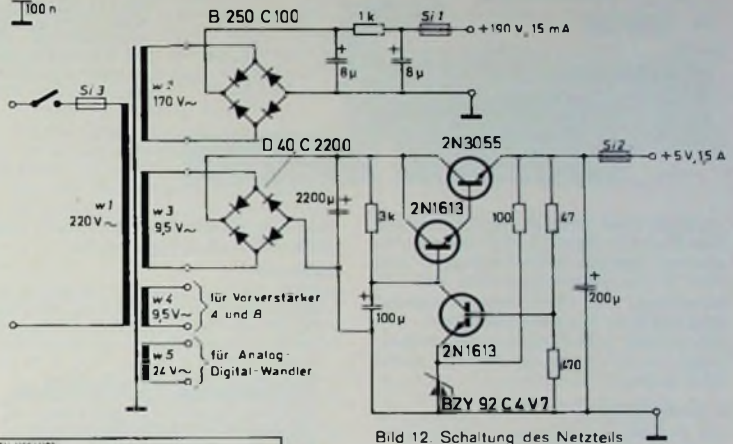
Bild 12. Schaltung des Netzteils
