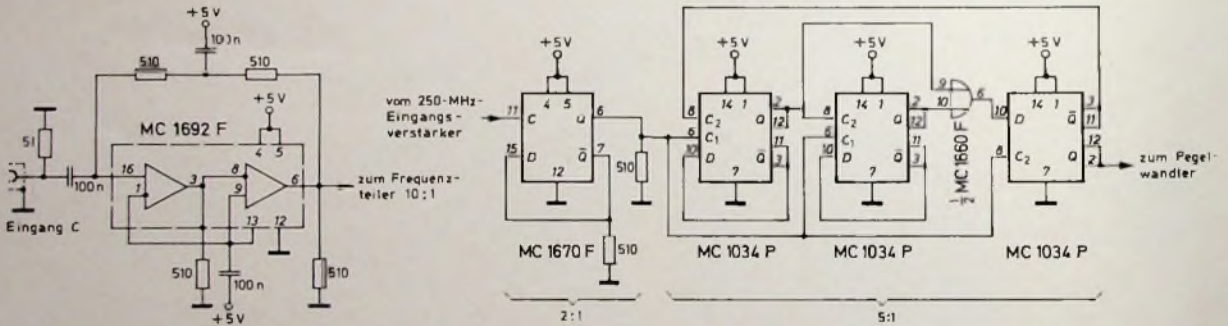
Bild 8. Schaltung des Eingangsverstärkers C
