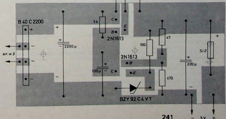
Bild 14 (unten) Gedruckte Schaltung mit Bestückungsplan für die stabilisierte Spannungsversorgung (Maßstab 1:1)
