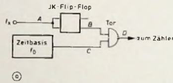
Bild 2 Prinzipschaltung der Zeitbasismessung
