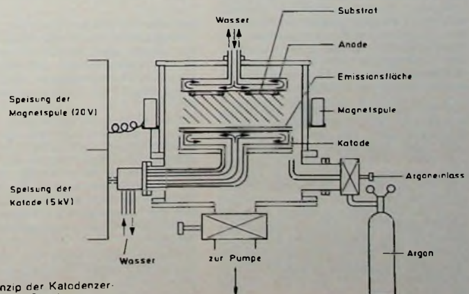
Bild 3. Prinzip der Katodenzerstäubung unter Gleichspannung
