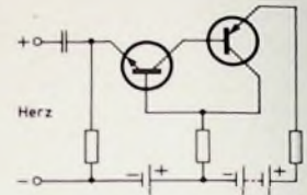
Bild 4 Schaltung eines Herzschrittmachers nach Kantrowitz (1964)
