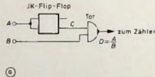
Bild 3 Prinzipschaltung der Verhältnismessung
