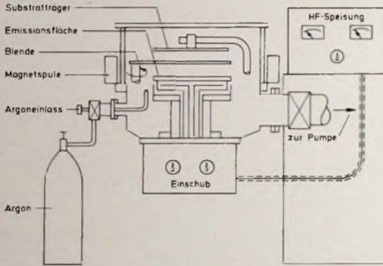
Bild 4 Prinzip der Katodenzerstäubung unter Wechsellspannung
