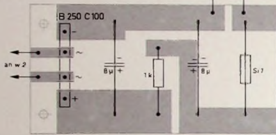
Bild 15. Gedruckte Schaltung mit Bestückungsplan für die 190-V-Spannungsversorgung (Maßstab 1:1)
