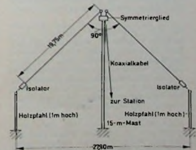
Bild 4 Inverted-V-Antenne für das 80-m-Band mit 90° Scheitelwinkel
