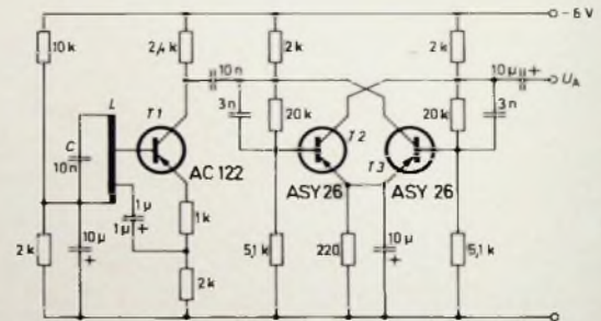
Bild 42. Rechteckgenerator hoher Frequenzkonstanz (untere Anzapfung 1/10 , obere Anzapfung 1/4 der Gesamtwindungszahl von L ; Kern: Siferrit-Schalenkern 18 \times 14 A 1 -400; AEG-Telefunken)
