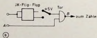
Bild 4 Prinzipschaltung für fortlaufendes Zählen
