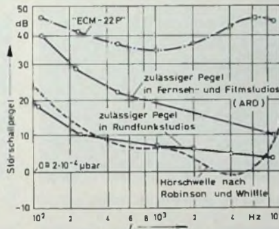
Bild 5 (unten). Zulässiger Störpegel in Rundfunk- und Fernsehstudios
