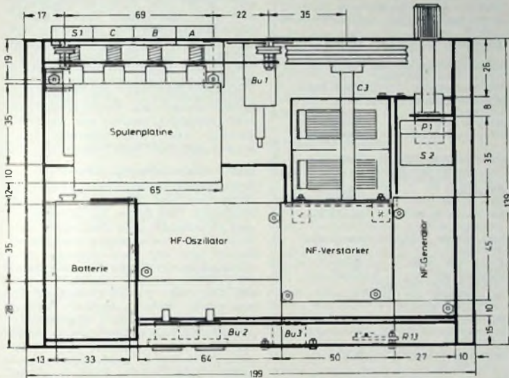
Bild 17 Aufbau der Bausteine auf der Bodenplatte
