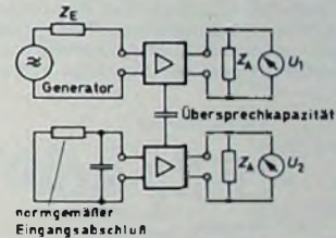
Bild 10 Anordnung zur Messung der Übersprechdämpfung
