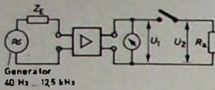
Bild 12 Meßanordnung Ermittlung des Dämpfungsfaktors
