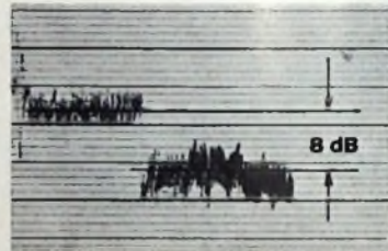
Bild 10. Wirkungswise des aufgesteckten Windschutzes
