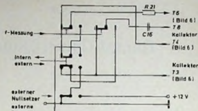
Bild 10. Erweiterung des Multimeters für Zeitmessungen
