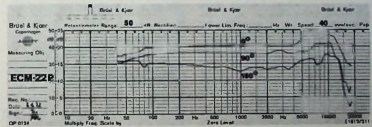
Bild 6 Frequenzgang des Übertragungsmaßes des „ECM-22P“ für die drei Schalleinfallrichtungen
