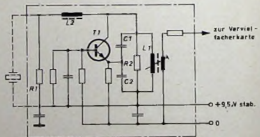
Bild 5. Schaltung des Empfänger-Quarzoszillators der Feststation
