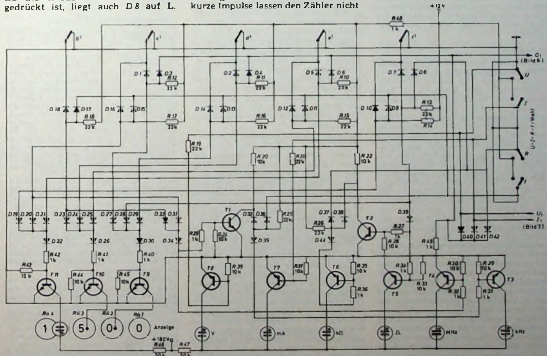
Bild 8. Bereichswahldecoder und Anzeige (D 1... D 44 sind Typ 1N4148, T 1... T 9 sind Typ BCY 59)
