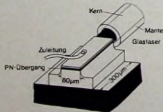
GaAs-Laserdiode mit angekoppelter Glasfaser
