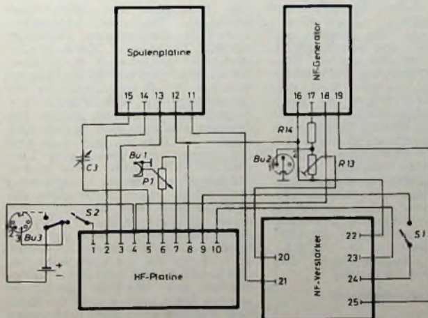
Bild 19 Verdrahtungsplan
