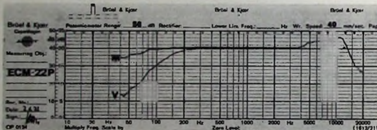
Bild 9. Wirkungswise von S1a, S1b (im Bild 4) für die Stellungen Musik (M) und Geräusch (V)
