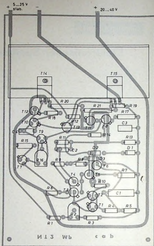
Bild 4 Bestückungsplan der Printkarte
