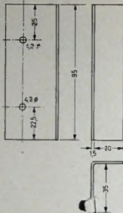
Bild 3 Maßskizze des Kühlkörpers (Aluminium, halbhart)
