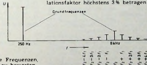
Bild 9 Die als Mischprodukt infolge Intermodulation entstehenden neuen Frequenzen
