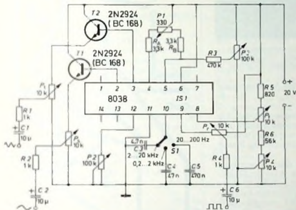
Bild 16. Kompletter Funktionsgenerator (20 Hz ... 20 kHz) mit Frequenzstellung durch veränderbare Gleichspannung
