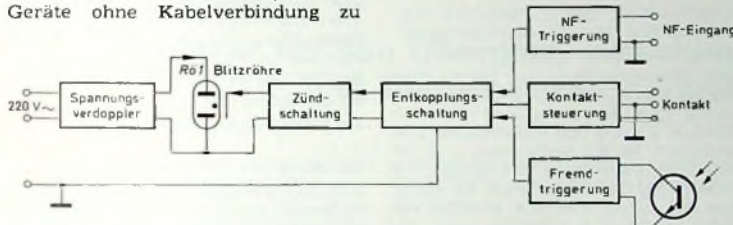
Bild 1. Prinzipschaltung des Lichtblitz-Stroboskops
