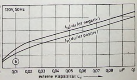
Bild 12 Verwendung einer externen Kapazität zwischen den Anschlüssen 5 und 7 zur zeitlichen Verzögerung der Ausgangsimpulse eines Nullspannungsschalters gegenüber dem Nulldurchgang der Netzspannung
