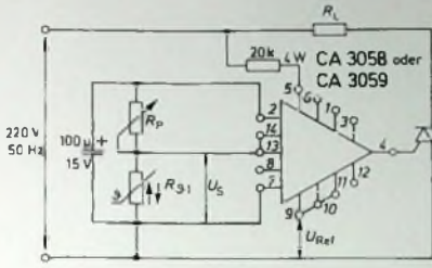
Bild 14 Einfacher Zweipunkt-Temperaturregler mit dem Nullspannungsschalter CA3058 oder CA3059
