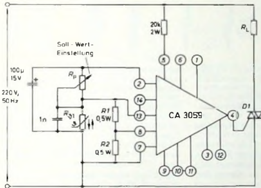
Bild 6. Zweipunkt-Temperaturregler mit Hysterese
