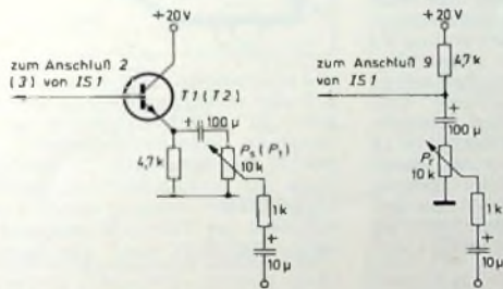
Bild 17 (oben). Gleichstromfreie Anschaltung der Ausgangspotentiometer
