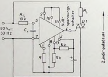
Bild 12 Verwendung einer externen Kapazität zwischen den Anschlüssen 5 und 7 zur zeitlichen Verzögerung der Ausgangsimpulse eines Nullspannungsschalters gegenüber dem Nulldurchgang der Netzspannung
