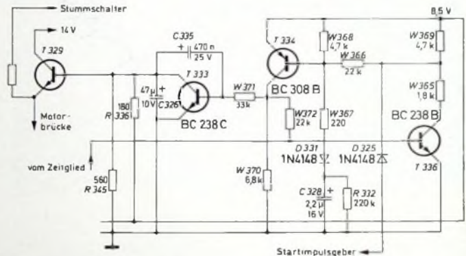
Bild 4. Geschaltete Stromversorgung
