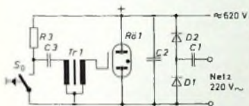
Bild 2. Spannungsversorgung und Zündschaltung der Blitzröhre
