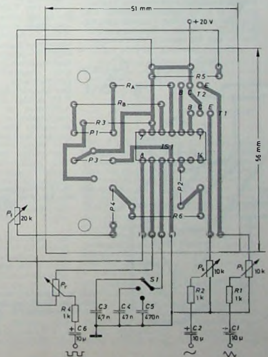
Bild 19. Bestückungsplan für die Schaltung nach Bild 16
