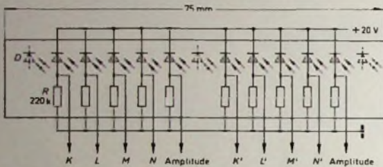
Bild 34 Mit einer Amplituden- und vier Tonspuren je Spielstimme können jeweils 16 Tonfrequenzen gesteuert werden
