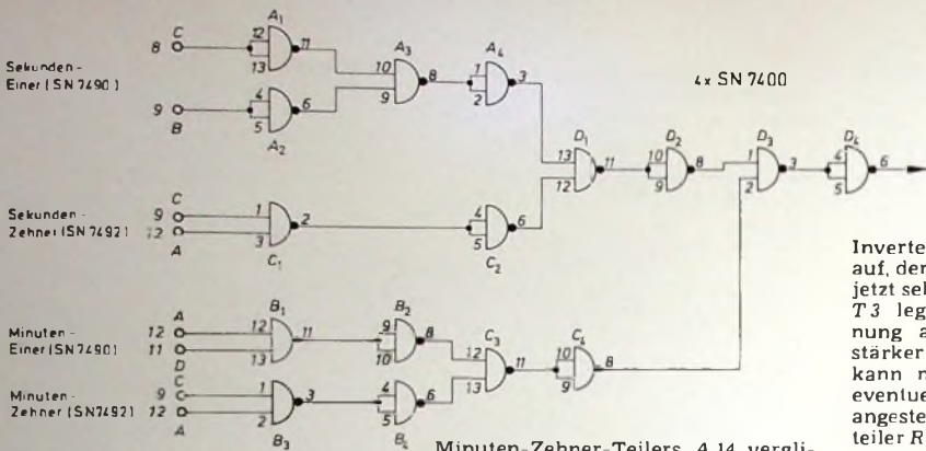
Bild 3 Logikschaltung zur Erzeugung der Zeitzeichensignale
