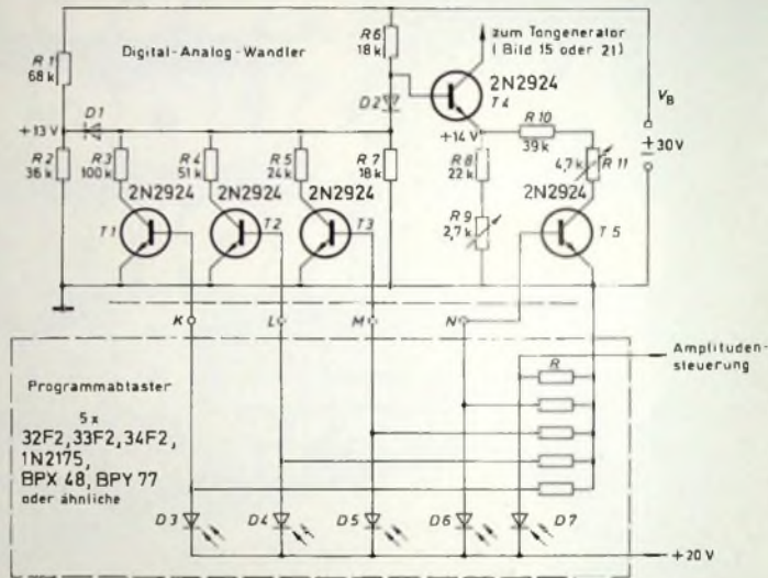
Bild 35 Die Binärwerte werden in eine Analoggröße umgewandelt, die der logarithmischen Tonleiterfunktion angenähert wird
