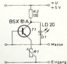
Bild 3 Schaltung eines LED-Voltmeters vom zweiten Anzeigertyp
