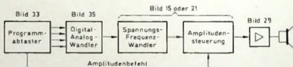
Bild 32 Umwandlung des binären Digitalprogramms in eine elektrische Analoggröße, die den Tonoszillator steuert
