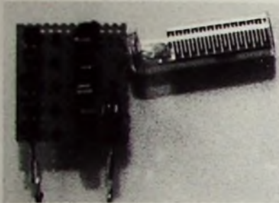
Bild 6. LED-Helligkeitsmeßgerät
