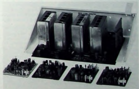
Bild 3. SECAM-PAL-Transcoder „22 ET 6550/00“
