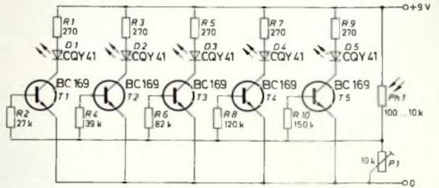
Bild 6. LED-Helligkeitsmeßgerät
