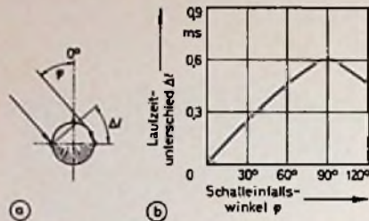
Bild 4 (oben). Entstehung von Laufzeitunterschieden \Delta t bei schief einfallenden ebenen Schallwellenfronten; a) Laufzeitunterschied als Folge unterschiedlicher Weglängen \Delta l zu den Ohren, b) Laufzeitunterschied \Delta t in Abhängigkeit vom Schalleinfallswinkel \varphi
