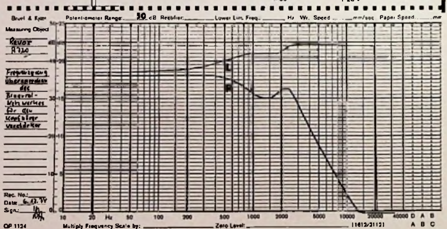
Bild 7. Frequenzgang der Ausgangsspannung und des Übersprechens an den Kopfhöreranschlüssen L und R bei frequenzabhängiger Eingangsspannung am Aux.-Eingang des Kanals L ( R_L = 18 \text{ k}\Omega )
