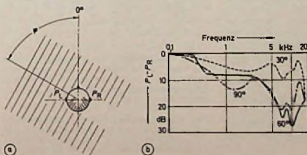
Bild 3. Entstehung von Intensitätsunterschieden bei seitlichem Schalleinfall für beidohriges Hören; a) Abschattung durch den Kopf, b) Frequenzgang der Schallbeugung um den Kopf in Abhängigkeit vom Schalleinfallswinkel
