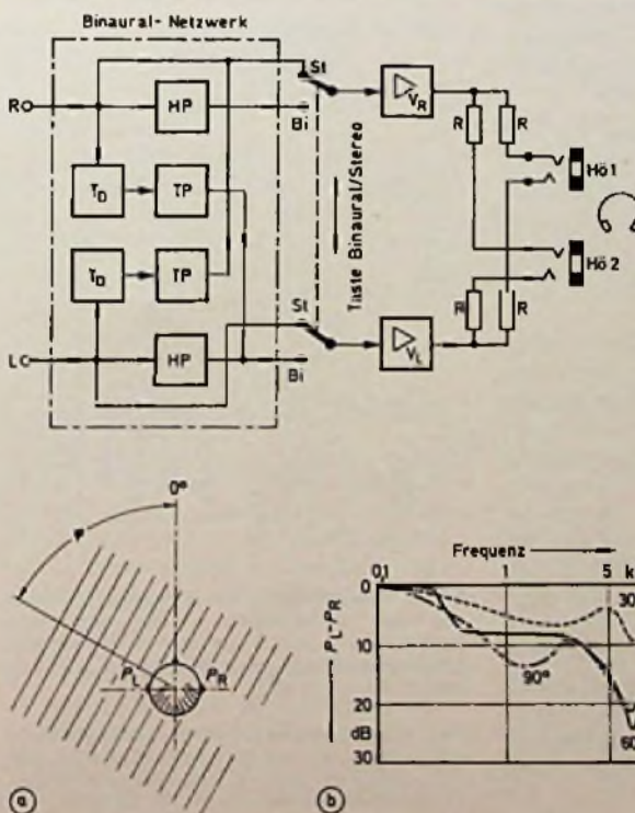
Bild 2. Blockschaltbild des Stereo-Kopfhörerverstärkers mit vorgeschaltetem Stereo-Binauralconverter (HÖ 1, HÖ 2 Kopfhöreranschlüsse, HP Hochpaß, TP Tiefpaß, TD Zeitverzögerung, V L , V R Verstärker für linken beziehungsweise rechten Kanal)
