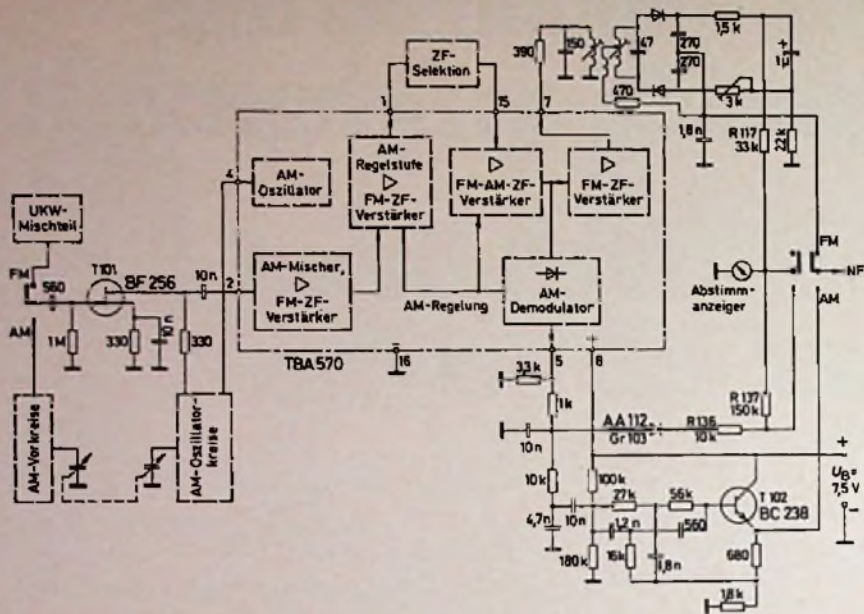
Bild 2. Vereinfachtes Schaltbild des HF-ZF-Verstärkers (gezeichnete Schalterstellung: UKW)
