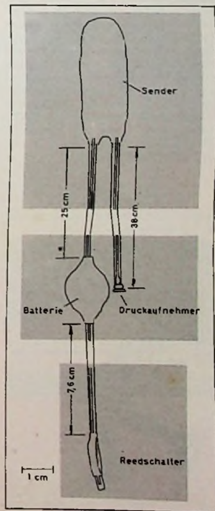
Bild 5. Implantierbare Sendeeinrichtung für Blutdruckmessung im Gefäßsystem.
