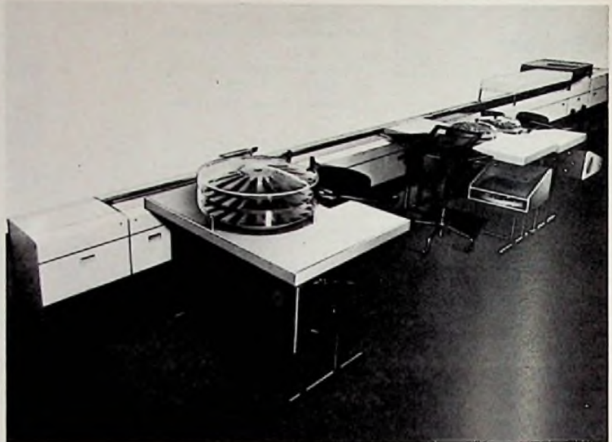
Bestückungs- und Lötanlage „Modul-Line“ für Leiterplatten.
