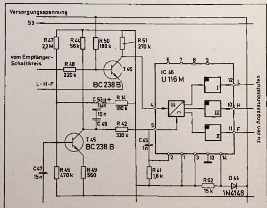
Baugruppen des Ultraschall-Empfängers: Selektion (oben) und D/A-Wandler (unten).
