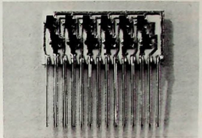
Oben: Je zwölf Widerstände und Transistoren enthält diese Dickfilmschaltung von AEG-Telefunken, bei der Leiterbahnen und passive Komponenten auf ein Keramikplättchen aufgedruckt sind, während Halbleiter-Bauteile als Chips aufmontiert wurden.
