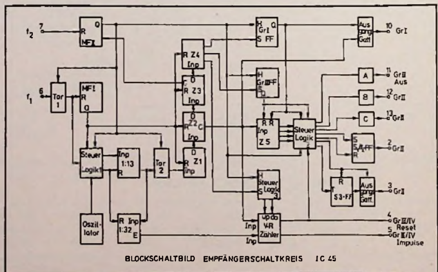
Blockschaltbild des Empfänger-Schaltkreises IC 45.
