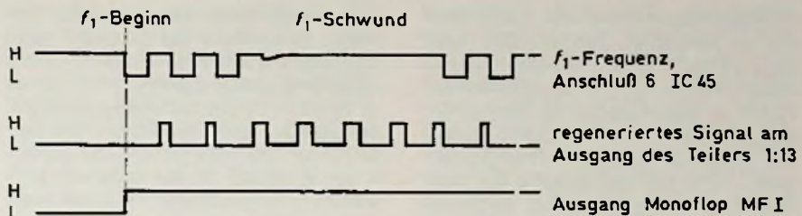
Schwundunterdrückung der f_1 -Frequenz
