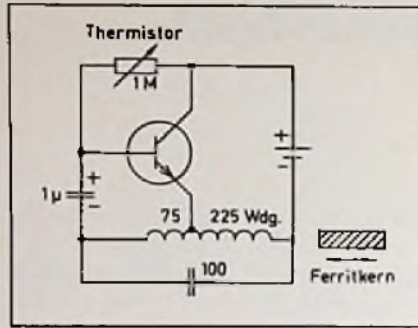
Bild 2. Sperrschwinger zur gleichzeitigen Übermittlung zweier biologischer Kennwerte [6].
