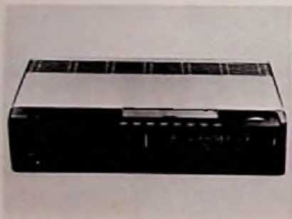
Marke: Teleton Modellname: TFS 80 Erstlieferung a. d. Handel: Jan. 76 Endverkaufspreis: liegt bei 1000 DM Bereiche: UKW, KW, MW, LW Nennleistung an 8 Ohm: 2 x 33 W Quadro: quasi
