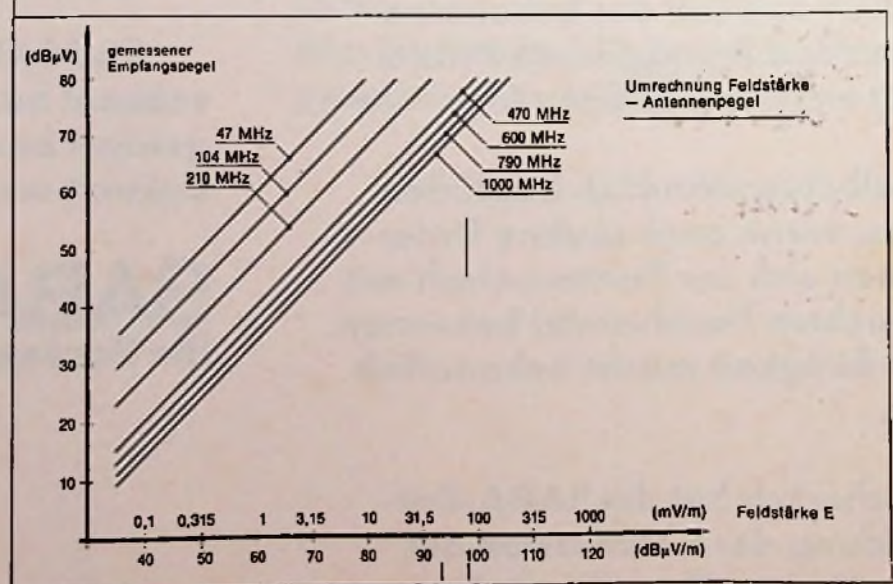
Zusammenhang zwischen Feldstärke und Spannungspegel mit der Frequenz als Parameter. (Diagramm: Philips)
