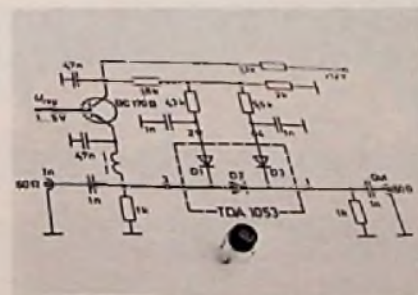
PIN-Dioden-Regler TDA 1053 (Intermetall).
