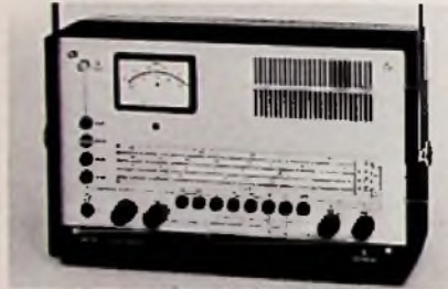
Marke: Siemens Modell: S 43101-M-B Bereich: Hör-Rundfunk Pegelbereich: 14–128 dB \mu V (LMK); 6–123 dB \mu V (UKW) Meßunsicherheit: \pm 3 dB Anzeige: Zeiger Tonwiedergabe: Lautsprecher Stromversorgung: Batterie, Akku Gewicht: 9,5 kg Preisbeobachtung: 2200 DM
