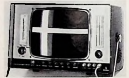
Marke: Siemens Modell: S 43201-M-D Bereich: Fernsehen Pegelbereich: 30–130 dB \mu V Meßunsicherheit: \pm 2 dB Anzeige: Bild, Zeiger Tonwiedergabe: Lautsprecher Stromversorgung: Netz, Batterie/Akku Gewicht: 14,5 kg Preisbeobachtung: etwa 3300 DM
