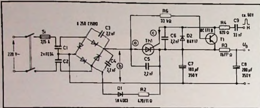
Bild 4. Netzteil mit elektronischer Sicherung mit Einschaltstrombegrenzung
