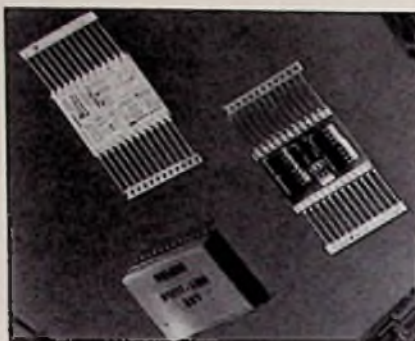
Dieses aktive RC-Filter hat Siemens in Tantal-Dünnschichttechnik mit hybridisierten Kondensatoren und Operationsverstärkern für den Frequenzbereich von 20 Hz bis 20 kHz ausgelegt.
