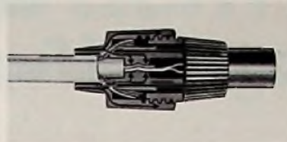
DIN-Stecker für Koaxialkabel mit einer neuartigen Klemmung ohne Madenschraube (Kathrein).
