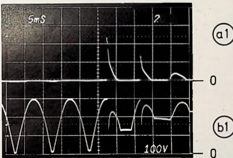
Bild 2. Oszillogramme zu der im Bild 1 gezeigten elektronischen Sicherung während der Einschaltphase des Thyristors Th1. Die Zündung erfolgte im Maximum einer Sinushalbwellen der gleichgerichteten Spannung.
