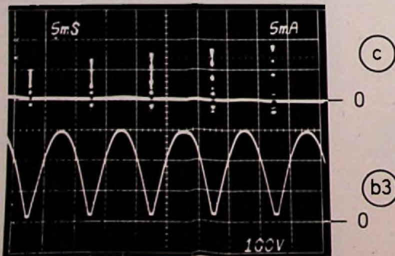
Bild 5. Verlauf des Gate-Stromes c und der Anodenspannung b3 am Thyristor Th1 während der Einschaltphase des Fernsehempfängers, kurz bevor der Thyristor Th1 gezündet wird
