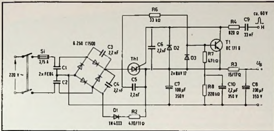
Bild 6. Netzteil mit elektronischer Sicherung; Einschaltstrombegrenzung und Stromstoßbegrenzung bei Kurzzeitunterbrechung
