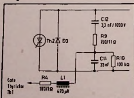
Bild 7. Ansteuerschaltung für den Thyristor Th1 der elektronischen Sicherung bei Fernsehempfängern mit Netztrennung
