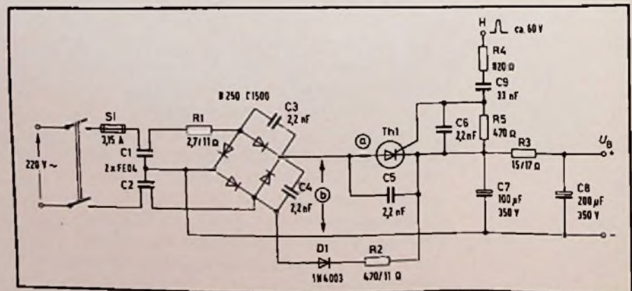
Bild 1. Netzteil mit elektronischer Sicherung in herkömmlicher Schaltungstechnik
