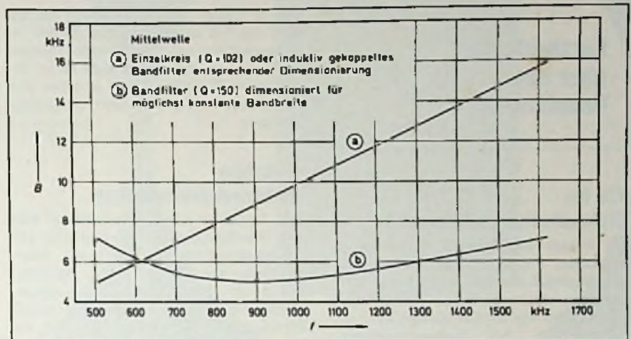
Bild 5. Die Bandbreite eines Einzel-Schwingkreises oder eines induktiv gekoppelten Filters (a) im Vergleich zu einem Zweikreis-Filter (b) mit möglichst konstanter Bandbreite; berechnet für den Mittelwellenbereich
