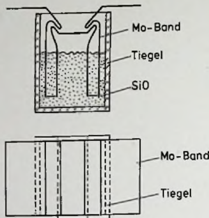
Bild 5. Verdampfer für SiO 2
