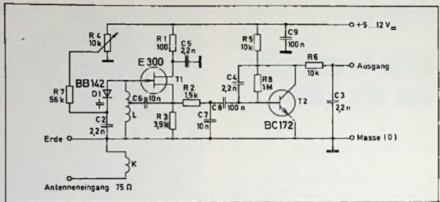
Bild 1. Schaltung des Pendelrückkopplungs-Empfängers für Kopfhörerwiedergabe oder nachgeschaltetem NF-Verstärker
