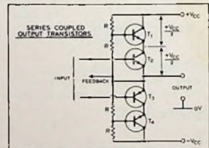
Das von Motorola entwickelte Konzept des reihengekoppelten Ausgangs
