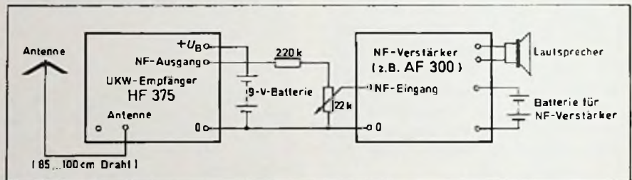
Bild 2. Ankopplung eines NF-Verstärkers AF 300; es lassen sich jedoch auch andere Verstärker verwenden
