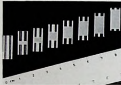
Bild 13. Dämpfungsglieder (0...70 dB) in Dünnschichttechnik für HF-Anwendung
