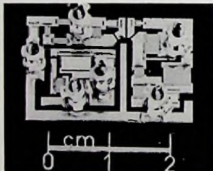
Bild 14. 60-MHz-Gegenkopplungsnetzwerk in NiCr/SiO-Technologie
