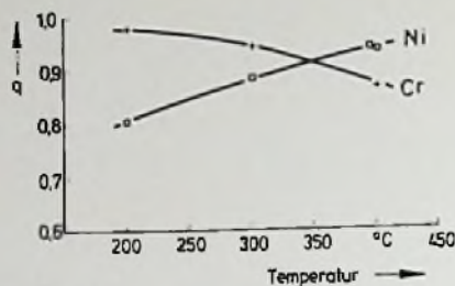
Bild 2. Kondensationskoeffizient von Nickel und Chrom
