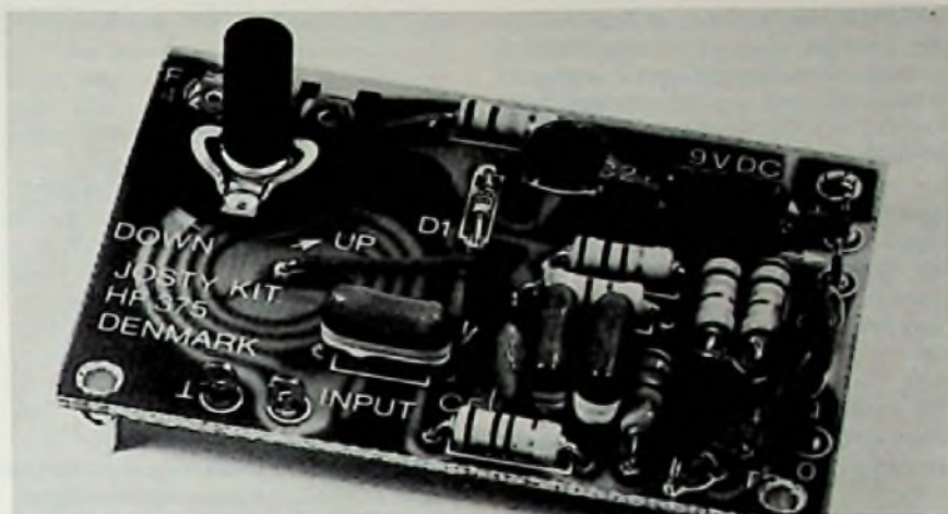
Der betriebsfertige UKW-Empfänger
