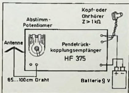
Bild 4. Anschluß von Antennen, Batterie und Kopfhörer an den UKW-Empfänger
