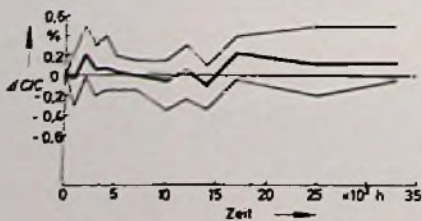
Bild 9. Dauerversuch von Al-SiO 2 -Al-Kondensatoren (90 % relative Feuchte, R. T.)
