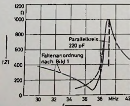
Bild 2. Frequenzgang der Impedanz |Z|, die der Selektion der Fallenanordnung entspricht
