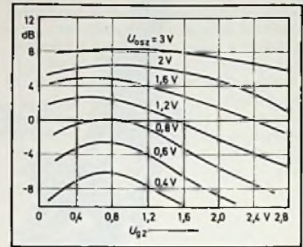
Bild 3. Mischverstärkung in Abhängigkeit von der Gate-2-Spannung
