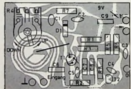
Bild 3. Das fertig bestückte Gerät; die Leiterbahnen befinden sich auf der anderen Seite der Platine
