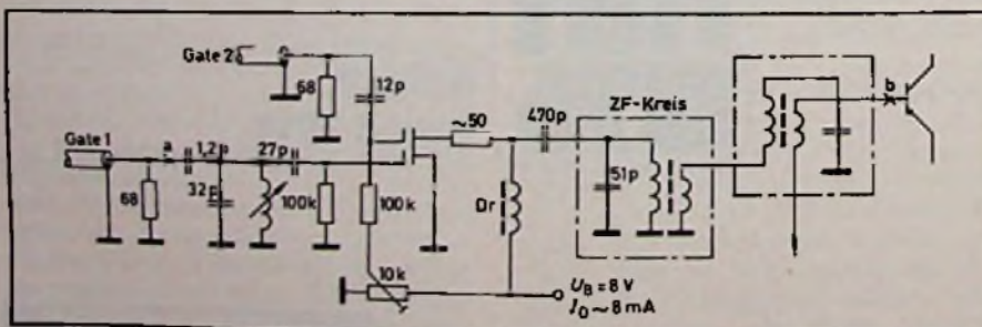
Bild 1. Multiplikative Mischschaltung mit Dual-Gate-MOS-FET BF-900
