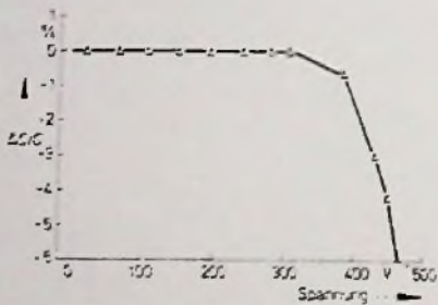
Bild 8. Relative Kapazitätsänderung \Delta C/C von Al-SiO 2 -Al-Kondensatoren im Überspannungsversuch (SiO 2 hat 1 \mu\text{m} )
