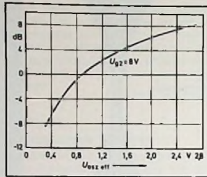
Bild 2. Mischverstärkung in Abhängigkeit von der Oszillatoramplitude
