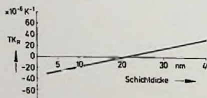
Bild 4. TK_R von NiCr-Widerstandsschichten
