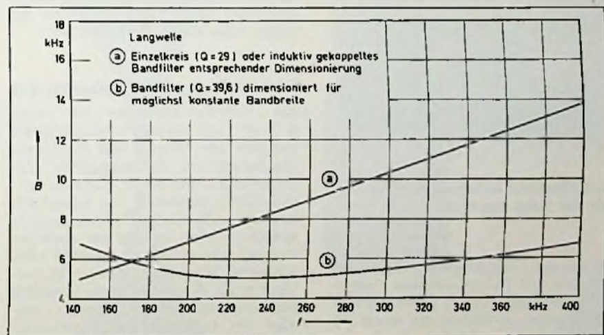
Bild 6. Die Bandbreite eines Einzel-Schwingkreises oder eines induktiv gekoppelten Filters (a) im Vergleich zu einem Zweikreis-Filter (b) mit möglichst konstanter Bandbreite; berechnet für den Langwellenbereich
