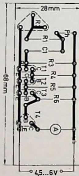
Bild 2. Schalt- und Bestückungsplan des Mustergerätes
