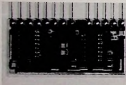
Eine Dickschichtschaltung mit Miniatur-ICs von Valvo-Signetics
