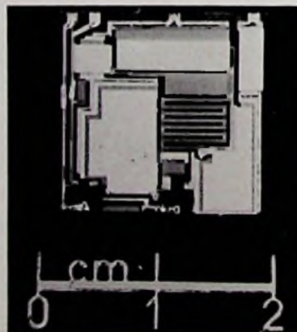
Bild 15. RC-Nullfilterverstärker (2,14 MHz)
