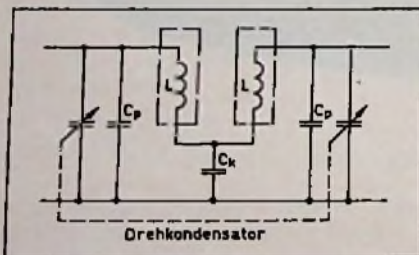
Bild 4. Praktische Ausführung eines abstimmbaren zweikreisigen Bandfilters mit kapazitiver Querkopplung über C_k
