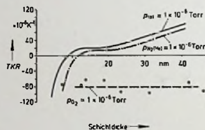
Bild 3. Aufgedampfte CrNi-Schichten (UHV)
