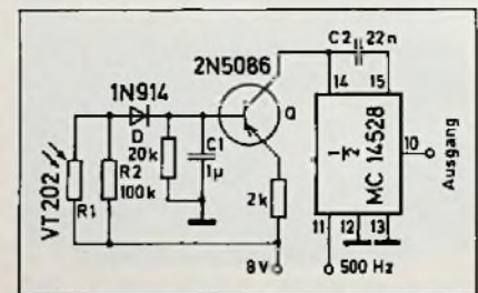
Die Schaltung des automatischen Dämmerungsreglers für Leuchtanzeigen
