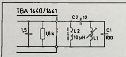
Bild 1. Die von Siemens empfohlene Schaltung des Trägerkreises; L1: 5 Wdg. 0,3 CuL auf Spulenkörper Vogt D 4100 mit Becher, ohne Glockenkern
