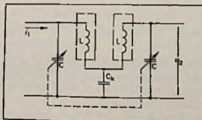
Bild 1. Prinzipschaltung eines abstimmbaren zweikreisigen Bandfilters mit kapazitiver Querkopplung über C_k
