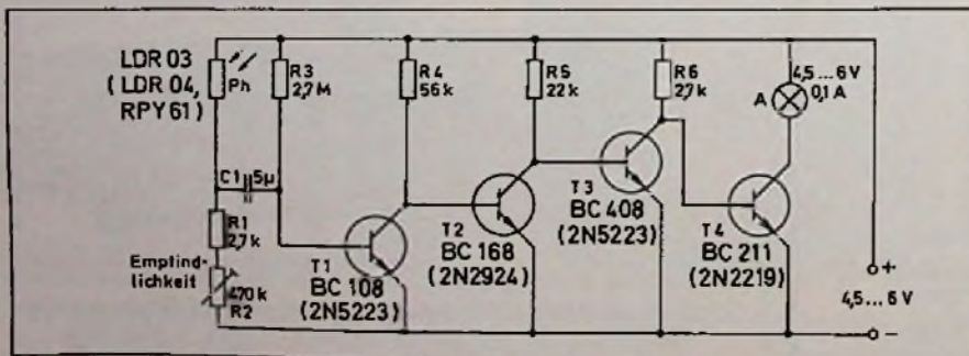
Bild 1. Die Schaltung verarbeitet nur rasche Beleuchtungsänderungen, an langsame paßt sie sich an
