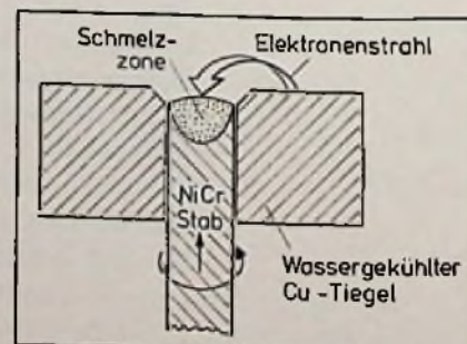
Bild 1. Prinzip der Verdampfung vom Stab mit E-Kanone
