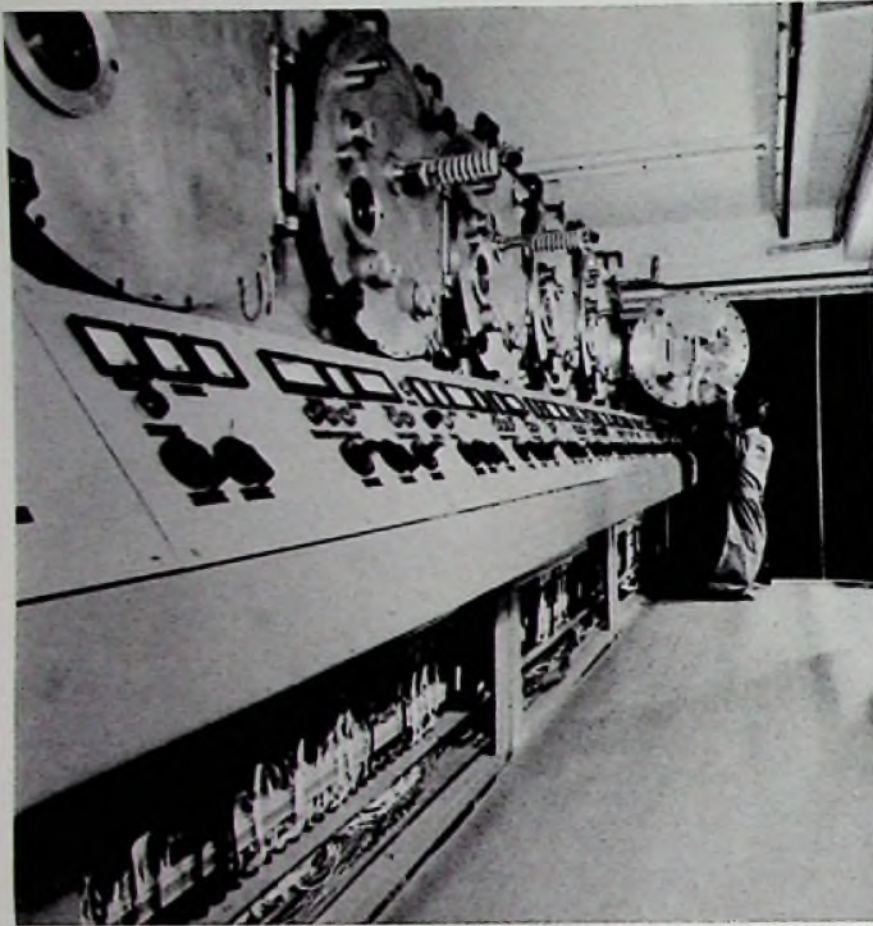
Bild 11. Lineare Aufdampfanlage für Schichtschaltkreise
