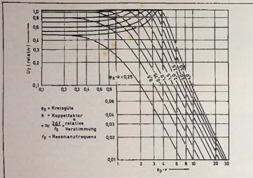
Bild 2. Abhängigkeit der Spannung u_2 am Sekundärkreis eines Zweikreis-Bandfilters von der normierten Verstimmung \rho_0 \cdot \nu ; als Parameter dient die normierte Kopplung \rho_0 \cdot k
