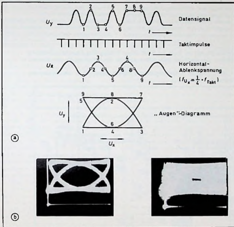
Bild 14. „Augen“-Diagramm zur Beurteilung von Datensignalen; a) zur Entstehung des Augen-Diagramms, b) Augen-Diagramme von Datensignalen mit verschiedenen Störwirkungen
