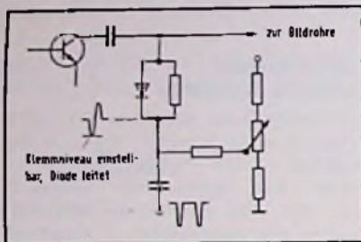
Bild 45. Prinzip einer Klemmschaltung (Grundlg)
