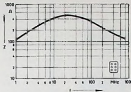
Bild 1.88 Scheinwiderstandsverlauf von Ferrit-Drosselspulen mit 2,5 Windungen bei einer Feldstärke H \leq 10 mA/cm (Siemens)
