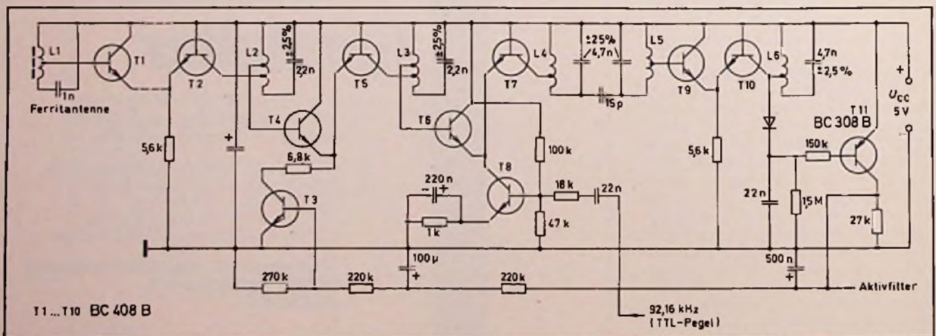
Bild 5. Überlagerungsempfänger
