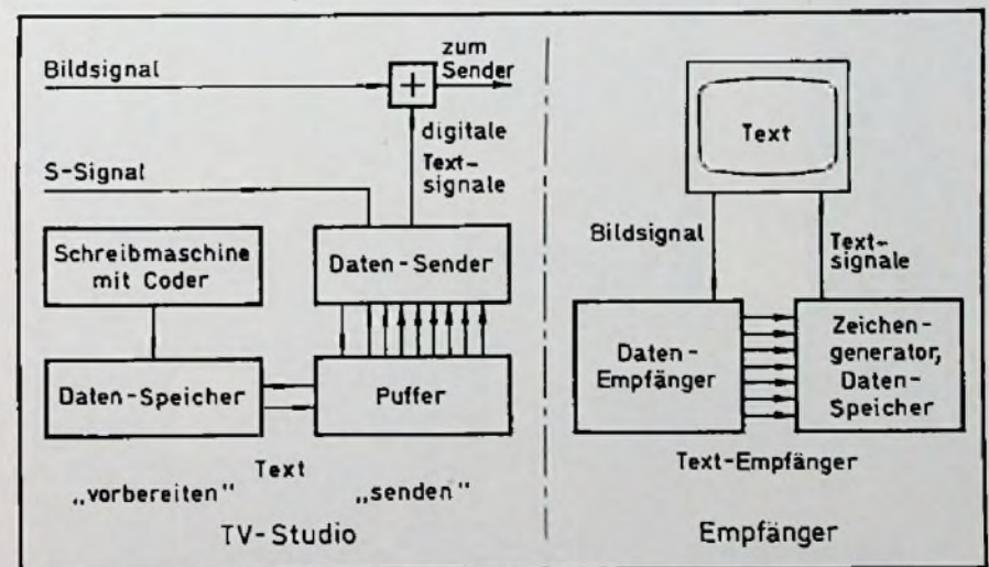
Bild 8. Funktionsschema der digital codierten Übertragung von Zeichen in der V-Auslastlücke des Fernsehsignals
