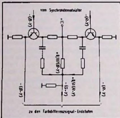
Bild 46. Prinzipschaltung einer Matrix (Grundlg)
