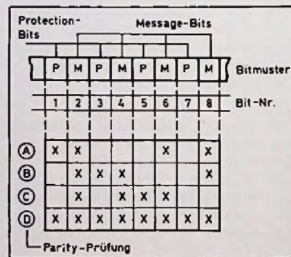
Bild 6. Schema der Hamming-Codierung zur Erkennung und Korrektur von Fehlern in Bitmustern
