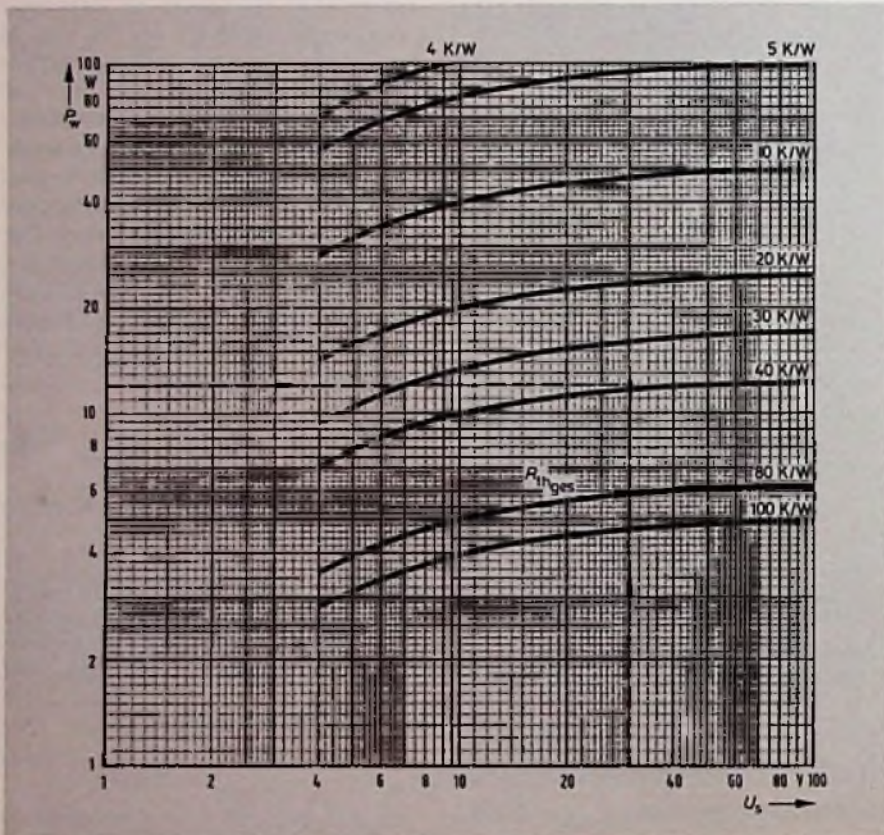
Bild 132. Wechselleistung P_w = f(U_s) . Parameter: Gesamter Wärmewiderstand R_{Th\ ges} eines Transistors
