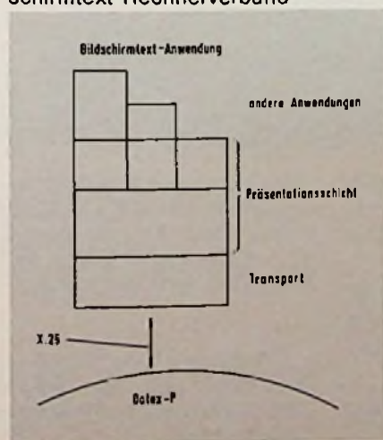
Bild 5. Schichtenstruktur der Kommunikations-Protokolle für Bildschirmtext-Rechnerverbund
