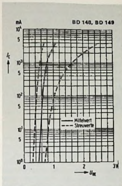
Bild 133. Kollektorstrom I_C = f(U_{BE}) für den Leistungstransistor BD 148 (Siemens)
