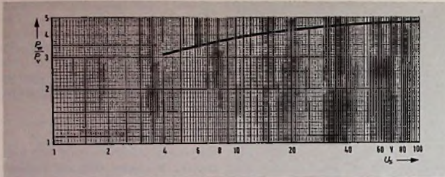
Bild 131. Verhältnis der Wechselleistung des gesamten Verstärkers ( P_w ) zur Verlustleistung eines Endstufentransistors ( P_v ) als Funktion von U_s
