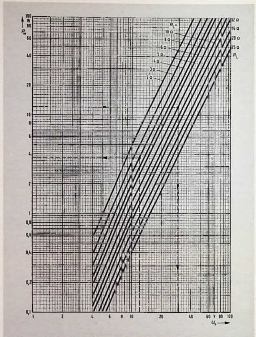
Bild 129. Wechselleistung P_w = f(U_s) . Parameter: R_L = 2 \Omega bis 25 \Omega .
