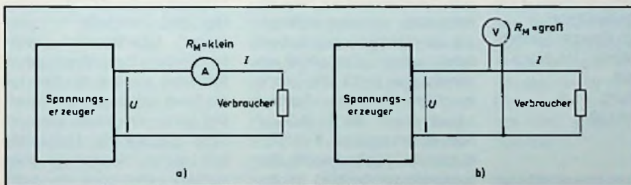
Bild 2. a) Schaltung des Meßinstrumentes beim Strommessen; b) Schaltung des Meßinstrumentes beim Spannungsmessen
