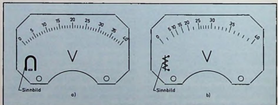
Bild 1. Skalentellung von Spannungsmessern: a) beim Drehspulinstrument; b) beim Dreheiseninstrument
