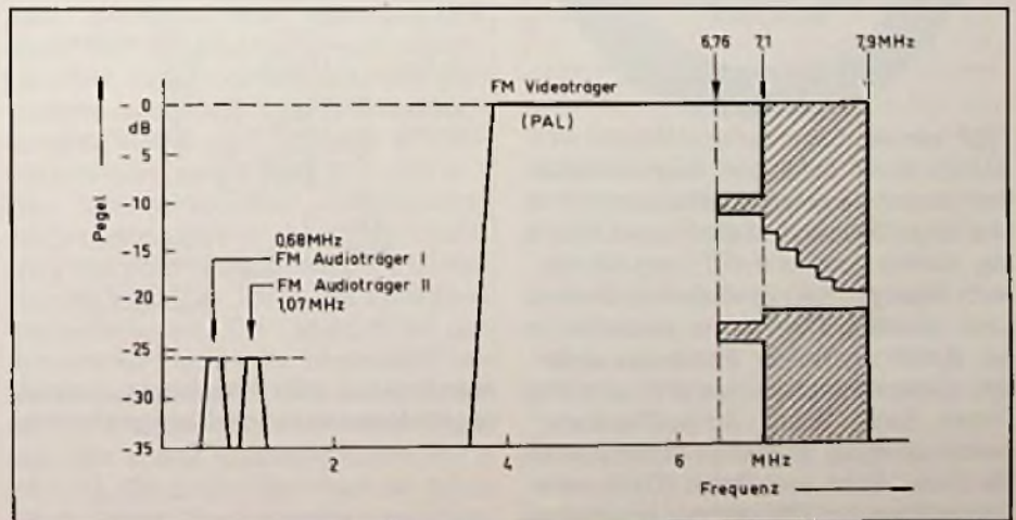
Bild 14. Das VLP-Frequenzspektrum für die PAL-Norm
