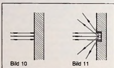
Bild 10. Reflexion an einer ebenen Fläche
