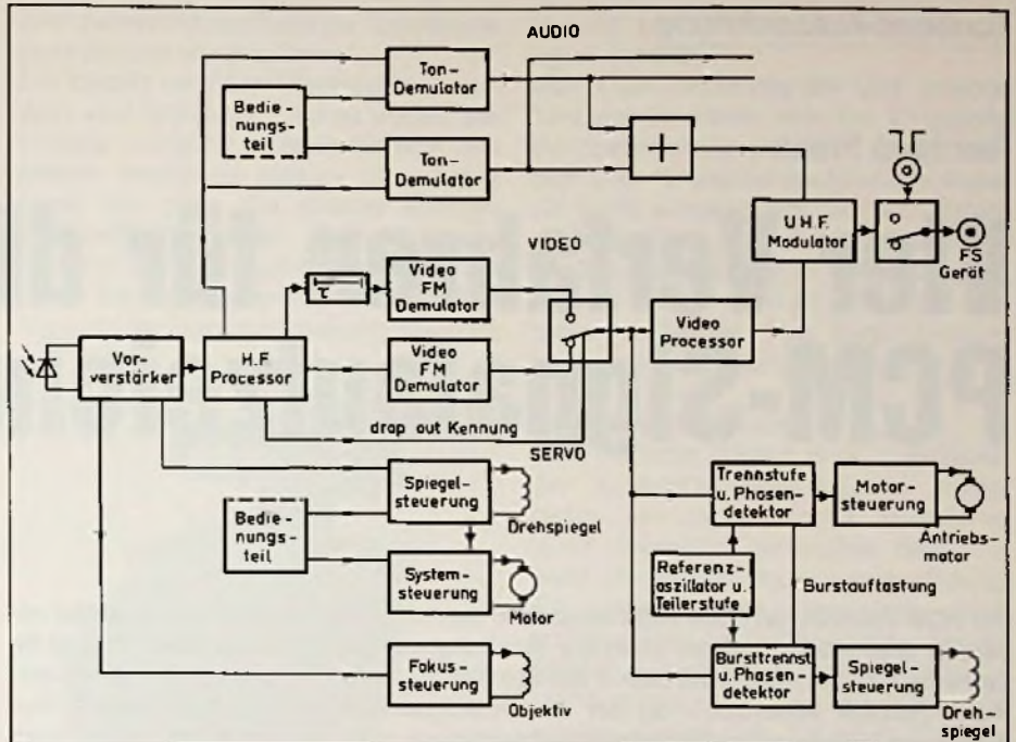
Bild 20. (rechts) Blockscha des Audio-, Video- und Servotells eines VLP-Plattenspielers
