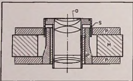
Bild 16. (unten) Prinzip der elektrodynamischen Objektivauflösung: O = Objektiv; P = Polschuhe; M = Magnet; S = Spule
