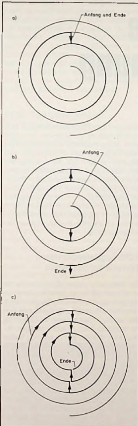
Bild 19. Diese Wege geht der Strahl bei Sonderfunktionen: a) Standbild; b) Zeitraffer; c) Bildrücklauf
