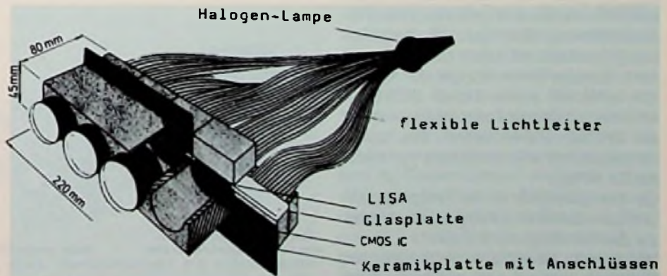
Bild 1: Prinzipielle Anordnung eines Druckkopfes für die Lichtschaltanrichtung (Valvo)
