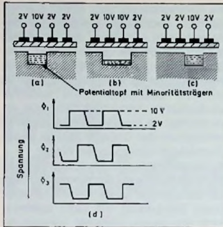
Bild 3: Durch geeignetes Taktten der Zellen wandert der Potentialtopf samt Inhalt von einer Zelle zur anderen
