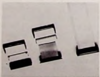
Bild 1: Das „TCL“ Steckverbinder System von Du Pont Berg Electronics ermöglicht kostengünstige Steckverbindungen bei hoher Packungsdichte mit einem definierten Wellenwiderstand, der wahlweise 50, 75 oder 100 V betragen kann.
