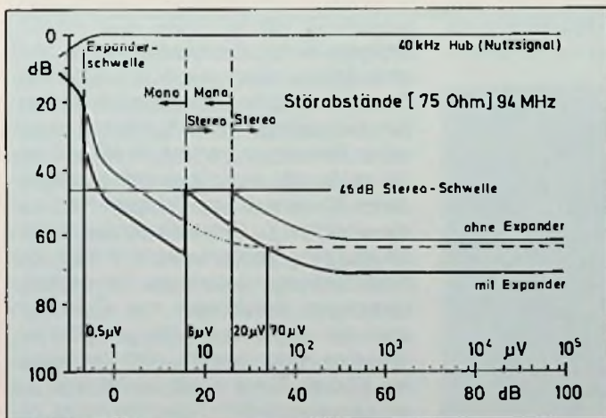
Bild 1: Störabstände mit und ohne Expander
