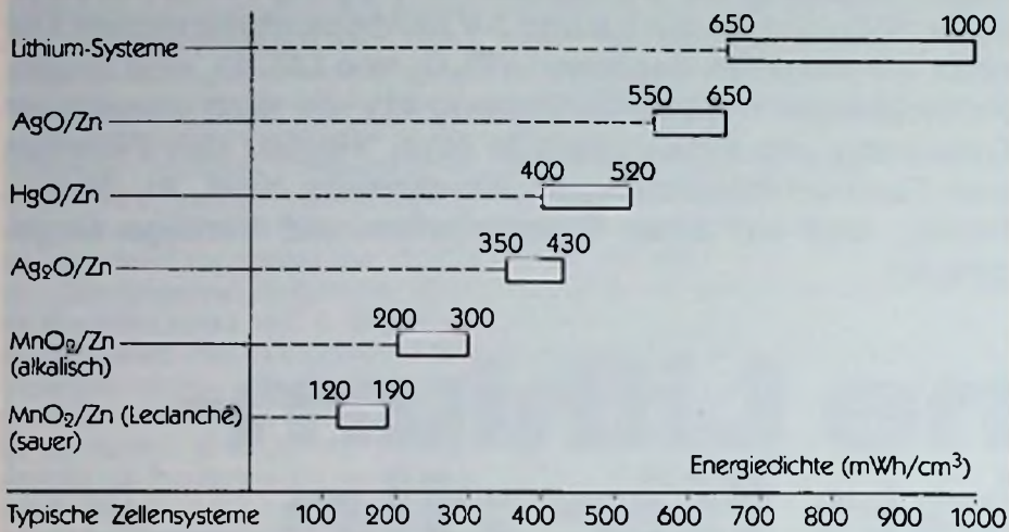
Bild 2: Energiedichten der wichtigsten Batteriesysteme (Primer-Systeme)
