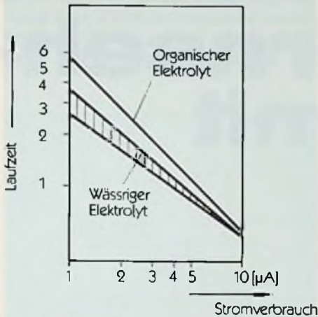
Bild 3: Laufzeiten von Knopfzellen in Quarzanaloguehren
