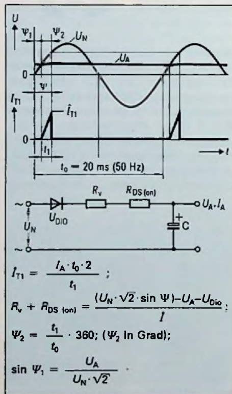
Bild 5: Berechnung der Schaltung nach Bild 3
