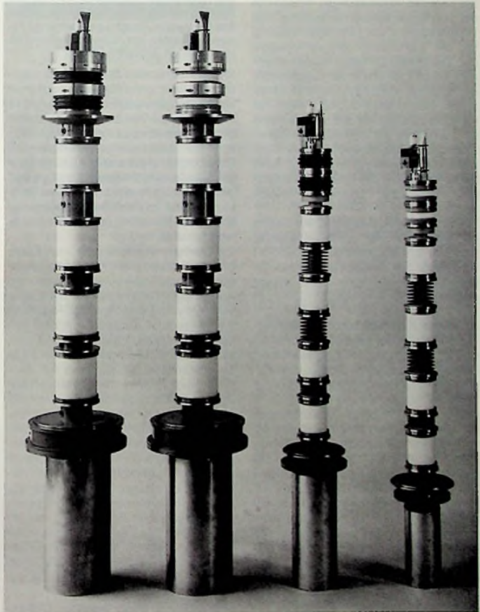
Bild 1: Moderne Klystrons für Fernsehsender mit 20 kW und 60 kW Ausgangsleistung (Valvo-Pressbild)
