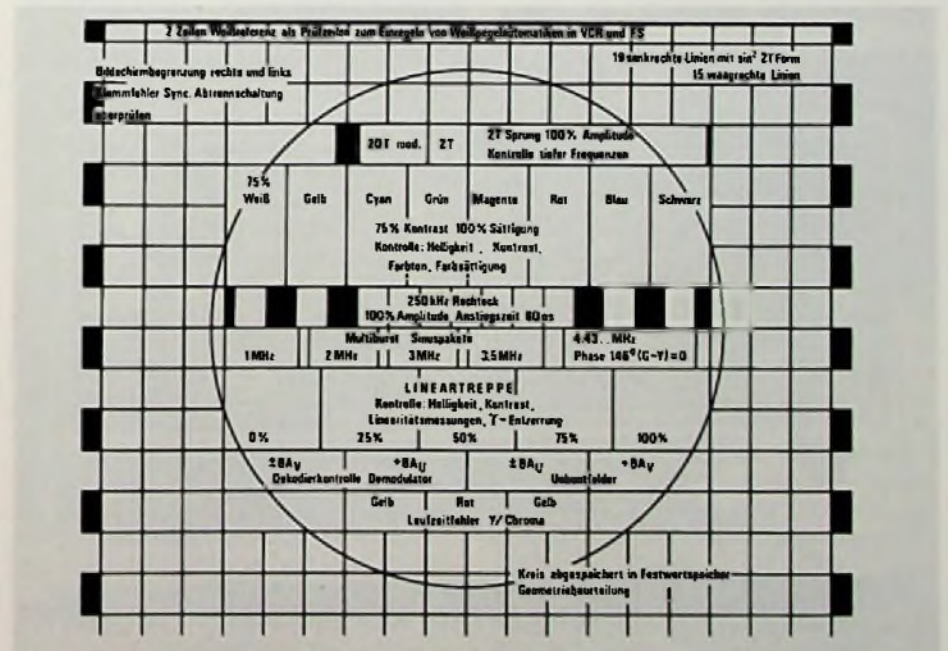
Bild 1: Universal-Testbild zur visuellen und/oder meßtechnischen Überprüfung von Video-Geräten
