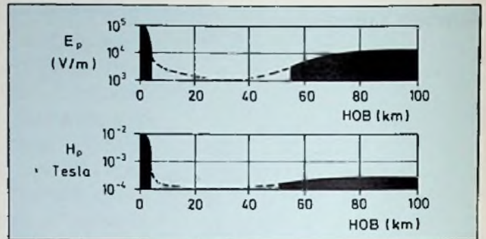
Bild 3: Abhängigkeit der elektrischen Feldstärke und der entstehenden Magnetfeldichte von der Explosionshöhe über dem Erdboden (HOB)
