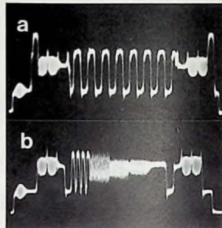
Bild 4: Verwendung des vom Sender ausgestrahlten FuBK-Testbildes zur visuellen Überprüfung; a) des Einschwingverhaltens mit dem 250 kHz-Sprungimpuls; b) des Übertragungsbereiches eines Videorecorders
